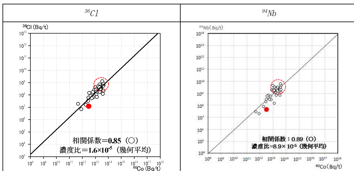
図 13(2)-1(1) (図 I. 8-ZrTN804D (BWR チャンネルボックスの本体) の難測定核種及び Key 核種 ( ^{60}\text{Co} ) の散布図 (放射化計算結果) から抜粋)
