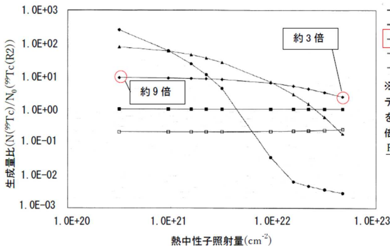
図 4.3.1-52 ^{98}\text{Mo}(n, \gamma)^{99}\text{Mo}(\beta^-)^{99}\text{Tc} のスペクトル感度 (熱外中性子)
