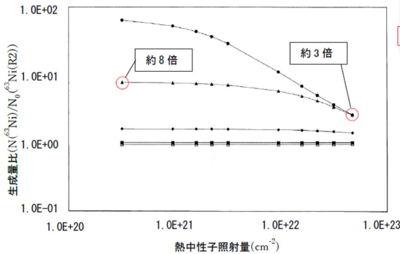
図 4.3.1-39 ^{62}\text{Ni}(n, \gamma)^{63}\text{Ni} のスペクトル感度 (熱外中性子)
