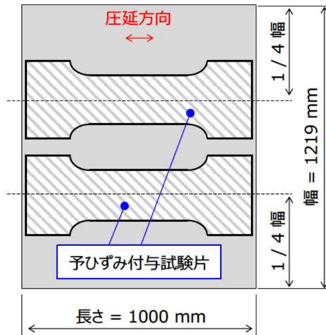
(a) 予ひずみ付与試験片の採取
