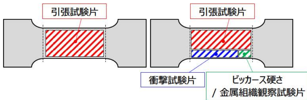
(c) 各種材料試験片の採取
