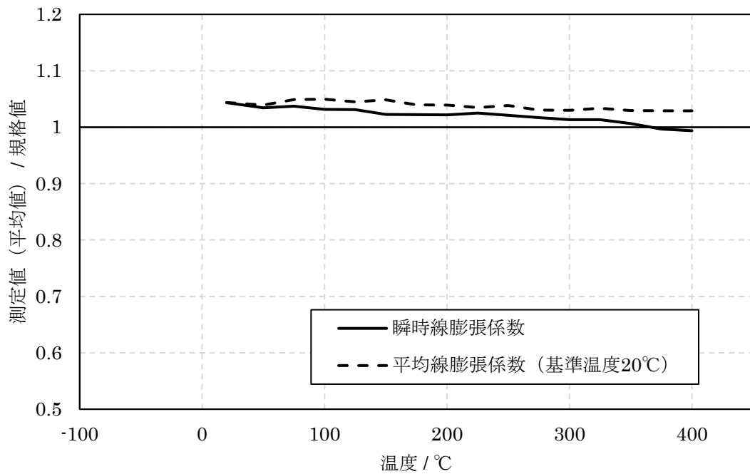
図 別 1-10 線膨張係数 (瞬時及び室温からの平均) の比較 : SG295 と 材料規格分類 [TE1] (炭素鋼、合金鋼[区分 I])
