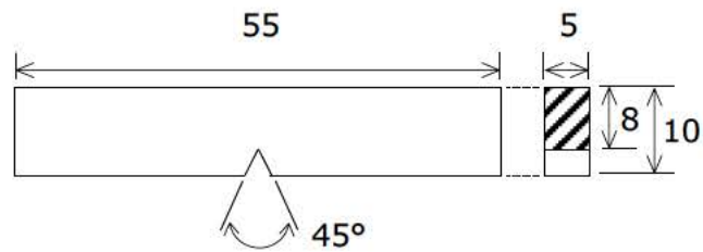
図 別 5-5 シャルピー衝撃試験形状 (JIS Z 2242 5 mm サブサイズ試験片)
