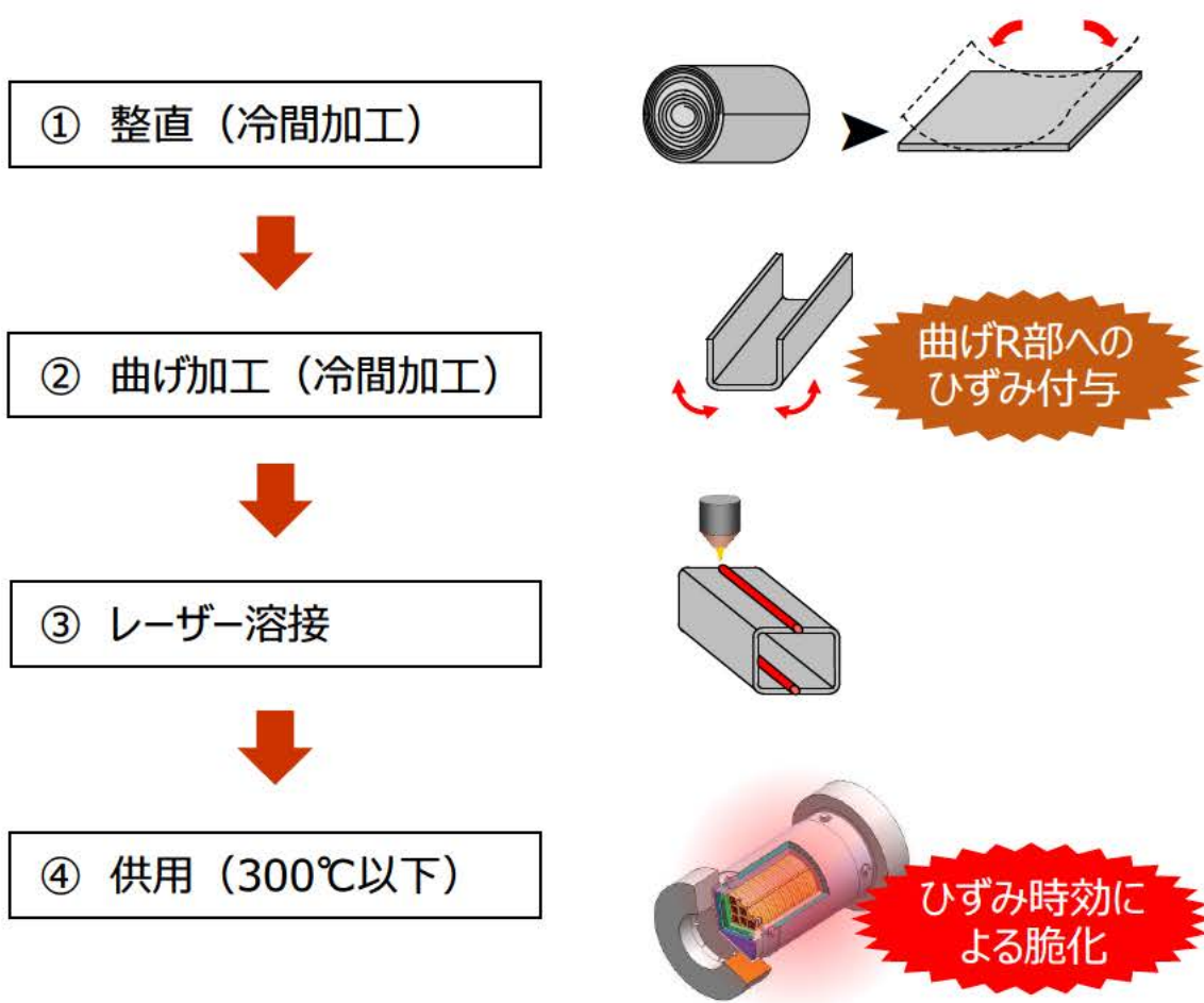
図 別 2-1 コンパートメントの製作及び供用のフロー
