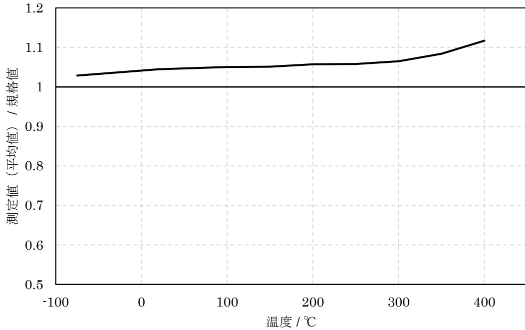
図 別 1-9 縦弾性係数の比較 : SG295 と材料規格分類 [E1-1] (炭素量が 0.3%以下の炭素鋼)
