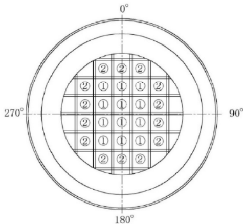
別紙4-1図 燃料の収納条件
