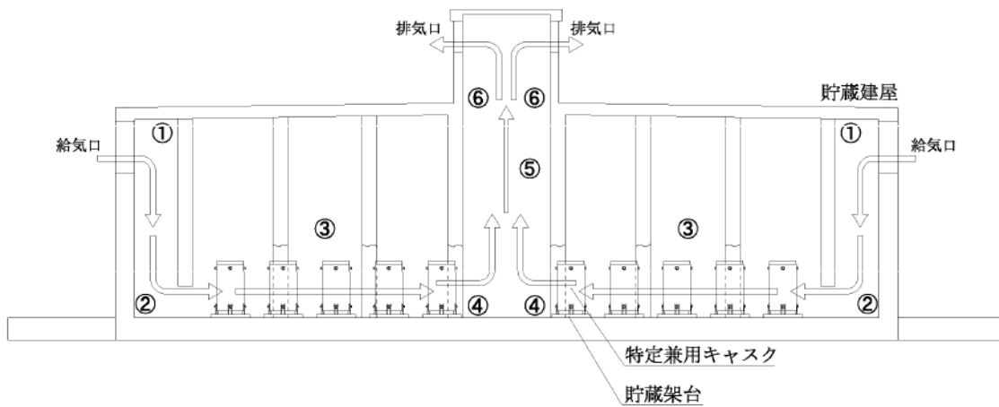
別紙3-1図 貯蔵建屋の熱の流路(例)
