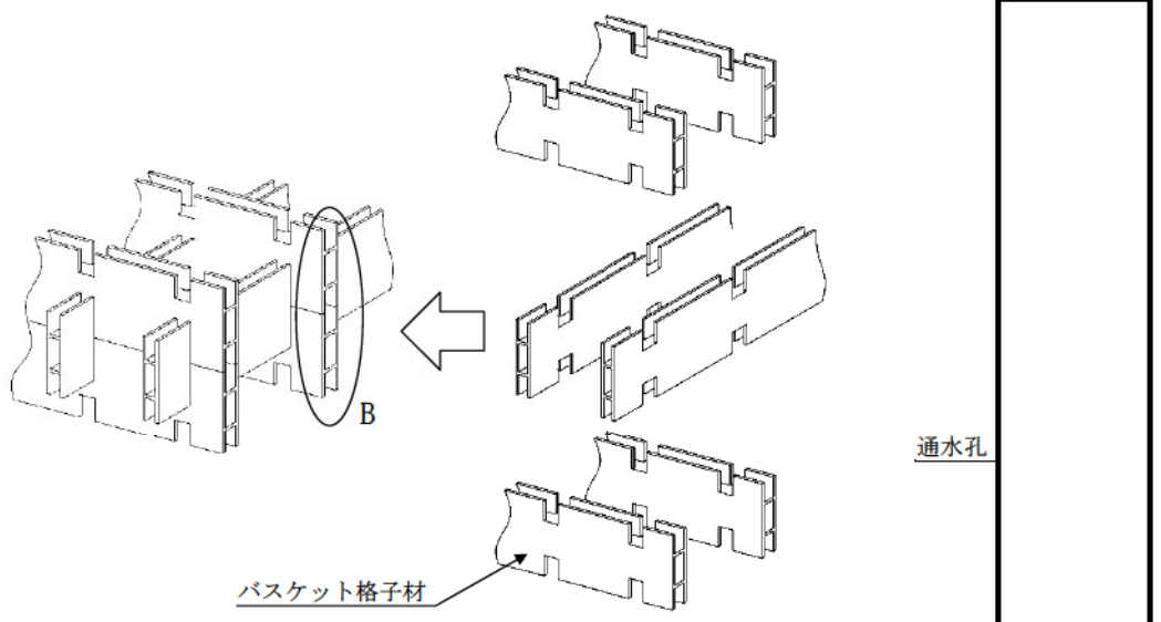
バスケット格子組立図
