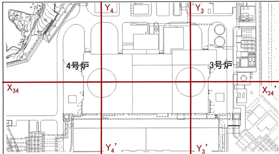
断面位置図
