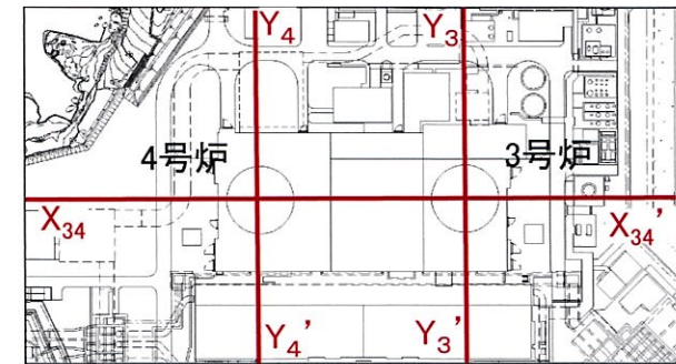
断面位置図
