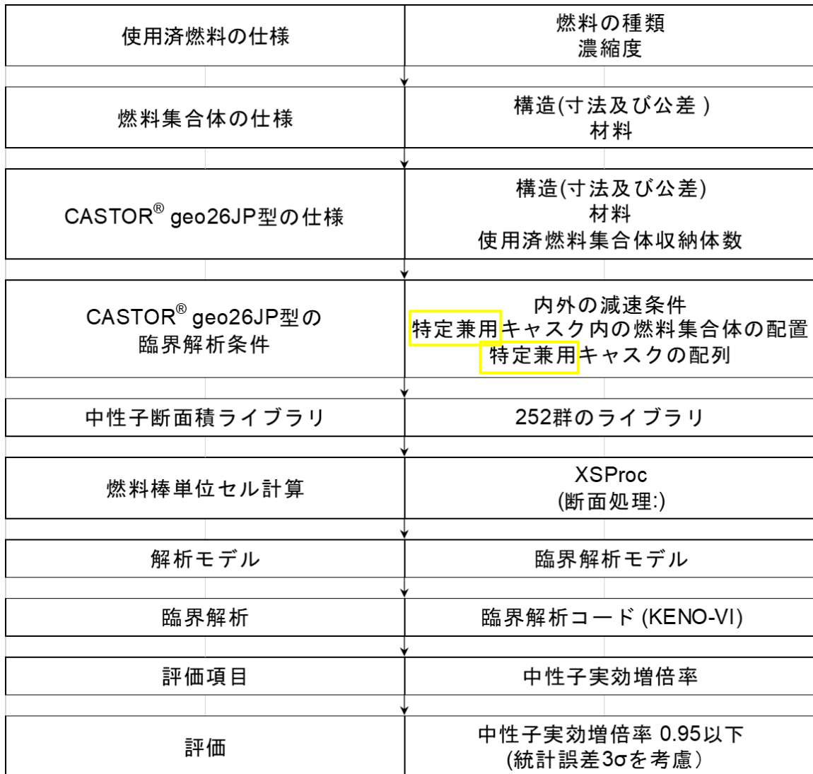
図 2 CASTOR ® geo26JP の臨界解析フロー
