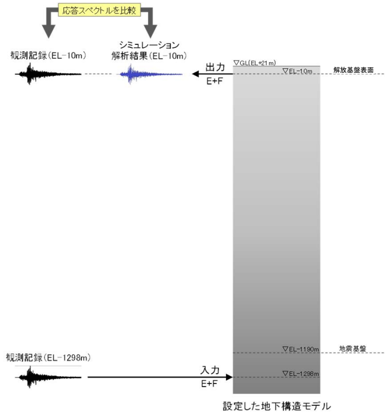
地震動シミュレーションによる地盤増幅特性の検討概要 (3.1.1項)
