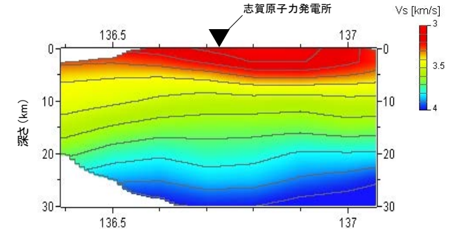
申請後に得られた知見において評価された速度構造
