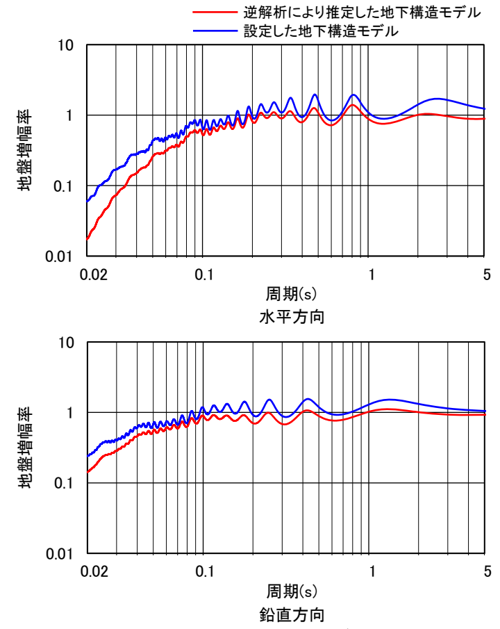
逆解析により推定した地下構造モデルの地盤増幅率と設定した地下構造モデルの地盤増幅率の比較
