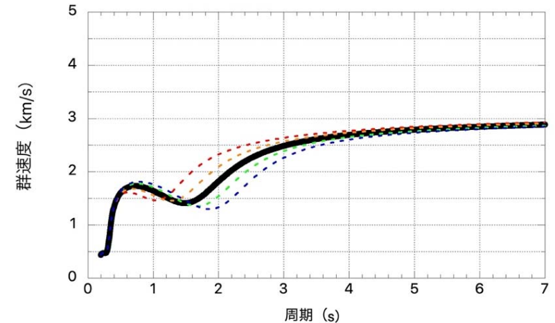
地震基盤の位置を変動させた場合の理論群速度
