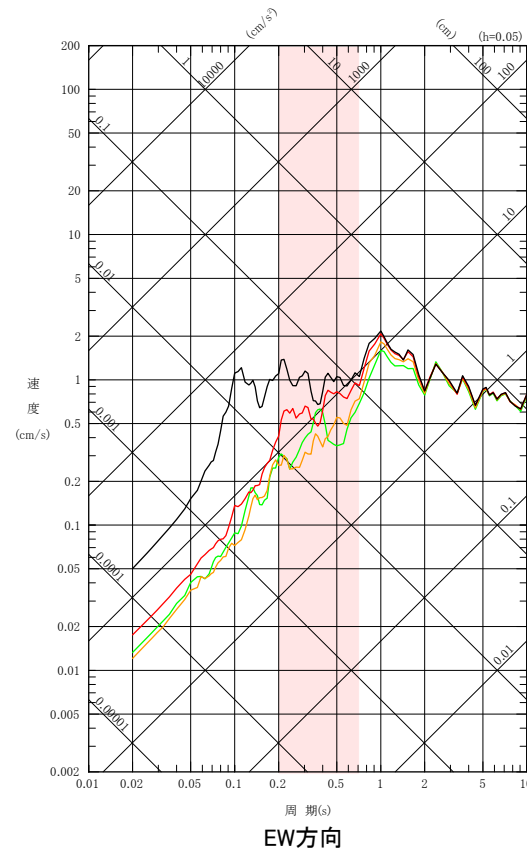
深度別の擬似速度応答スペクトル(No.4(2007年新潟県中越沖地震))
