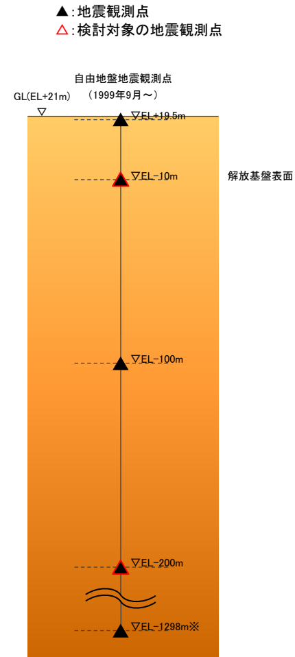
鉛直アレー地震観測点断面図
