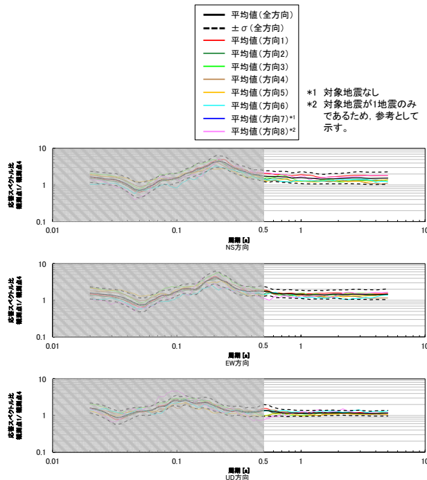
応答スペクトル比(観測点1/観測点4)の地震波の到来方向ごとの比較(1.3.3項)
