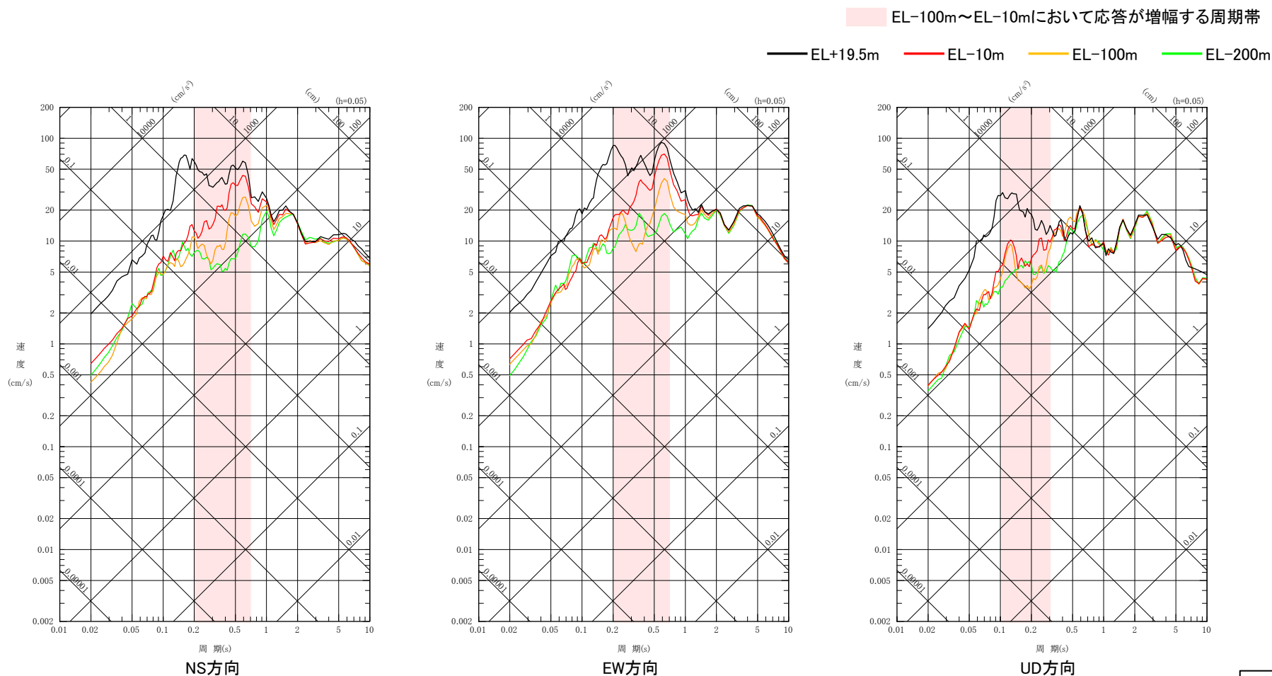
深度別の擬似速度応答スペクトル(No.3(2007年能登半島地震))
