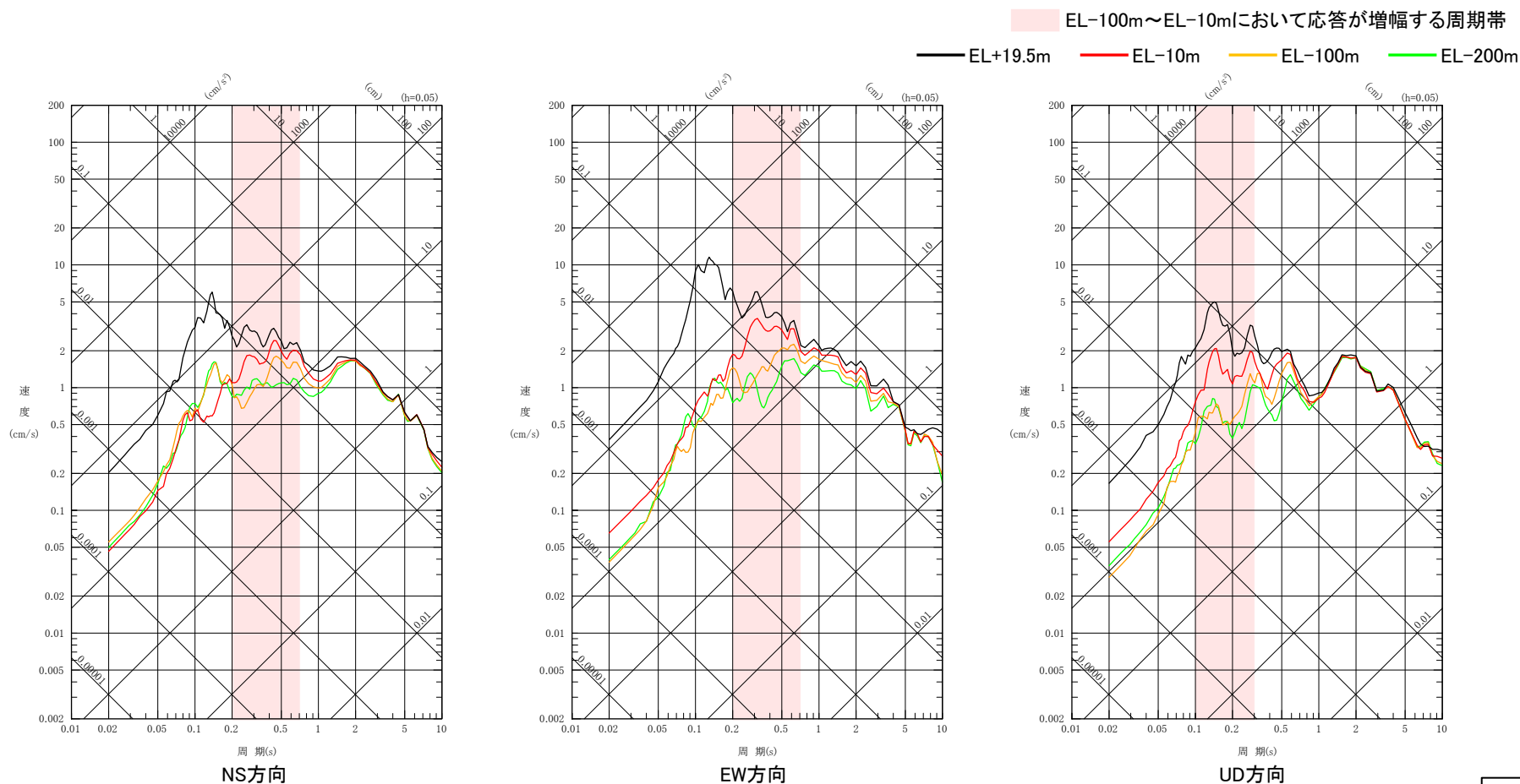
深度別の擬似速度応答スペクトル(No.1(2000/06/07 石川県西方沖の地震))
