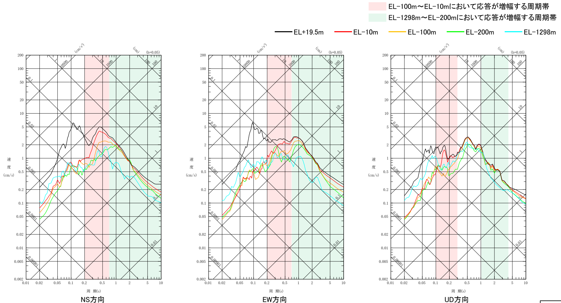
深度別の擬似速度応答スペクトル(No.5(2020/03/13 石川県能登地方の地震))
