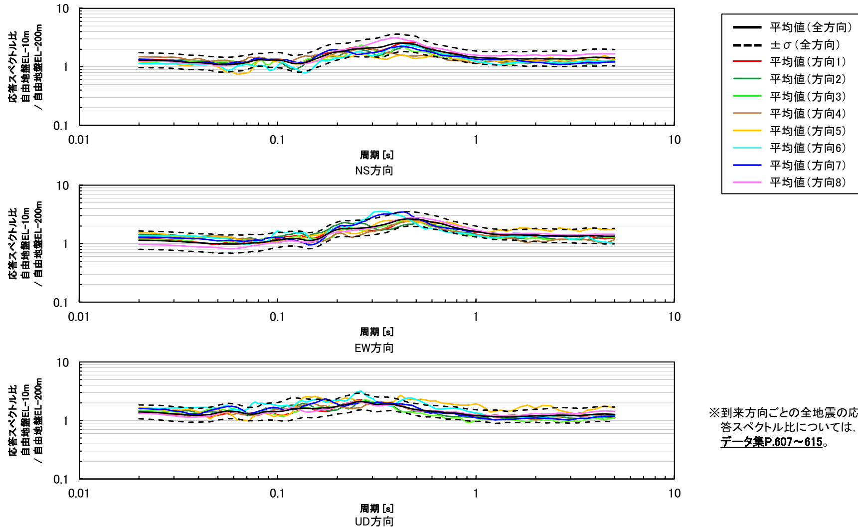
応答スペクトル比(自由地盤EL-10m/自由地盤EL-200m)の地震波の到来方向ごとの比較
