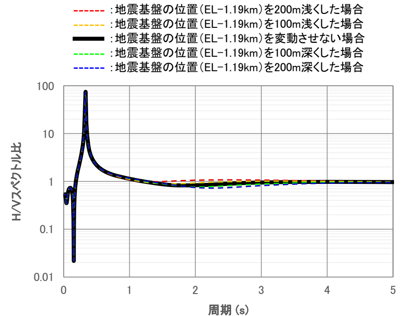
地震基盤の位置を変動させた場合の理論H/Vスペクトル比
