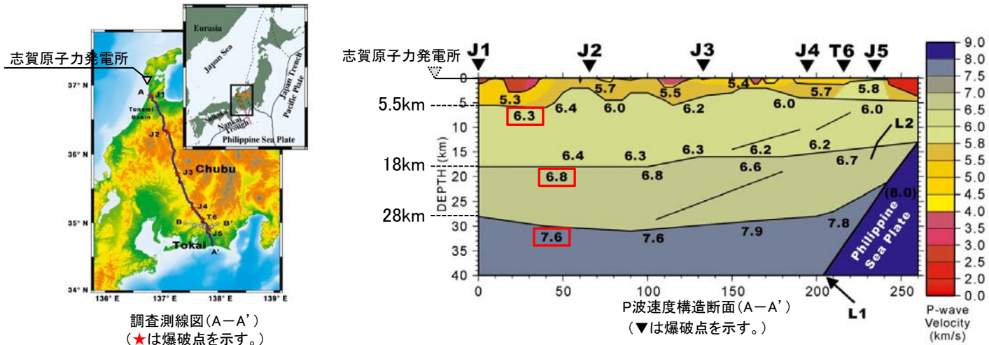
Iidaka et al.(2003)による調査測線図及びP波速度構造断面
