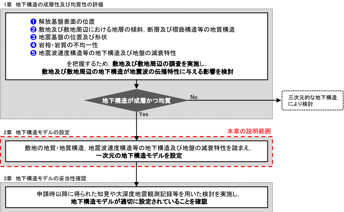
地下構造評価フロー
