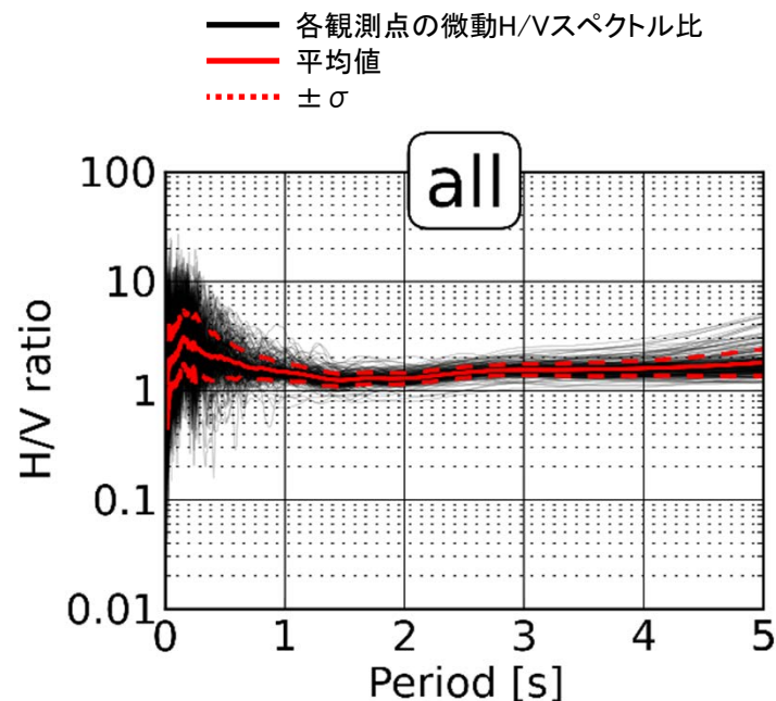
各観測点の微動H/Vスペクトル比の比較
