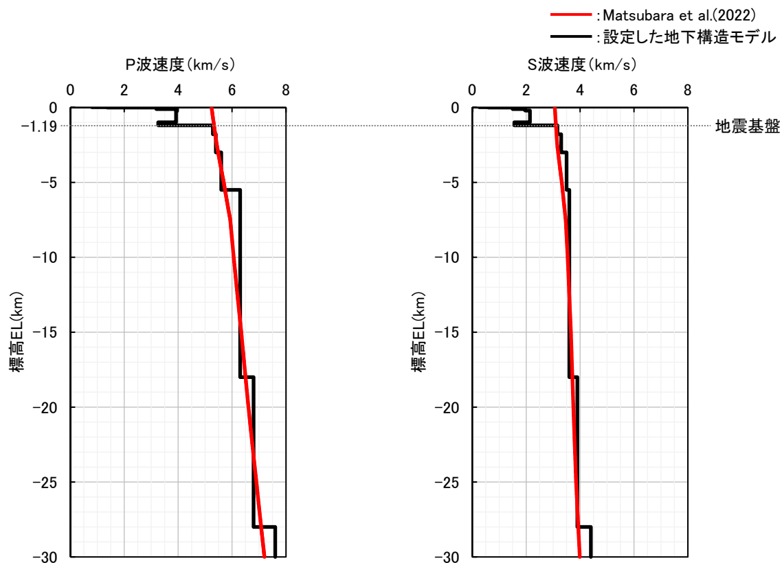
P波速度構造 S波速度構造 Matsubara et al.(2022)により評価された敷地における速度構造と 設定した地下構造モデルの比較
