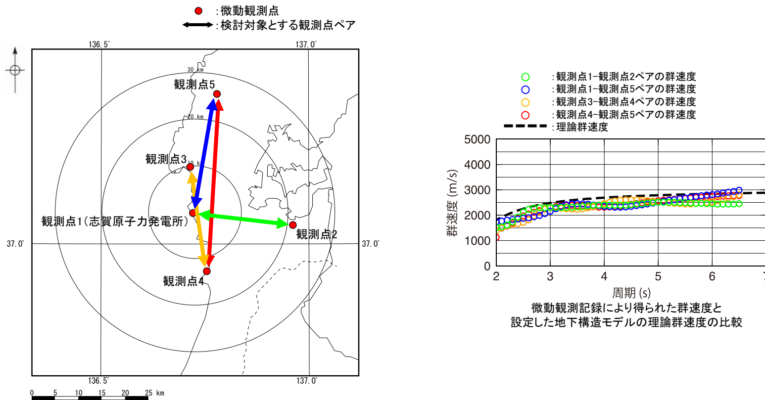
微動観測点配置図
