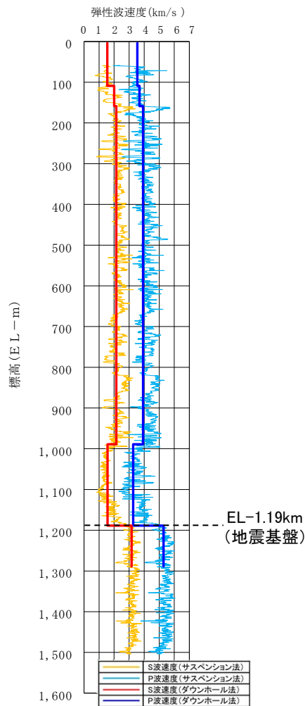
PS検層結果 大深度ボーリング調査結果(D-8.6孔)
