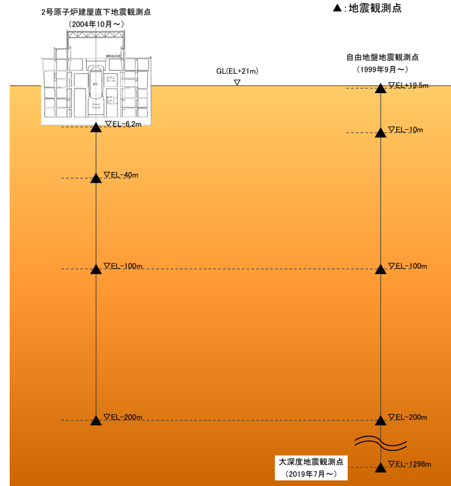
鉛直アレー地震観測点断面図
