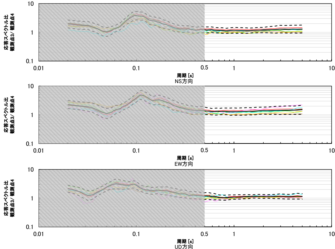
応答スペクトル比(観測点3/観測点4)の地震波の到来方向ごとの比較
