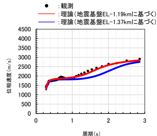
A地点の分散曲線
