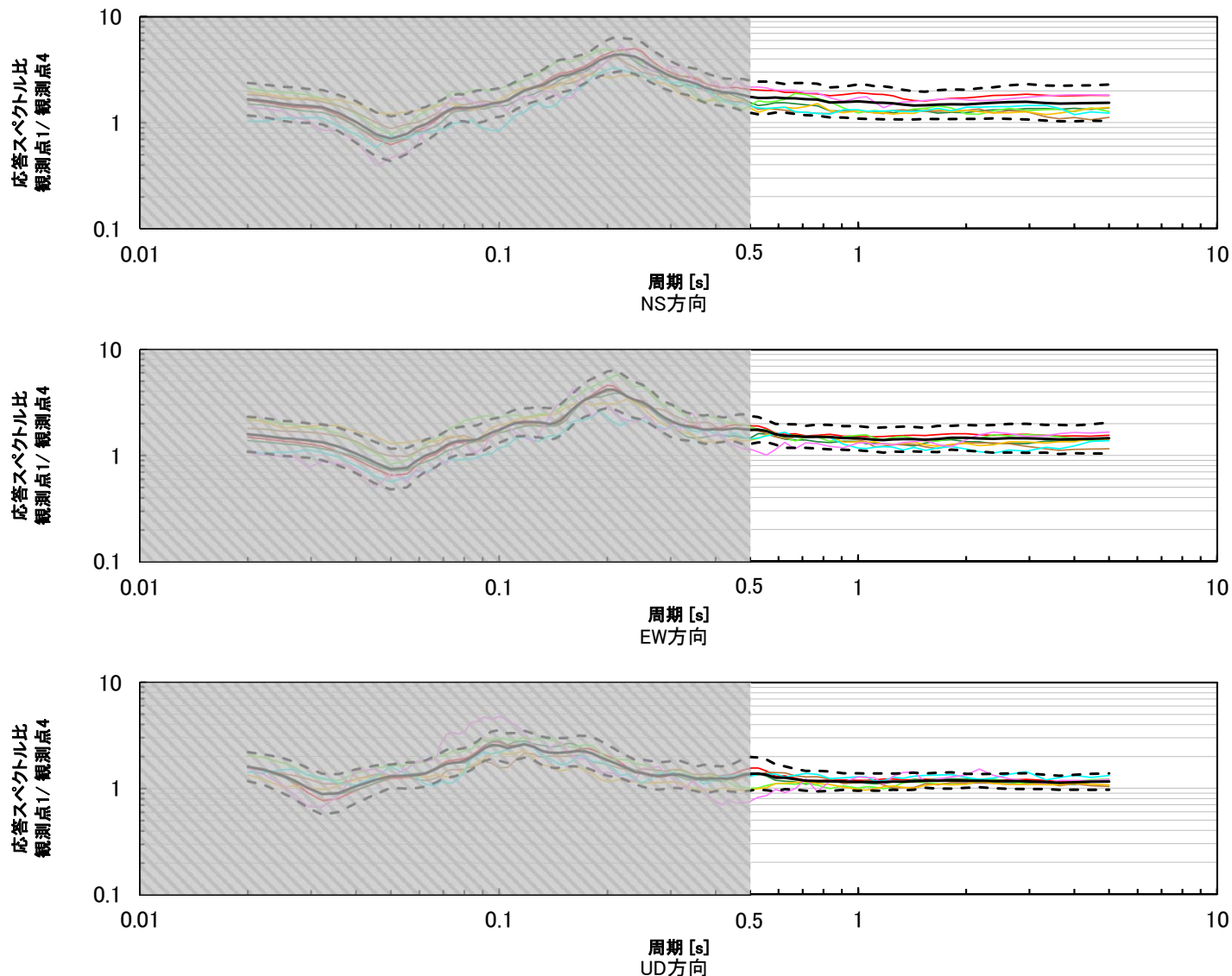
応答スペクトル比(観測点1/観測点4)の地震波の到来方向ごとの比較
