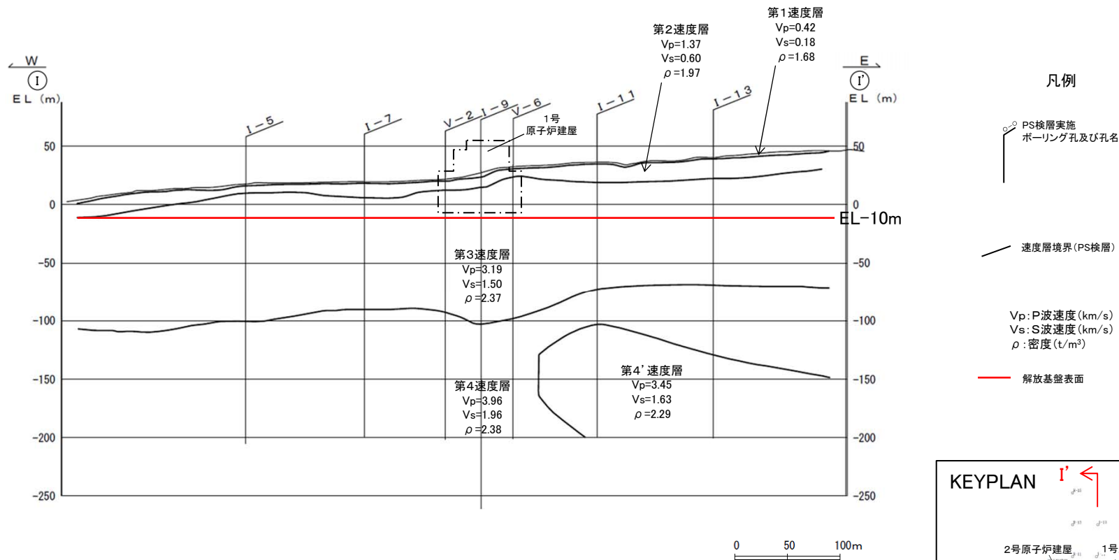
速度構造及び密度構造断面 (I-I' 断面)※
