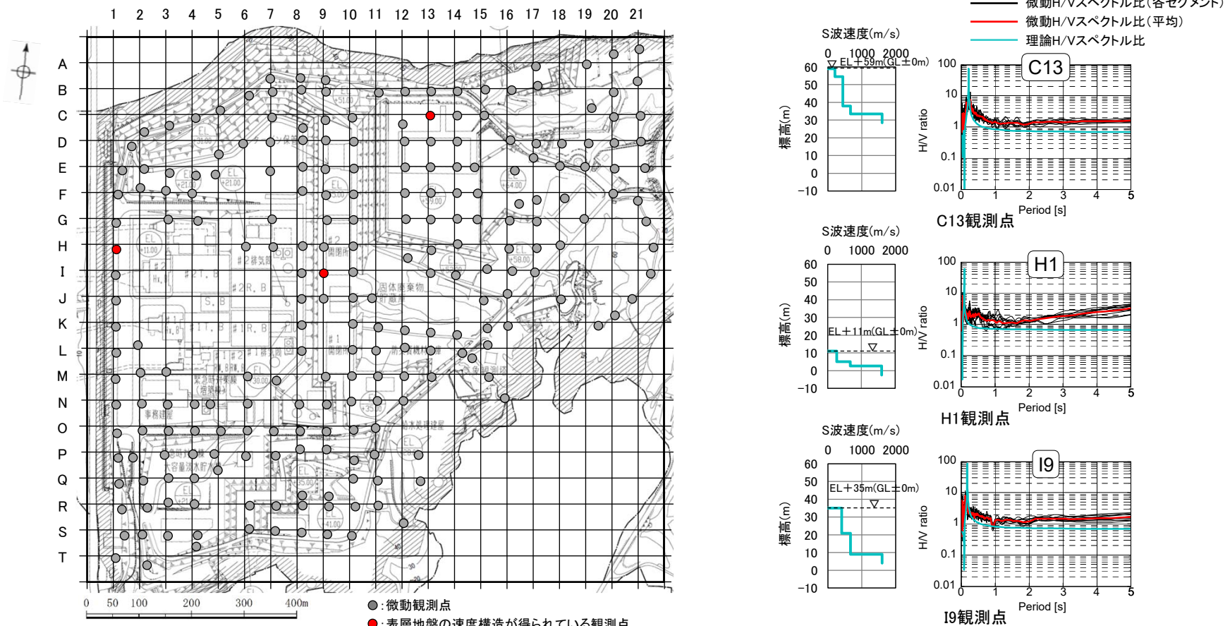
比較の対象とした観測点の表層地盤の速度構造(左)と 微動H/Vスペクトル比と理論H/Vスペクトル比の比較(右)
