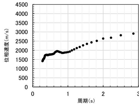
敷地における微動アレー探査により得られた位相速度
