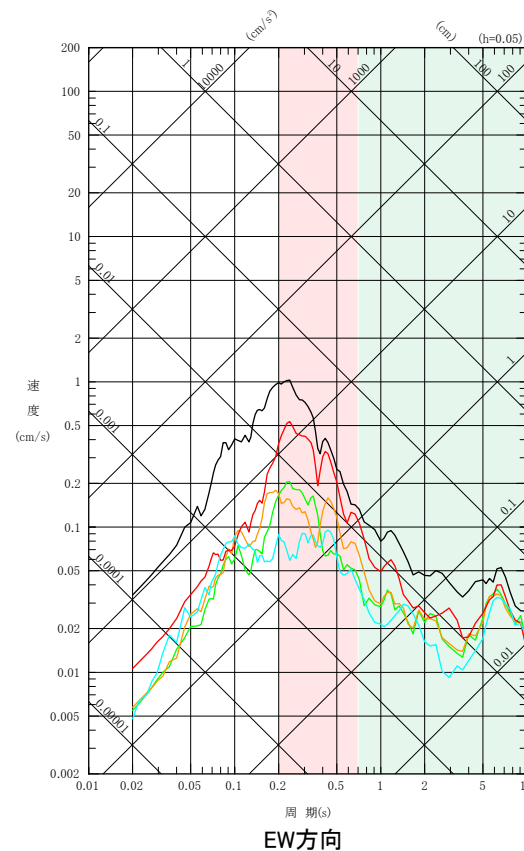
深度別の擬似速度応答スペクトル(No.10(2023/05/05 14:53 石川県能登地方の地震))
