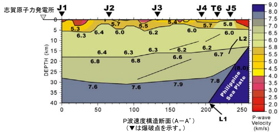
Iidaka et al.(2003)による調査測線図及びP波速度構造断面 ※ Iidaka et al.(2003)に一部加筆
