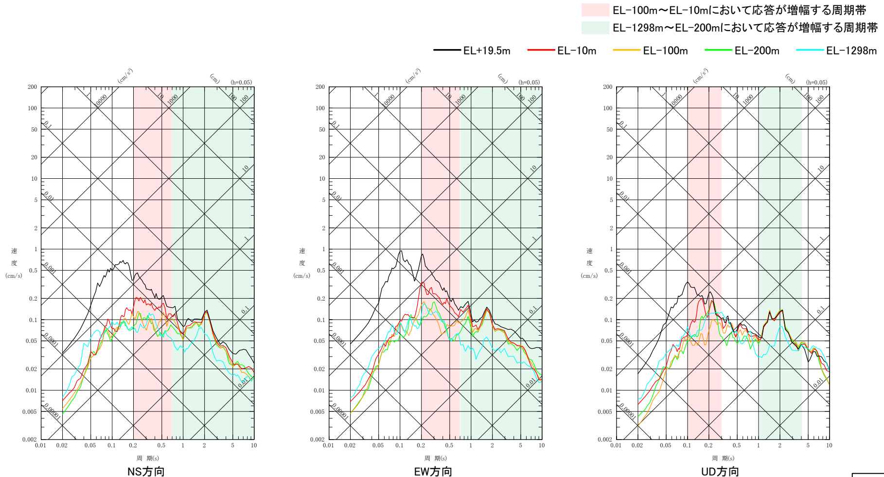
深度別の擬似速度応答スペクトル(No.6(2021/09/16 石川県能登地方の地震))
