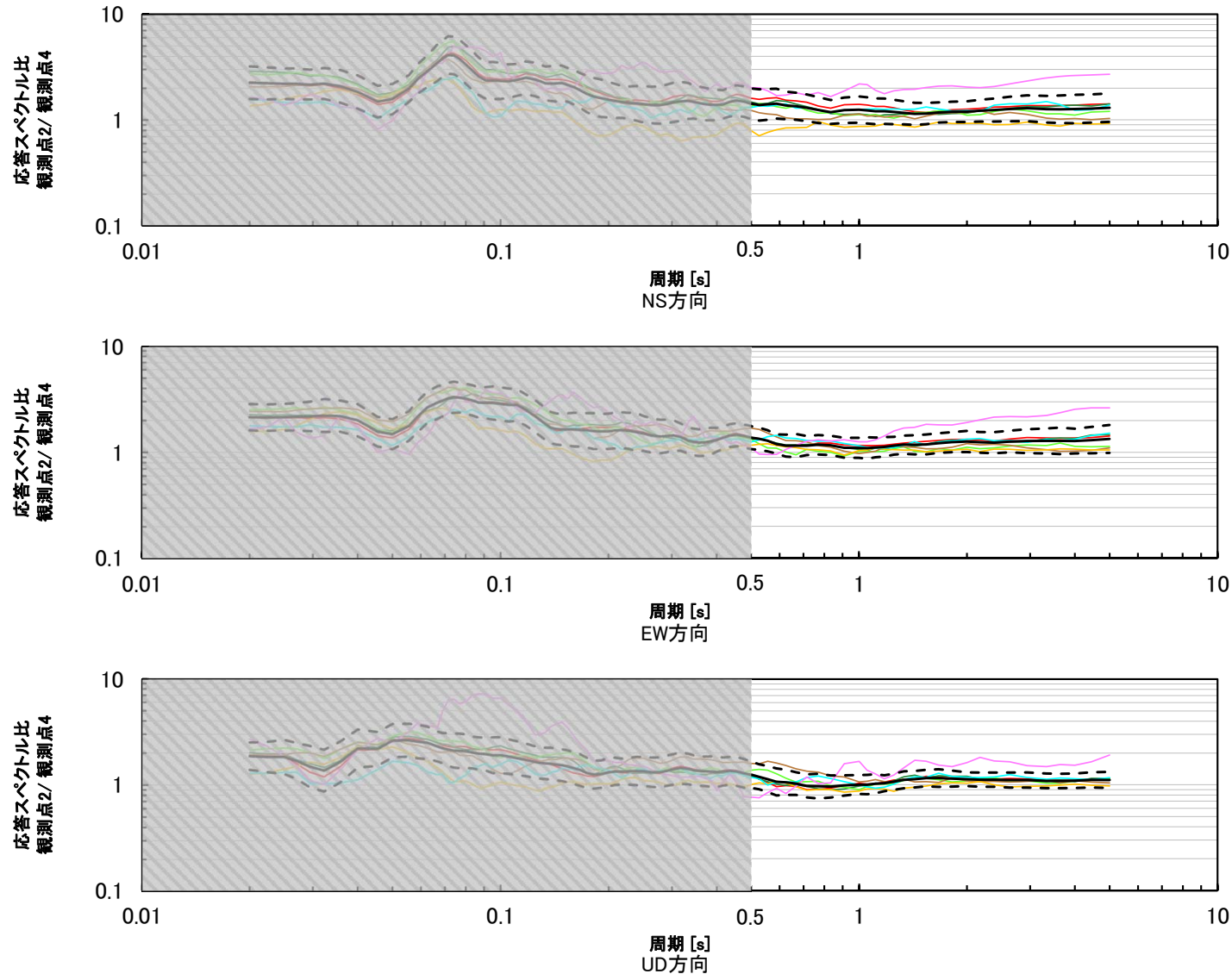
応答スペクトル比(観測点2/観測点4)の地震波の到来方向ごとの比較
