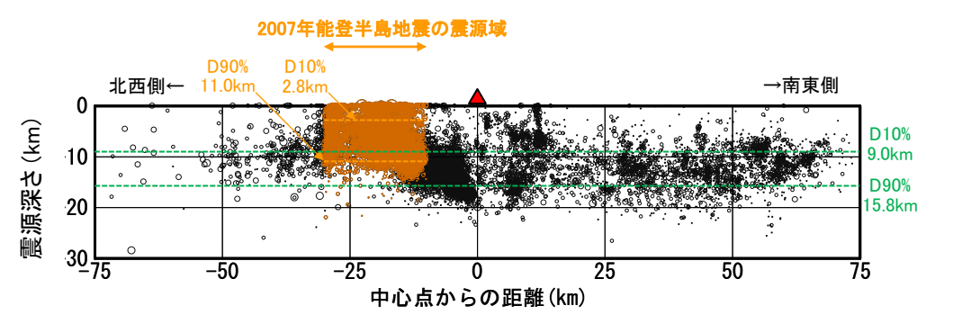
2007年能登半島地震発生日以後を含む地震の震源深さ分布図(1997年10月～2022年3月)
