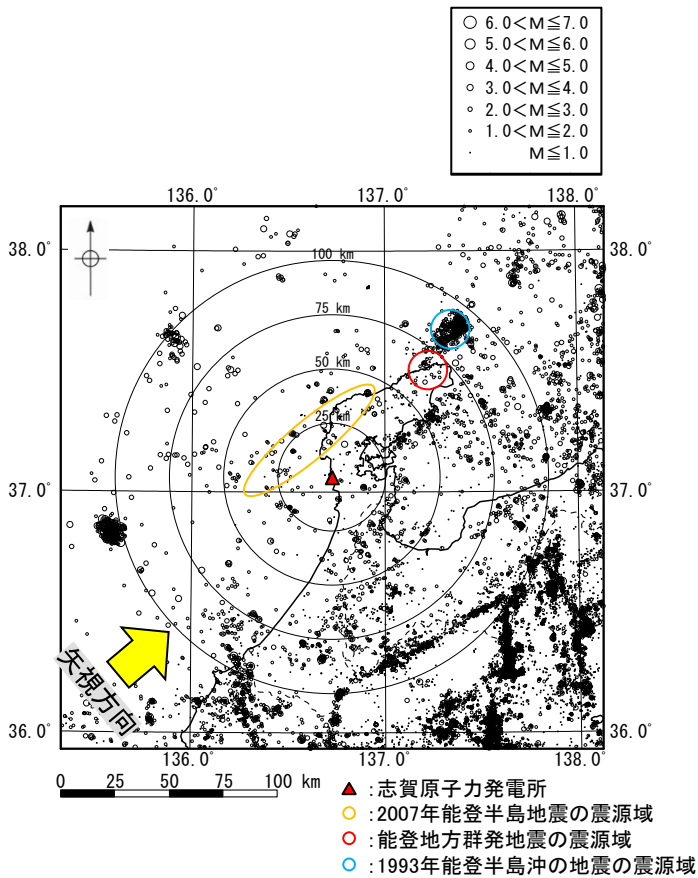
2007年能登半島地震発生日より前の地震の震央分布図(1997年10月～2007年3月24日)
