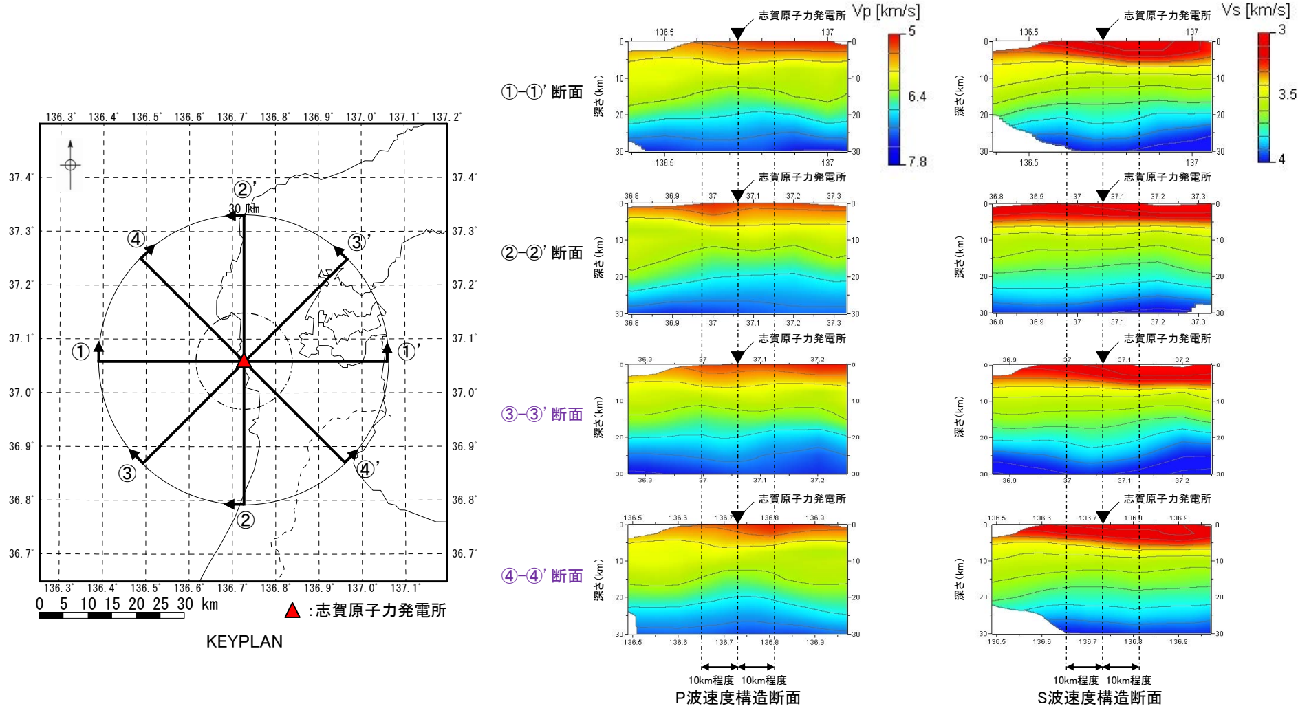
Matsubara et al.(2022)による敷地周辺の速度構造断面
