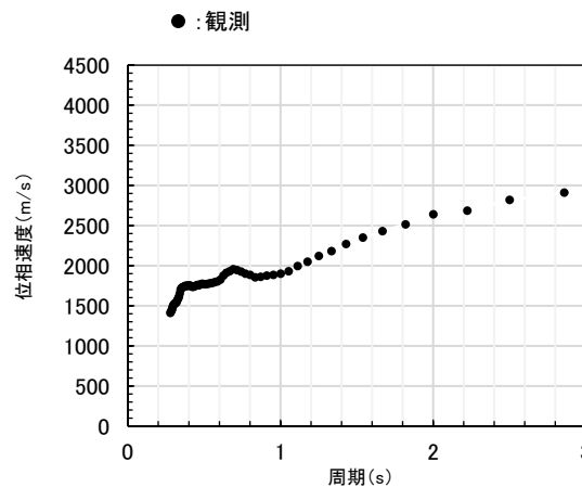
A地点の分散曲線
