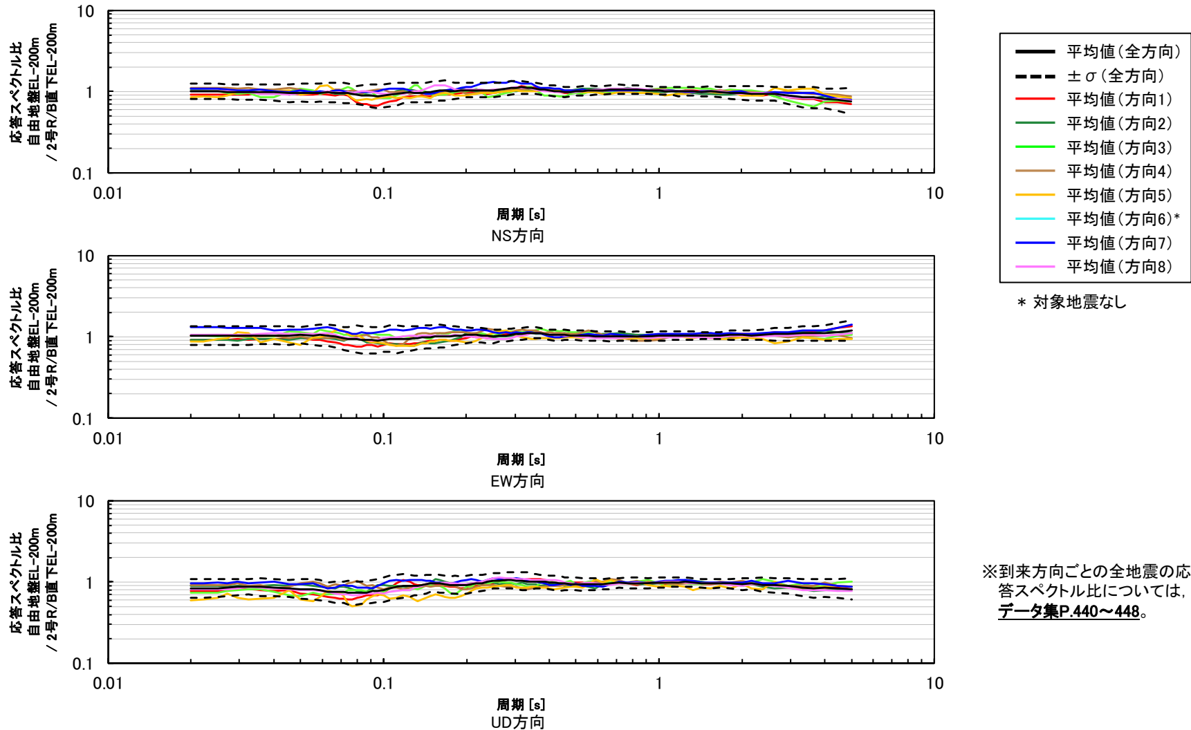
応答スペクトル比(自由地盤EL-200m/2号原子炉建屋直下EL-200m)の地震波の到来方向ごとの比較
