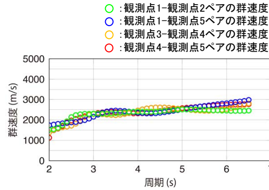
敷地周辺の微動観測記録により得られた群速度
