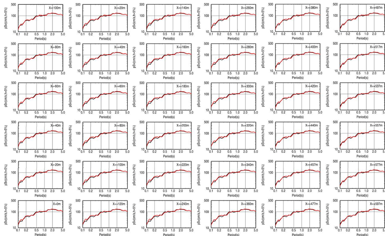
各評価地点の応答スペクトル
