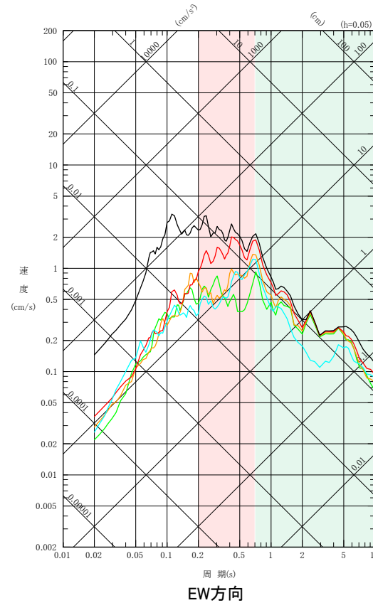
深度別の擬似速度応答スペクトル(No.11(2023/05/05 21:58 石川県能登地方の地震))
