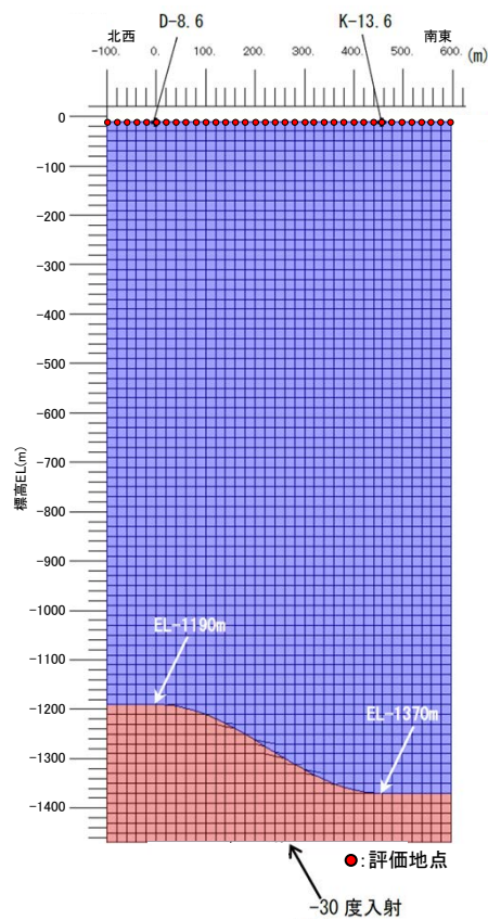
花崗岩上面の高度差をモデル化した 二次元FEMモデル
