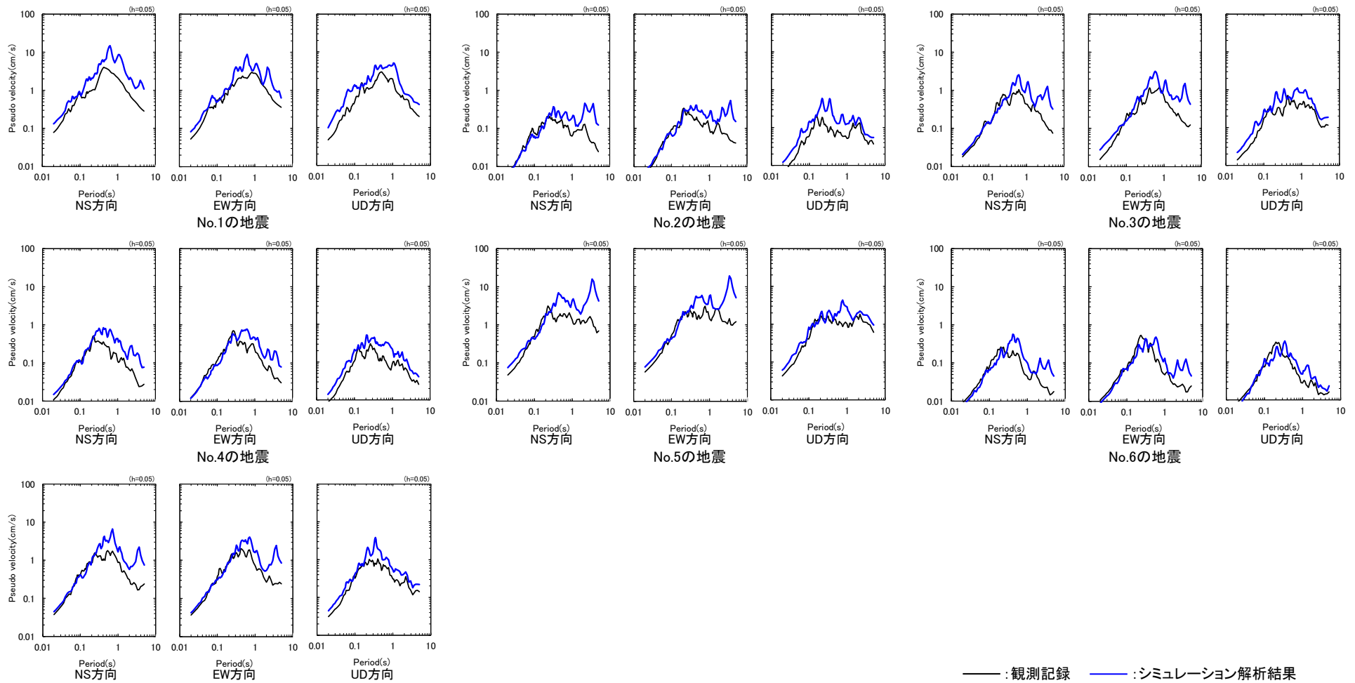
シミュレーション解析結果と観測記録の比較
