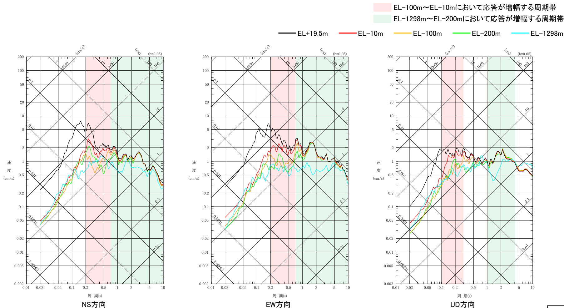
深度別の擬似速度応答スペクトル(No.9(2023/05/05 14:42 石川県能登地方の地震))
