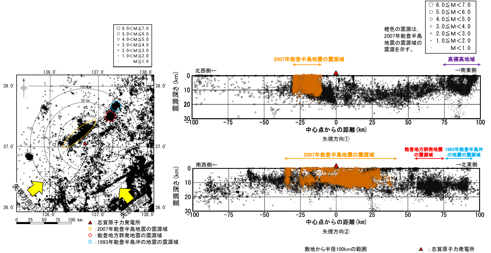
地震の震央分布図(1997年10月~2022年3月)
