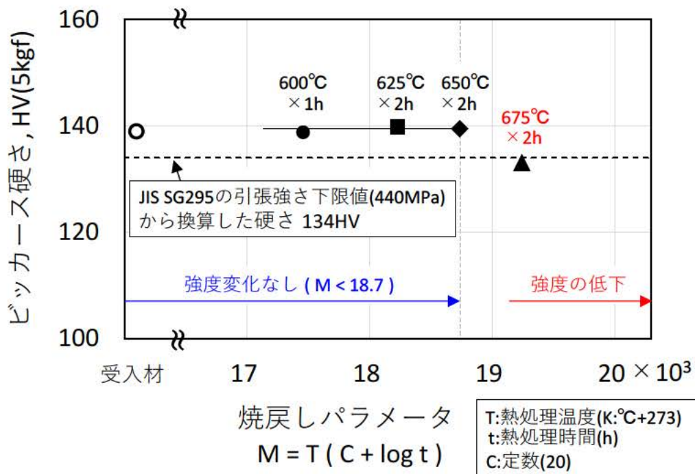
図 別 2-3 受入材と熱処理材のビッカース硬さ
