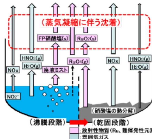
蒸発乾固時の事象進展に応じた放射性物質等の移行挙動の概念図 [1]
