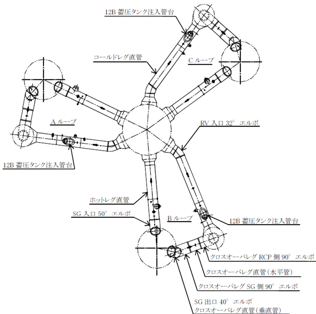
図3 1次冷却材管の熱時効評価対象部位
