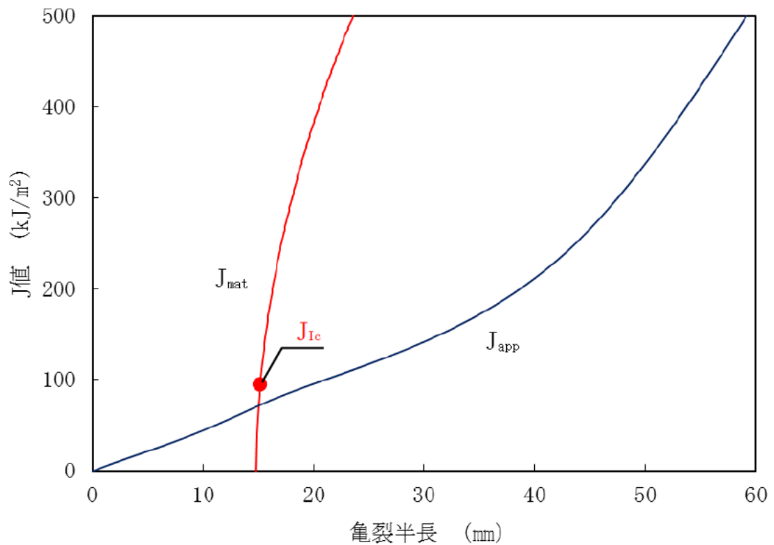
図9 蓄圧タンク注入ライン管台の亀裂安定性評価線図
