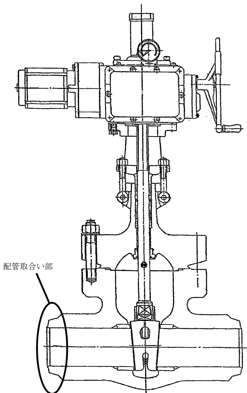
図1 余熱除去ポンプCループ側入口隔離弁の構造図
