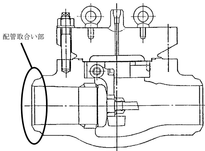
図1 蓄圧タンク出口第2逆止弁の構造図
