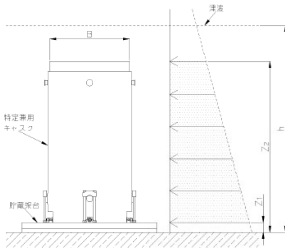
図2 津波波力の評価モデル
