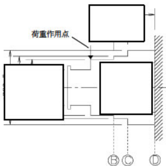
(a) 下部トラニオン (90° - 270° 側)
