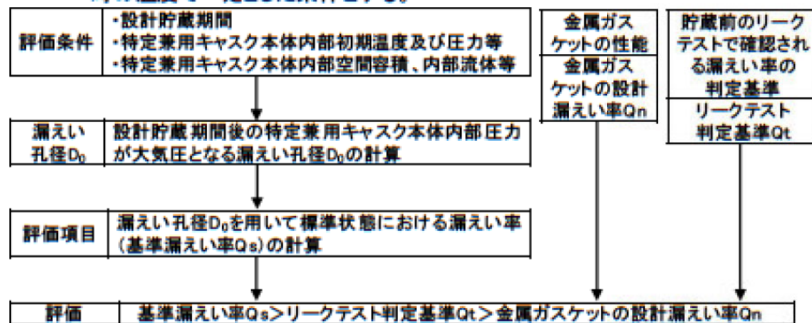
[閉じ込め機能評価フロー]
