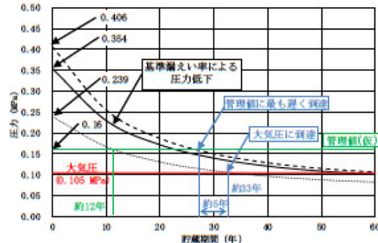
[貯蔵期間中の蓋間圧力の管理値設定例]
