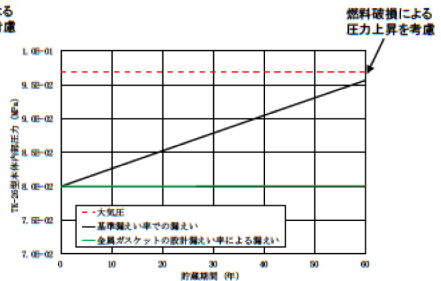
15×15燃料収納時
