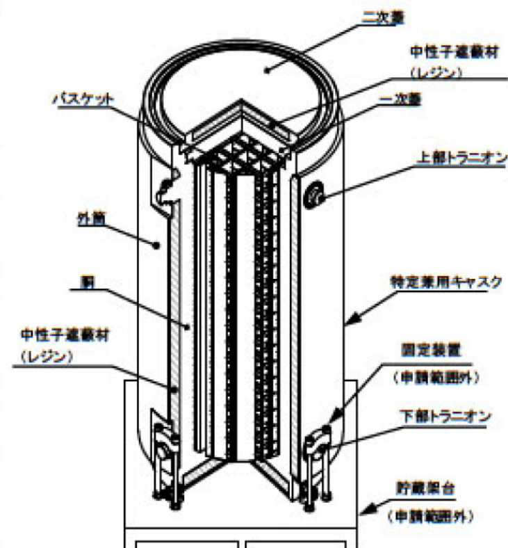
➤ TK-26型の構造図
