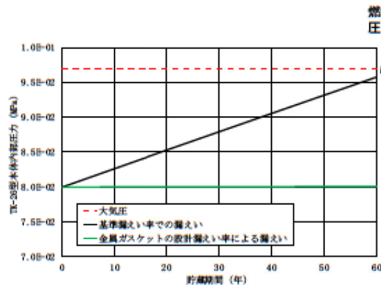
17×17燃料収納時
