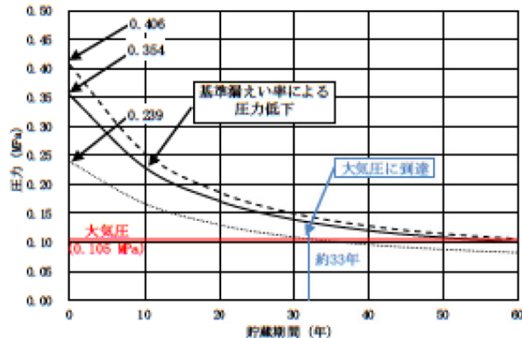
[金属ガスケットの基準漏えい率による蓋間圧力の経時変化]
