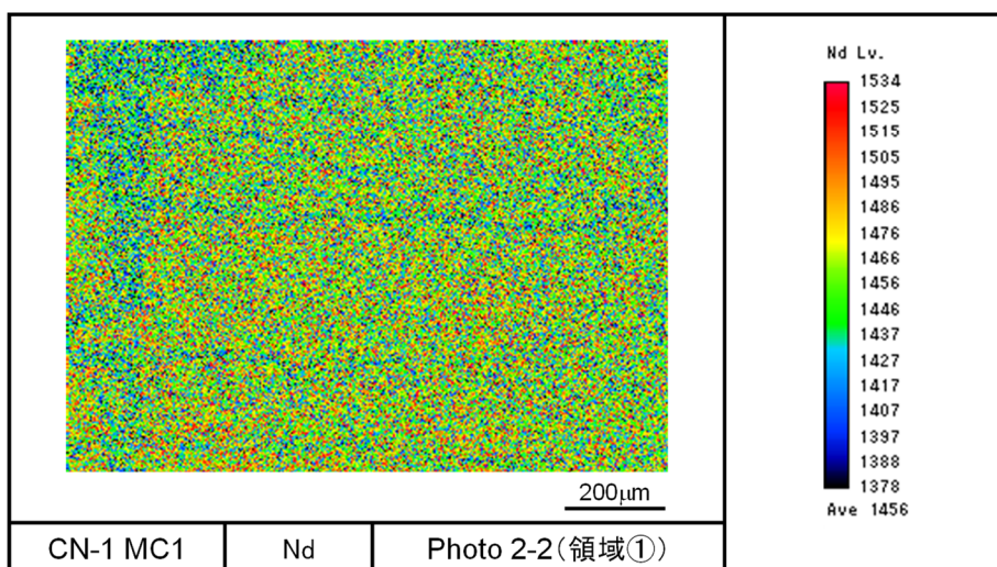
図 4.4.2-10(3) CN-1 燃料ペレット EPMA 写真 (領域①、カラスケール調整)
