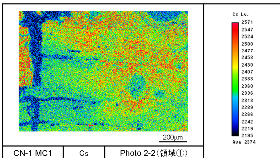
図 4.4.2-10(4) CN-1 燃料ペレット EPMA 写真 (領域①、カラスケール調整)
