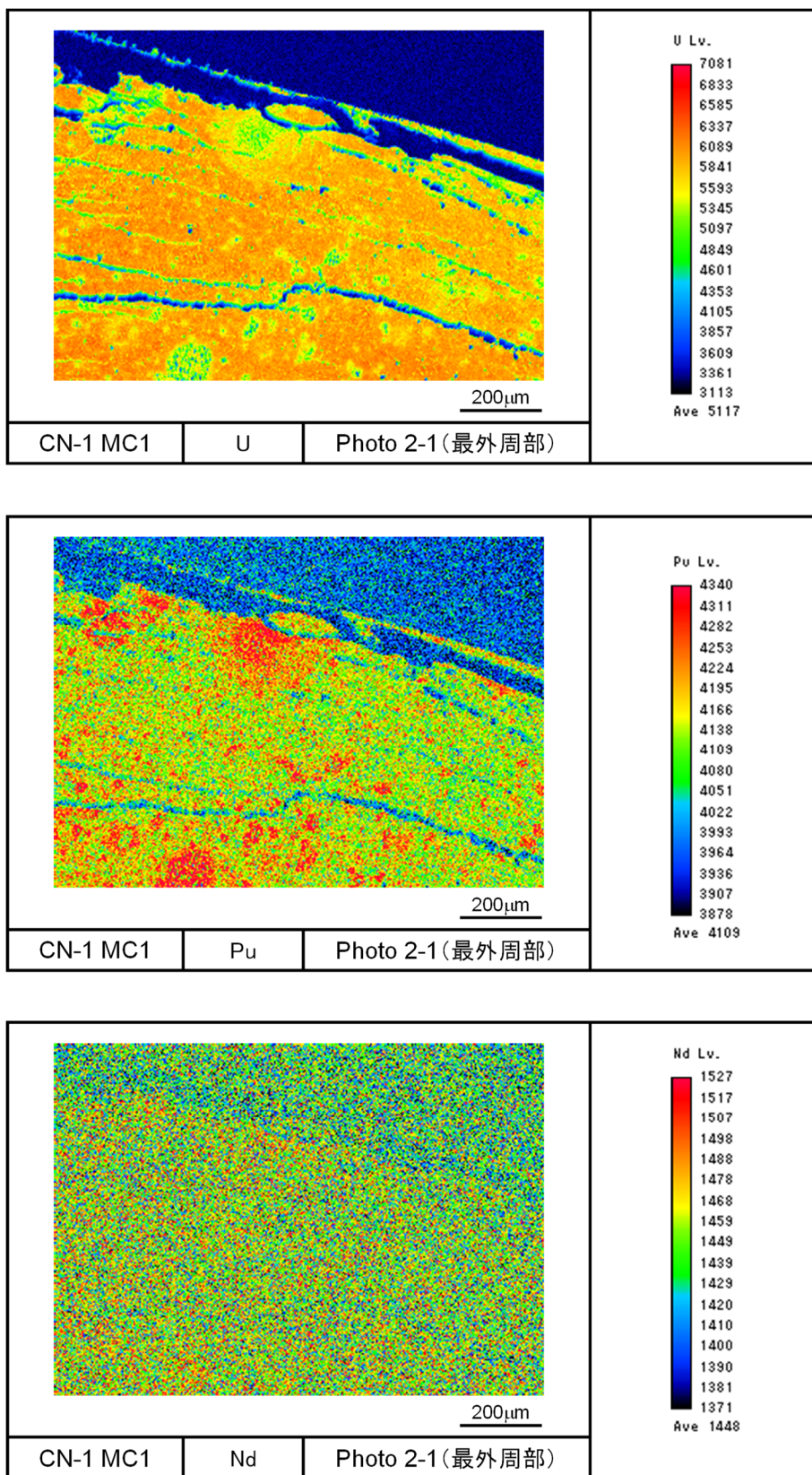
図 4.4.2-10(1) CN-1 燃料ペレット EPMA 写真 (最外周部、カラースケール調整)
