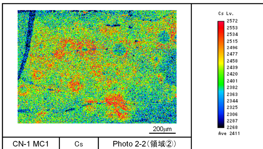
図 4.4.2-10(6) CN-1 燃料ペレット EPMA 写真 (領域②、カラスケール調整)
