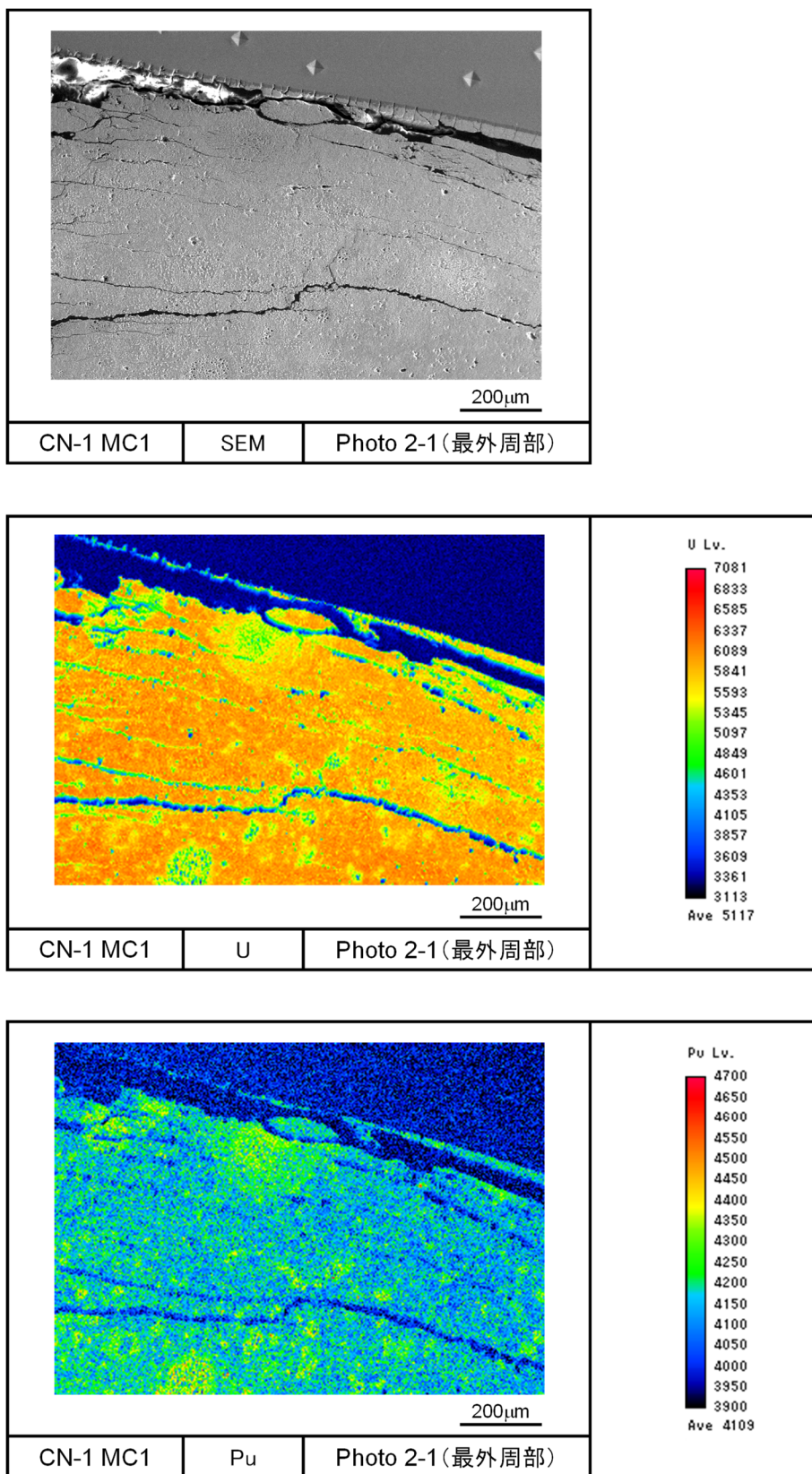
図 4.4.2-9(1) CN-1 燃料ペレット EPMA 写真 (最外周部、カラスケール統一)
