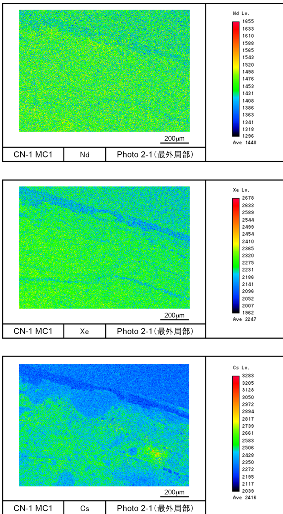
図 4.4.2-9(2) CN-1 燃料ペレット EPMA 写真 (最外周部、カラスケール統一)
