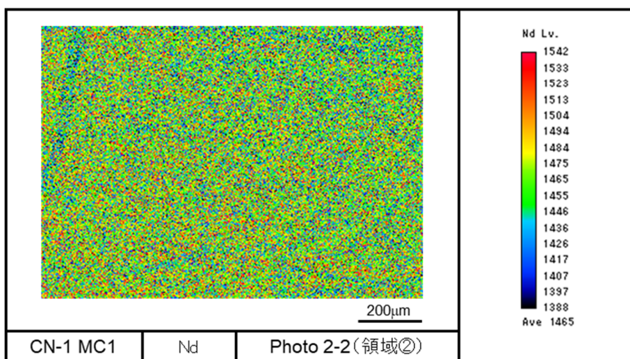
図 4.4.2-10(5) CN-1 燃料ペレット EPMA 写真 (領域②、カラスケール調整)
