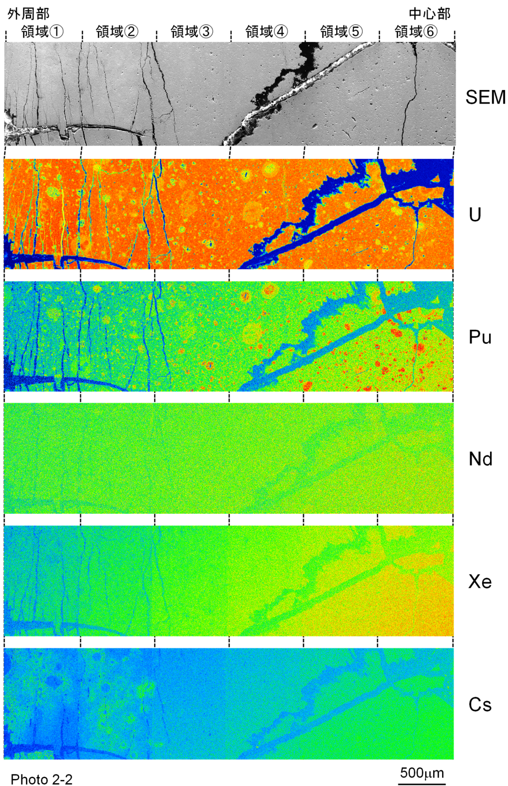
図 4.4.2-9(3) CN-1 燃料ペレット EPMA 写真 (外周部～中心部、カラースケール統一)
