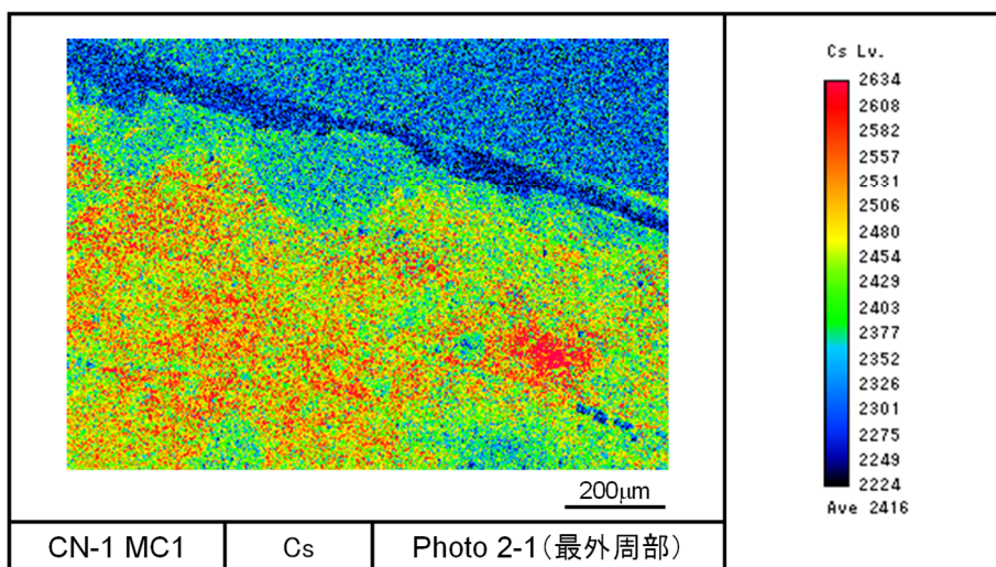
図 4.4.2-10(2) CN-1 燃料ペレット EPMA 写真 (最外周部、カラスケール調整)
