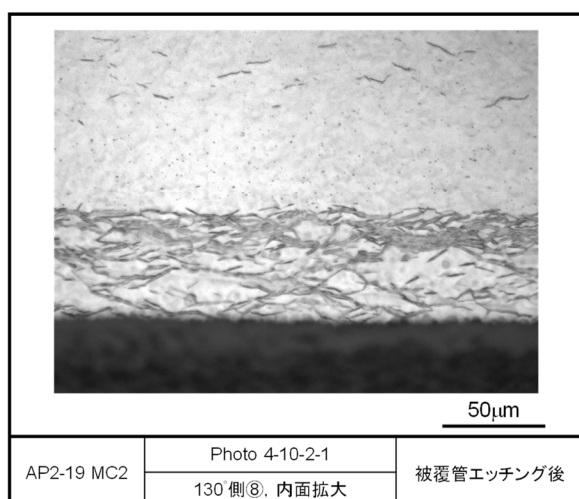
図 4.2.1-5(7) レファレンス試料の金相写真 (被覆管エッチング後, AP2-19 MC2)
