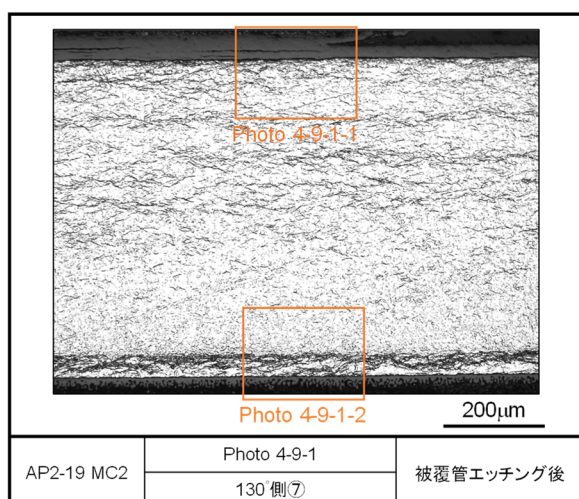
図 4.2.1-5(6) レファレンス試料の金相写真 (被覆管エッチング後, AP2-19 MC2)
