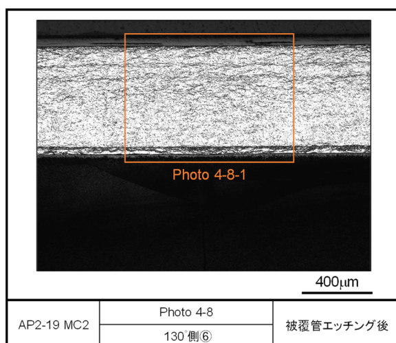
図 4.2.1-5(5) レファレンス試料の金相写真（被覆管エッチング後，AP2-19 MC2）
