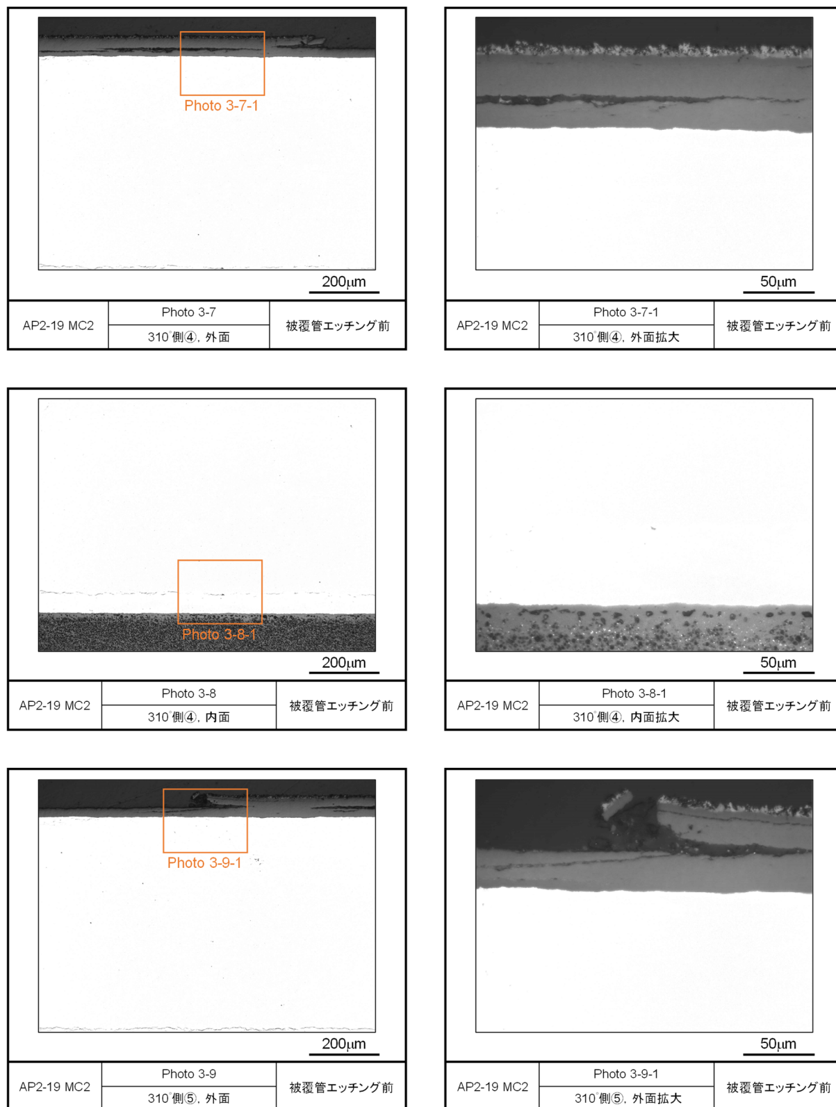
図 4.2.1-4(4) レファレンス試料の金相写真（被覆管エッチング前，AP2-19 MC2）
