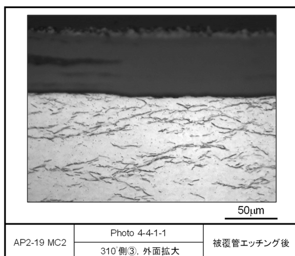
図 4.2.1-5(3) レファレンス試料の金相写真 (被覆管エッチング後, AP2-19 MC2)
