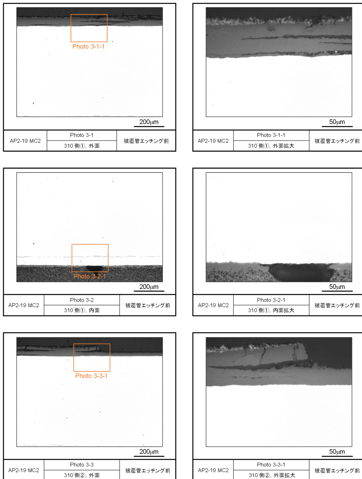
図 4.2.1-4(2) レファレンス試料の金相写真（被覆管エッチング前，AP2-19 MC2）
