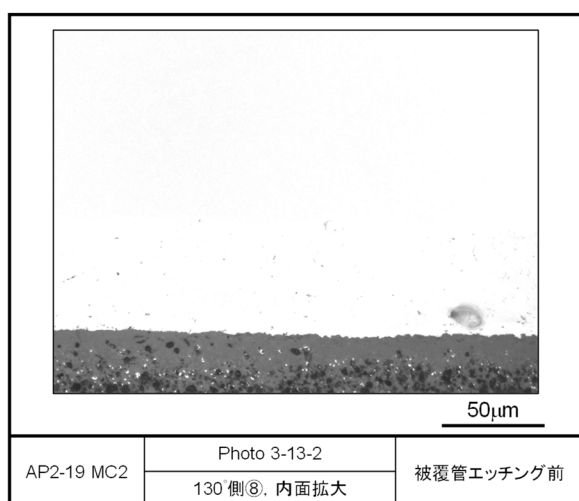
図 4.2.1-4(6) レファレンス試料の金相写真（被覆管エッチング前，AP2-19 MC2）
