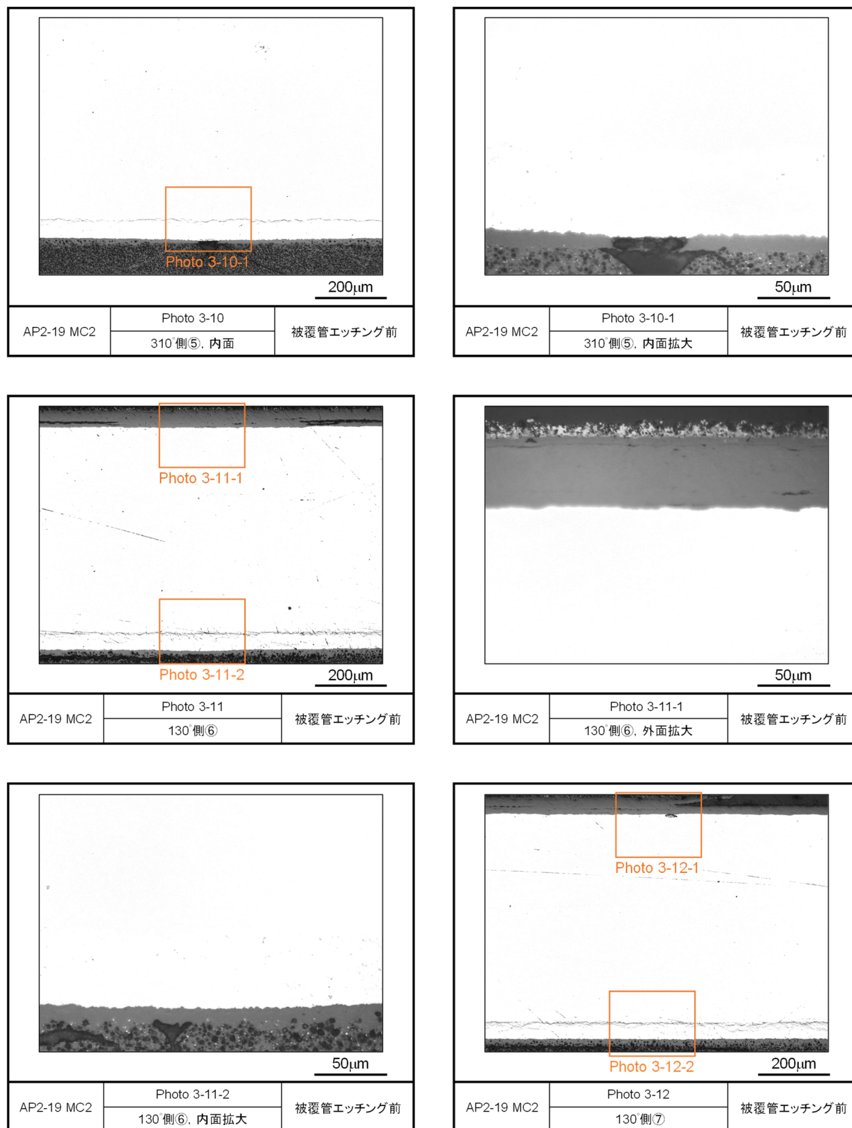
図 4.2.1-4(5) レファレンス試料の金相写真（被覆管エッチング前，AP2-19 MC2）
