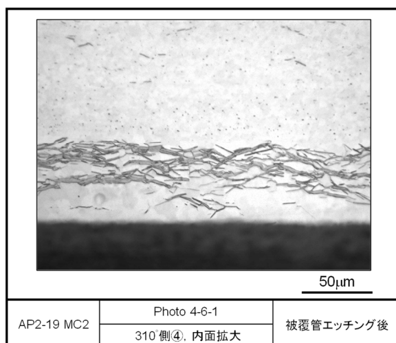
図 4.2.1-5(4) レファレンス試料の金相写真 (被覆管エッチング後, AP2-19 MC2)
