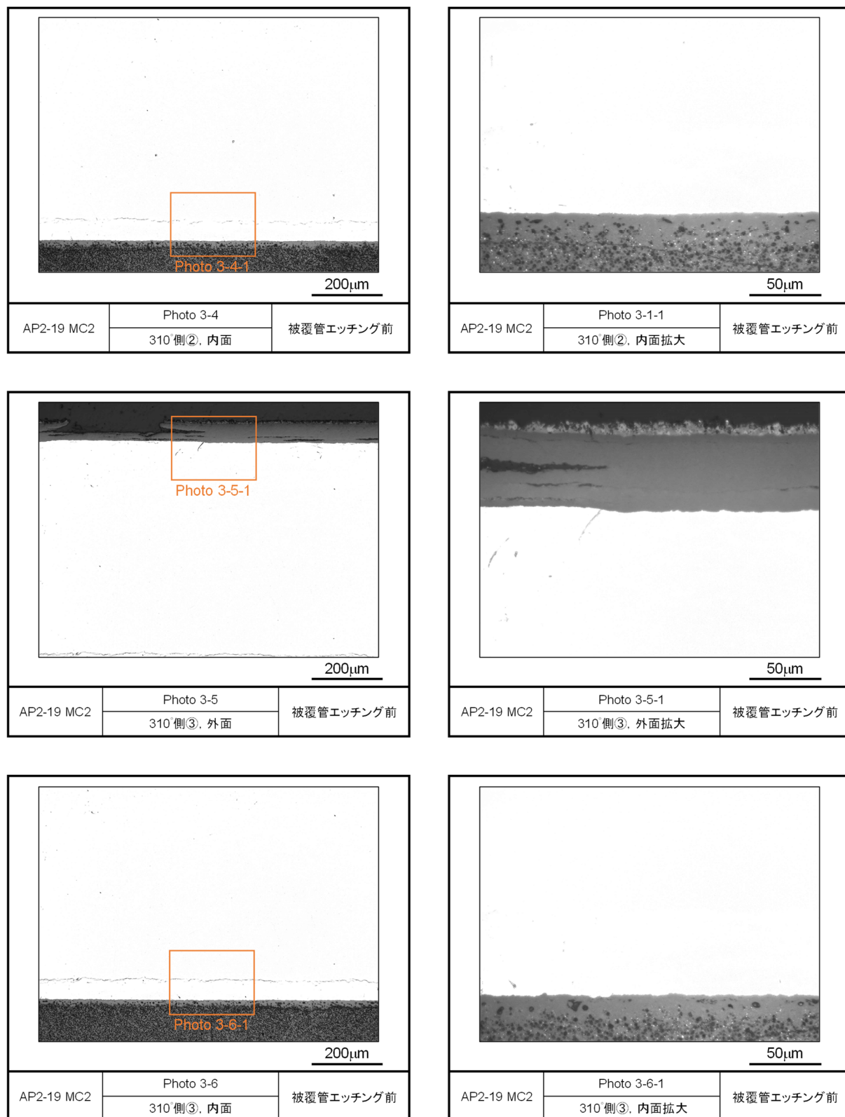
図 4.2.1-4(3) レファレンス試料の金相写真（被覆管エッチング前，AP2-19 MC2）
