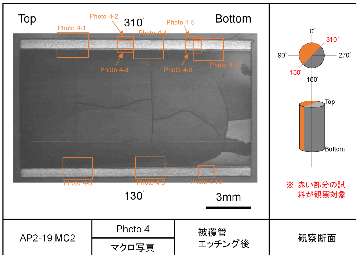
図 4.2.1-5(1) レファレンス試料の金相写真（被覆管エッチング後，AP2-19 MC2）
