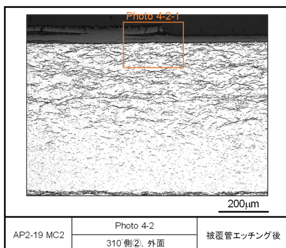
図 4.2.1-5(2) レファレンス試料の金相写真 (被覆管エッチング後, AP2-19 MC2)
