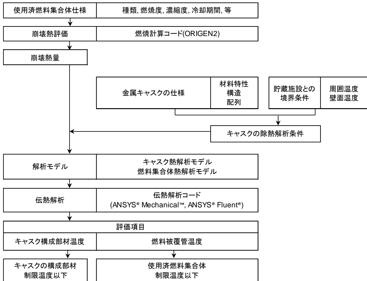
図 2 除熱評価のフロー
