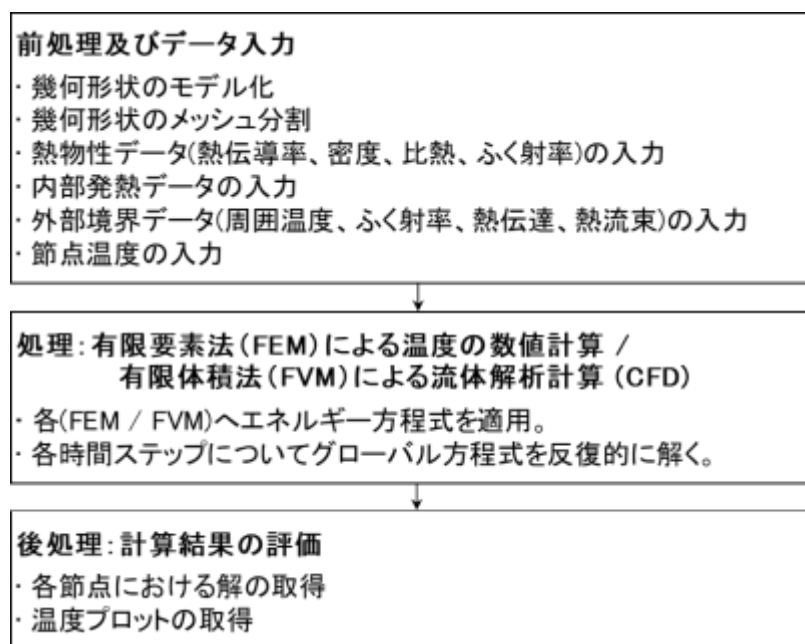
図 11 ANSYS®コードの解析フロー
