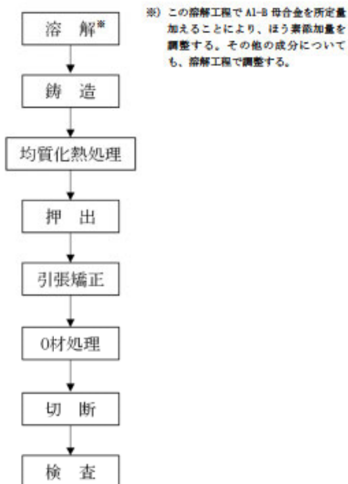
図 5-1 製造フロー
