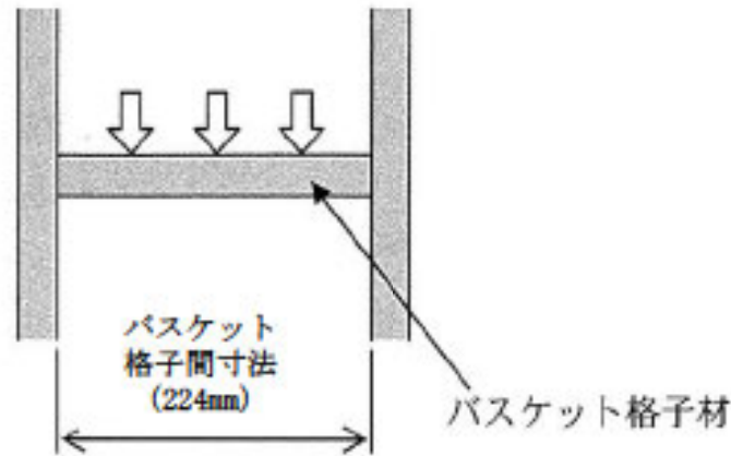
別紙 4-9 図 9m 水平落下事象でバスケットの強度評価に使用するモデル (両端固定・等分布荷重)
