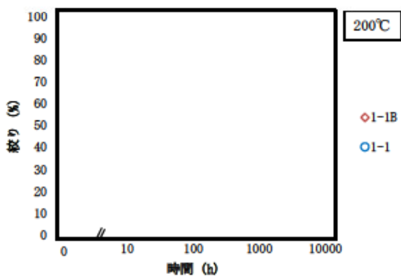
(p) 保持温度：200℃、絞り
