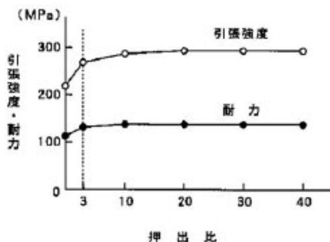
別紙 1-3 図 押出比が強度特性に及ぼす影響 (JIS A5056 基複合材) ①
