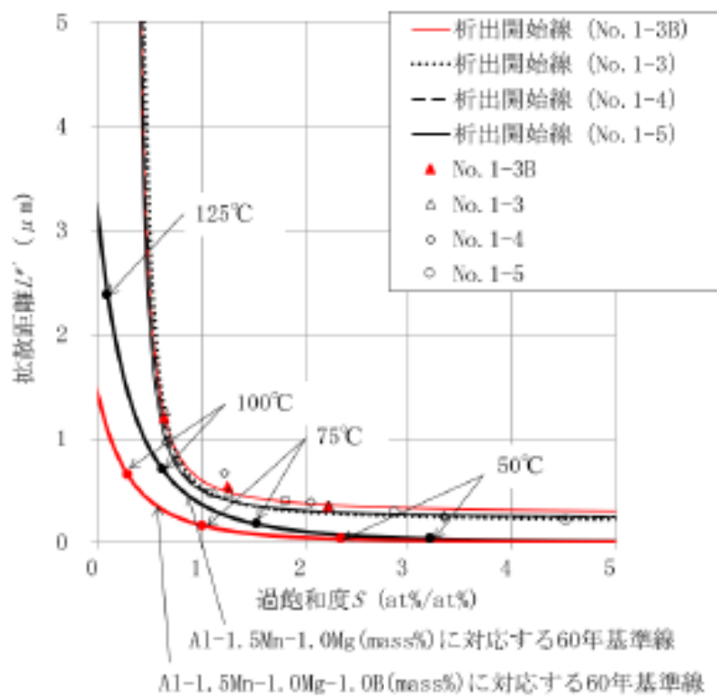
別紙 3-7 図 過飽和度と拡散距離による析出開始条件の評価 (SLP 線図)
