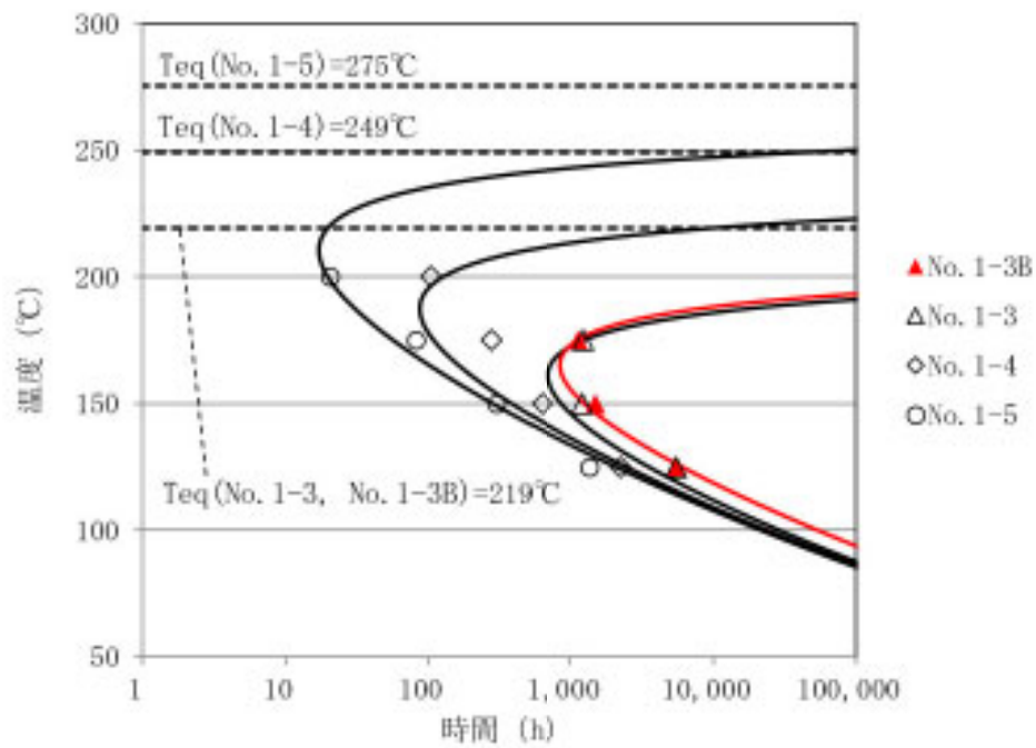
別紙 3-6 図 時効処理試験の結果から得られた TTP 線図
