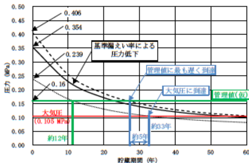
[貯蔵期間中の蓋間圧力の管理値設定例]
