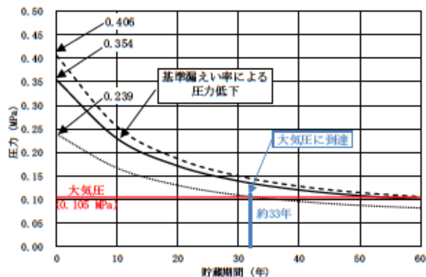
[金属ガasketの基準漏えい率による蓋間圧力の経時変化]
