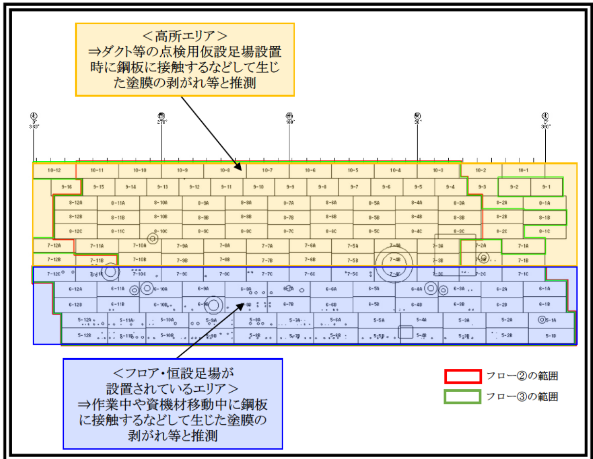
図 5. 3 軽微な劣化が確認された範囲（円筒部外面）
