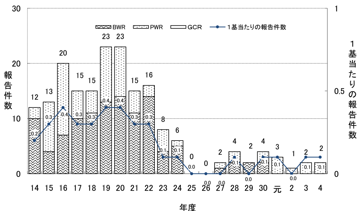
図 1-1 実用発電用原子炉(廃止措置中の原子炉及び特定原子力施設を除く)の報告件数 ※1 の推移
