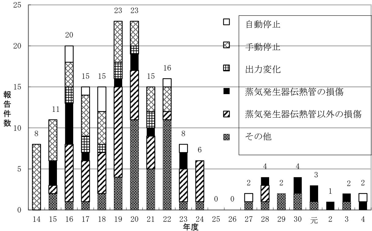
図 1-2 実用発電用原子炉(廃止措置中の原子炉及び特定原子力施設を除く)の報告件数 ※1 の事象別内訳の推移
