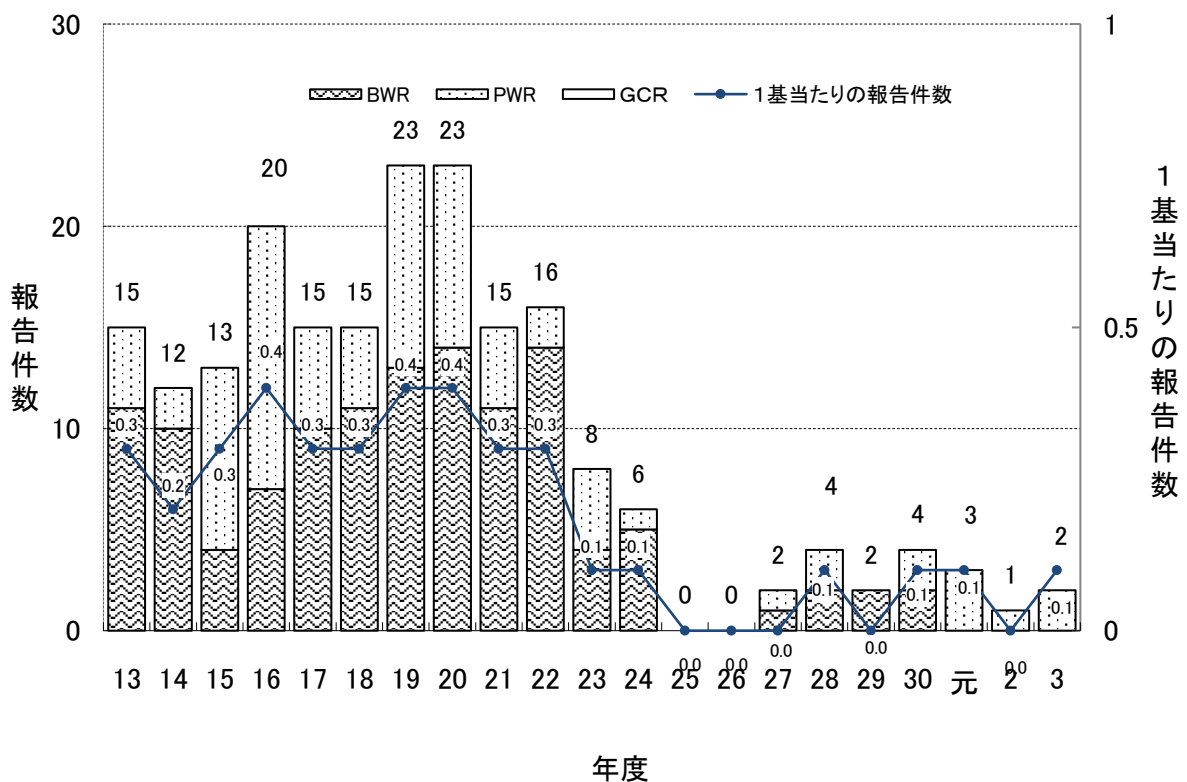
図 1-1 実用発電用原子炉(廃止措置中の原子炉及び特定原子力施設を除く)の報告件数 ※1 の推移
