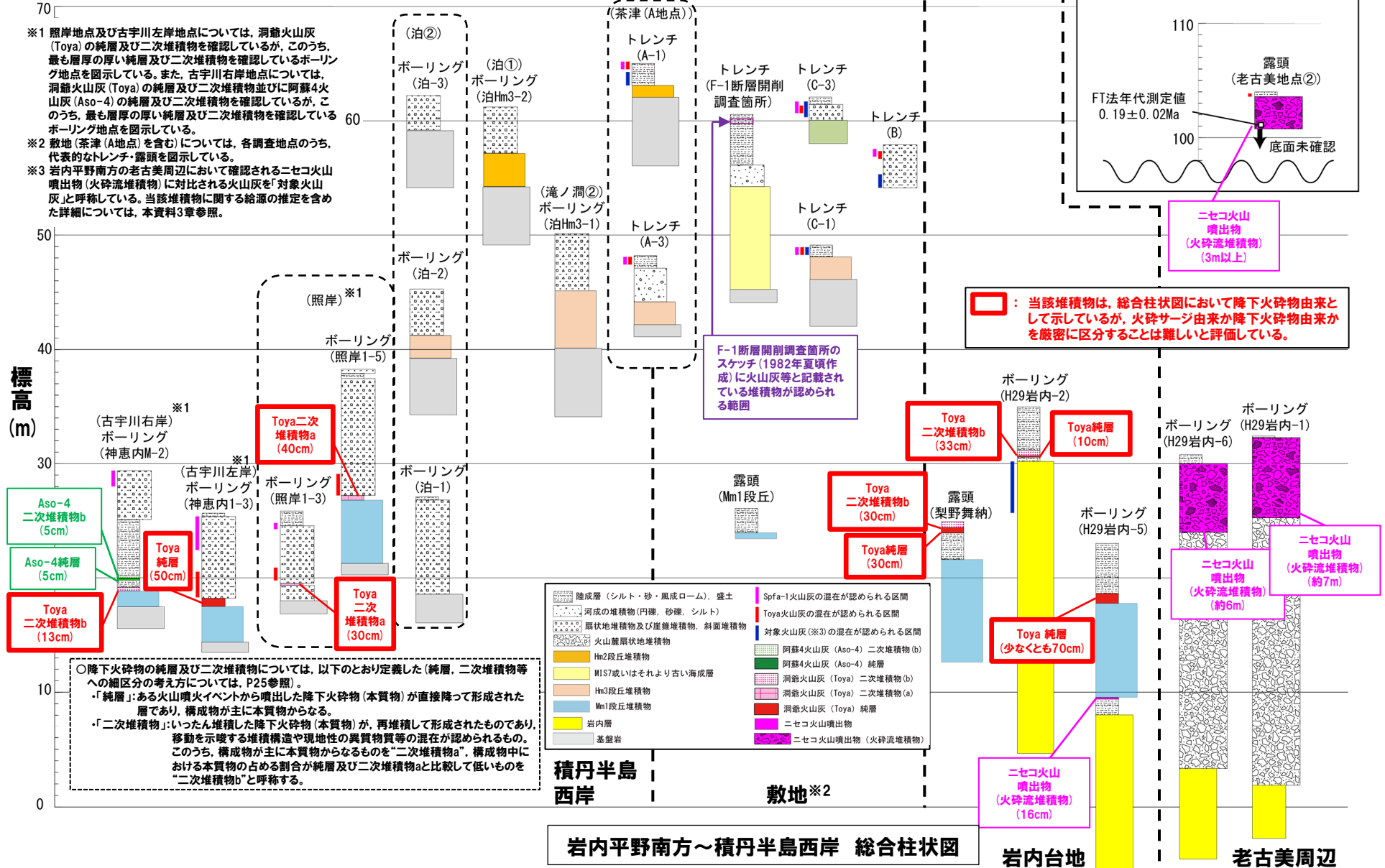
【総合柱状図】(2/2)
