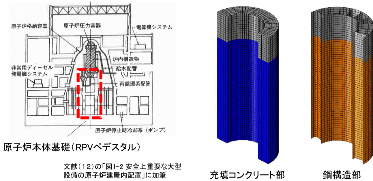
図1-6 原子炉本体基礎と解析モデル(1/2モデル)の一例
