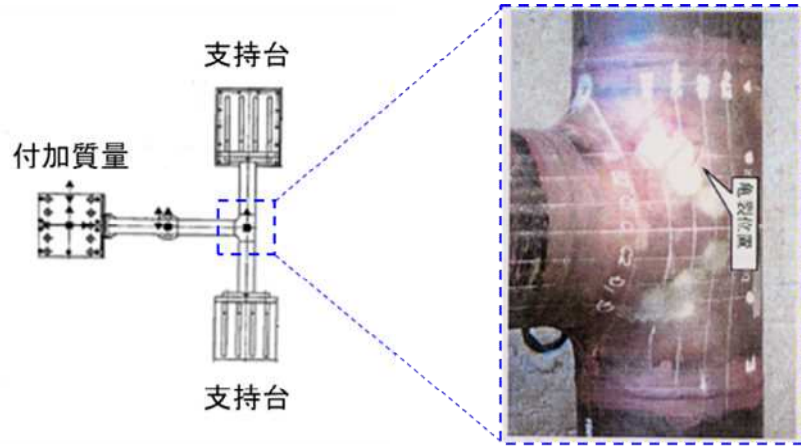
図1-5 配管要素の振動試験の一例
