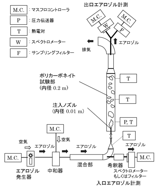
図3 中規模実験
