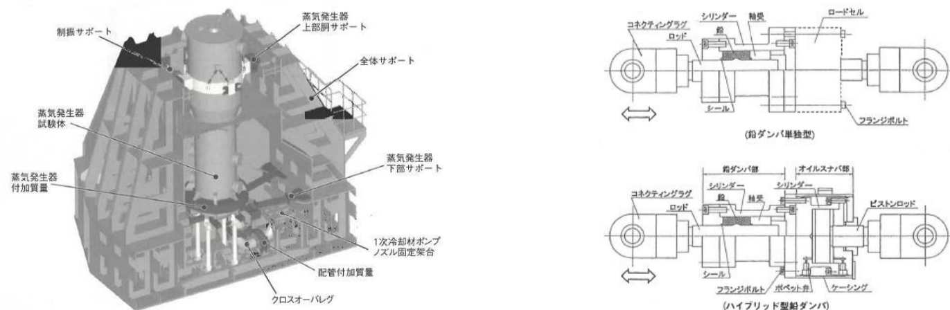
図1-7 過去に旧原子力発電技術機構で実施した制振装置(鉛ダンパ)の振動試験の例 (12) (左: 試験体の概要、右: 鉛ダンパの構造)
