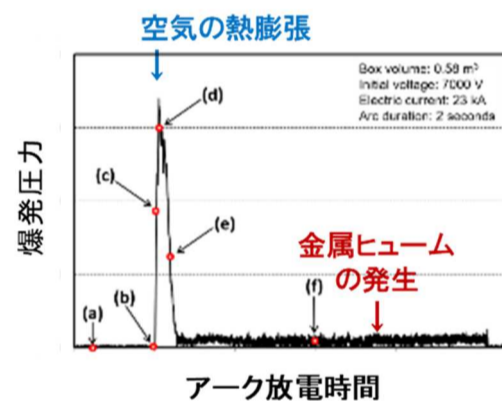
図1 筐体内における爆発圧力とアーク放電時間の関係
