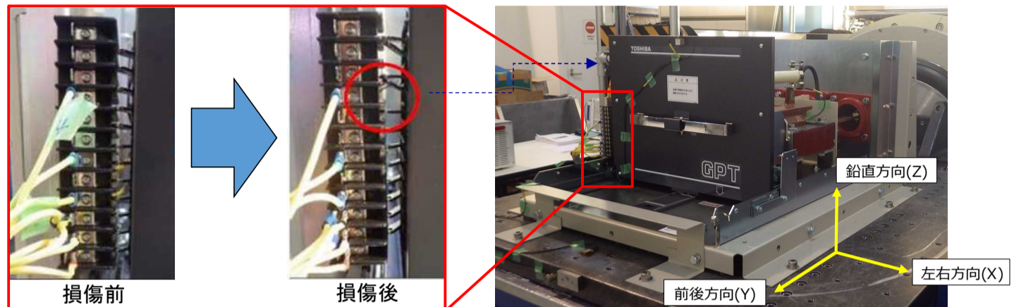
図3-3 ガタ系等を有する設備の衝撃振動試験とその損傷事例
