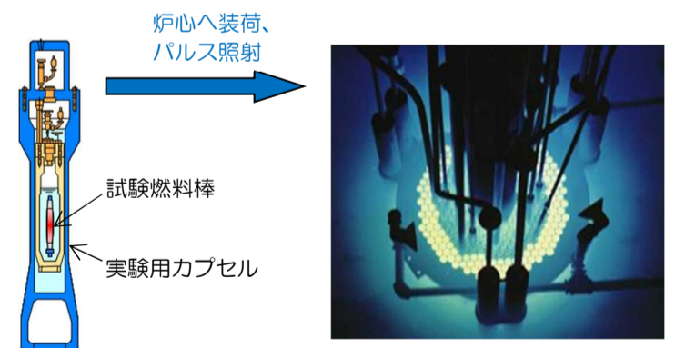
(a) 試験装置の概略図 (b) RIA 模擬試験用研究炉 (NSRR)
