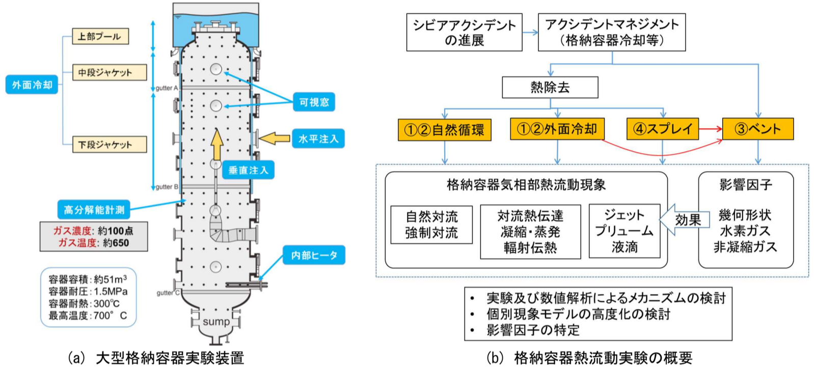
図6 大型格納容器模擬装置と実験の概要
