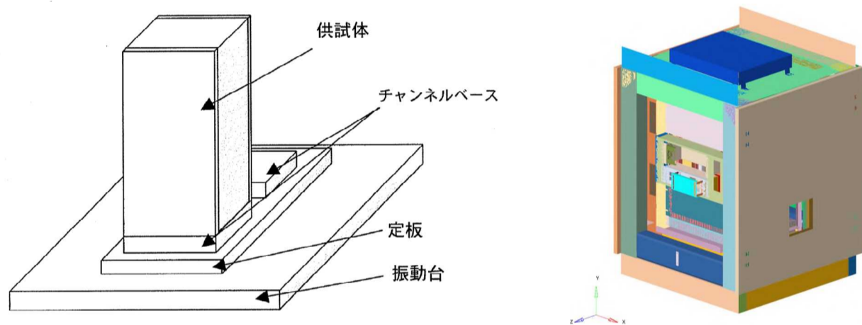
図3-4 衝撃振動試験のイメージと電気品の解析モデルの一例
