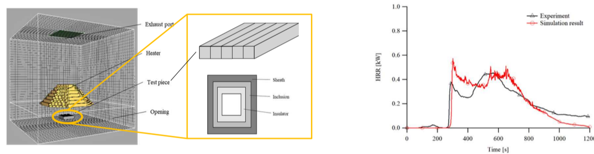
図 6 コーンカロリメータ試験の解析モデルの例
