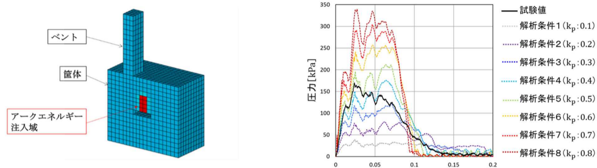
図 5 HEAF における爆発圧力の解析モデル例
