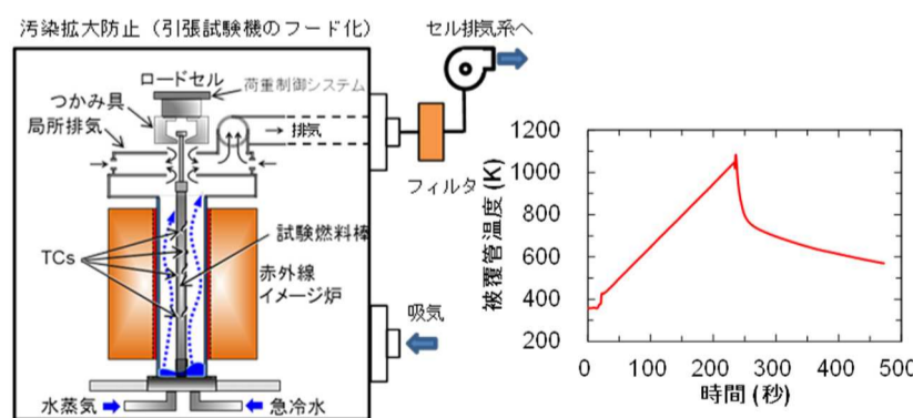
(a) 試験装置の概略図 (b) 試験時の温度履歴の例
