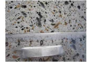
図1 模擬燃料デブリ (ドイツでの試験)
