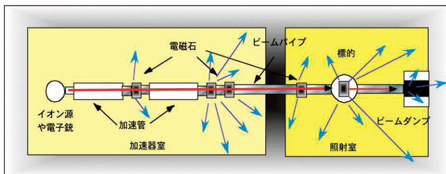
加速器の概念図
