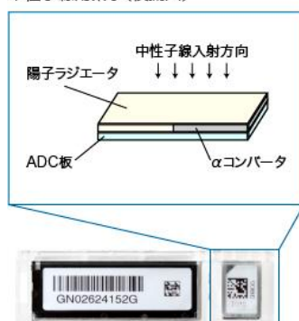
図 2.3 市販の CR-39 付線量計と CR-39 素子の構造
