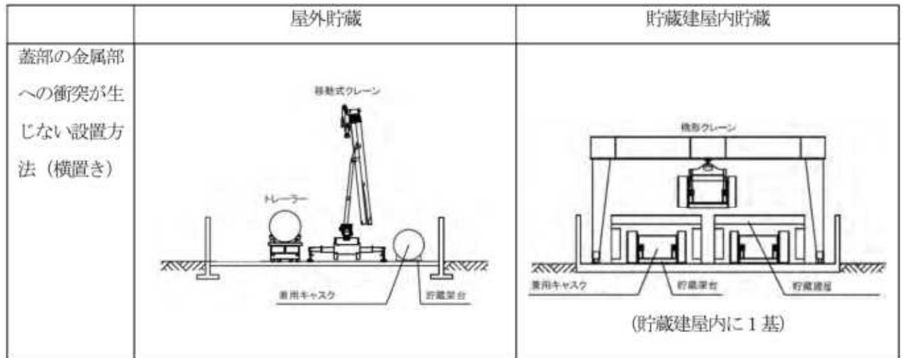
第12図 兼用キャスク貯蔵施設概要図（例）
