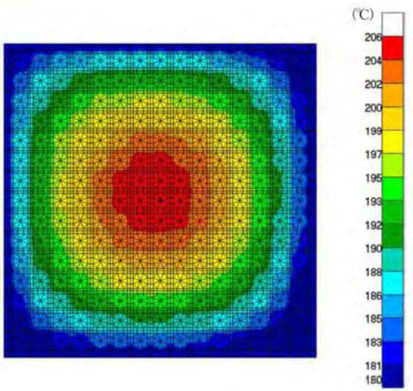
第 10 図 MSP-24P 型除熱解析結果(燃料集合体モデル)
