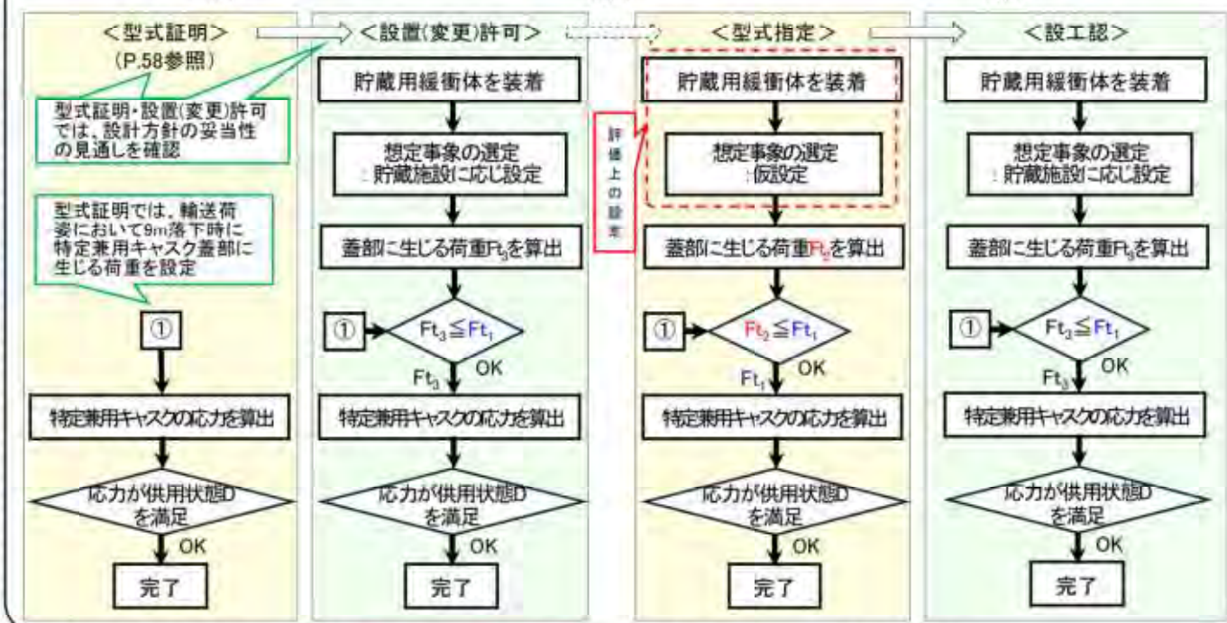
安全設計全般に係る設計方針の妥当性確認(安全評価)フロー (型式指定の前に設置(変更)許可が実施される場合)
