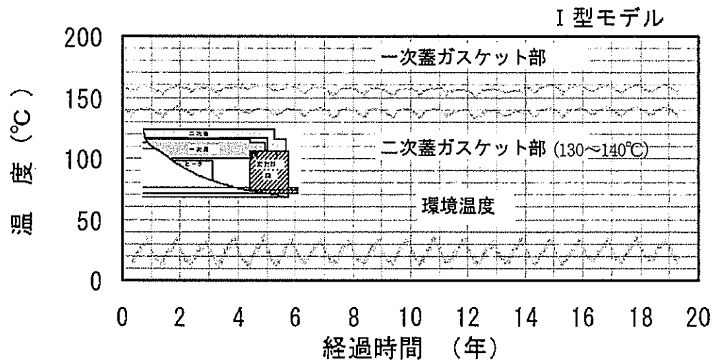
第7図 金属ガスケット (二次蓋) の長期密封性能試験結果 (眼鏡型) (3)
