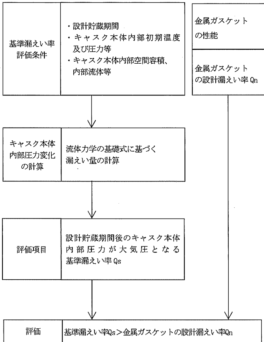
第4図 閉じ込め評価フロー
