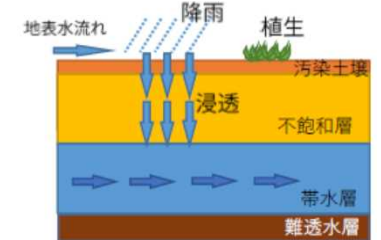
サイトの残存放射性物質 移行モデルの例
