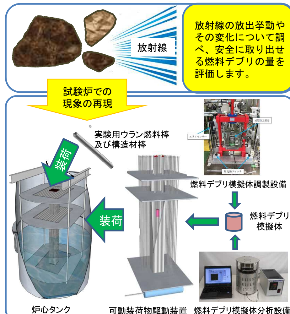
図1 試験炉における燃料デブリ模擬体を用いた実験の進め方例 （一部国立研究開発法人日本原子力研究開発機構の公開資料より抜粋）
