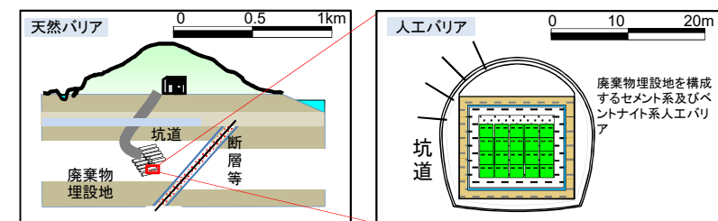
天然バリアの地質構造と配置
