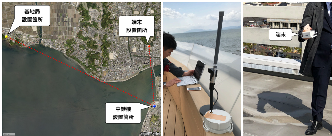
図 36 県庁との通信試験。(左) 基地局、中継機、端末の位置関係。端末と基地局の間は山と市街地のビル等で遮られた状態。(中) 県立美術館屋上に設置した中継機。(右) 県庁屋上に置いた。
