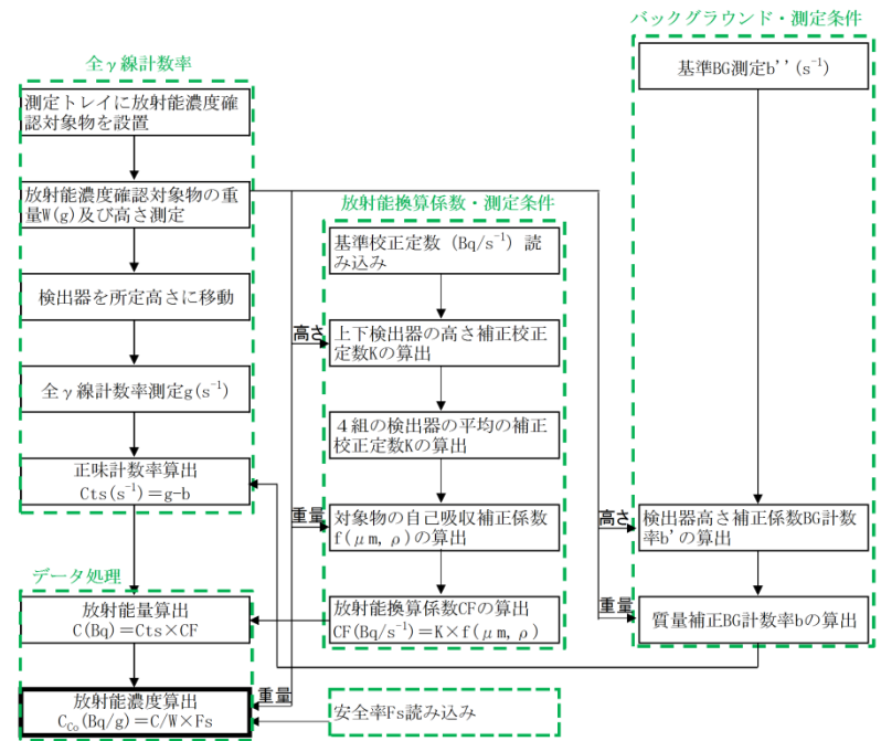
図 - 5 放射線測定法の処理フローと不確かさの要因の抽出
