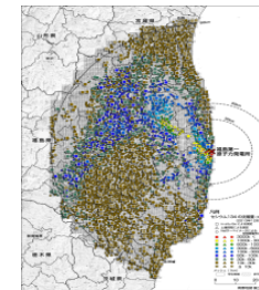
放射性セシウムの沈着量の変化傾向を数値化
