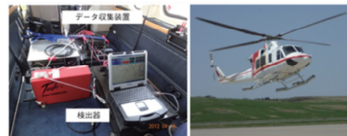
航空機モニタリング機器とヘリコプター
