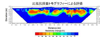
比抵抗探査トモグラフィーによる評価
