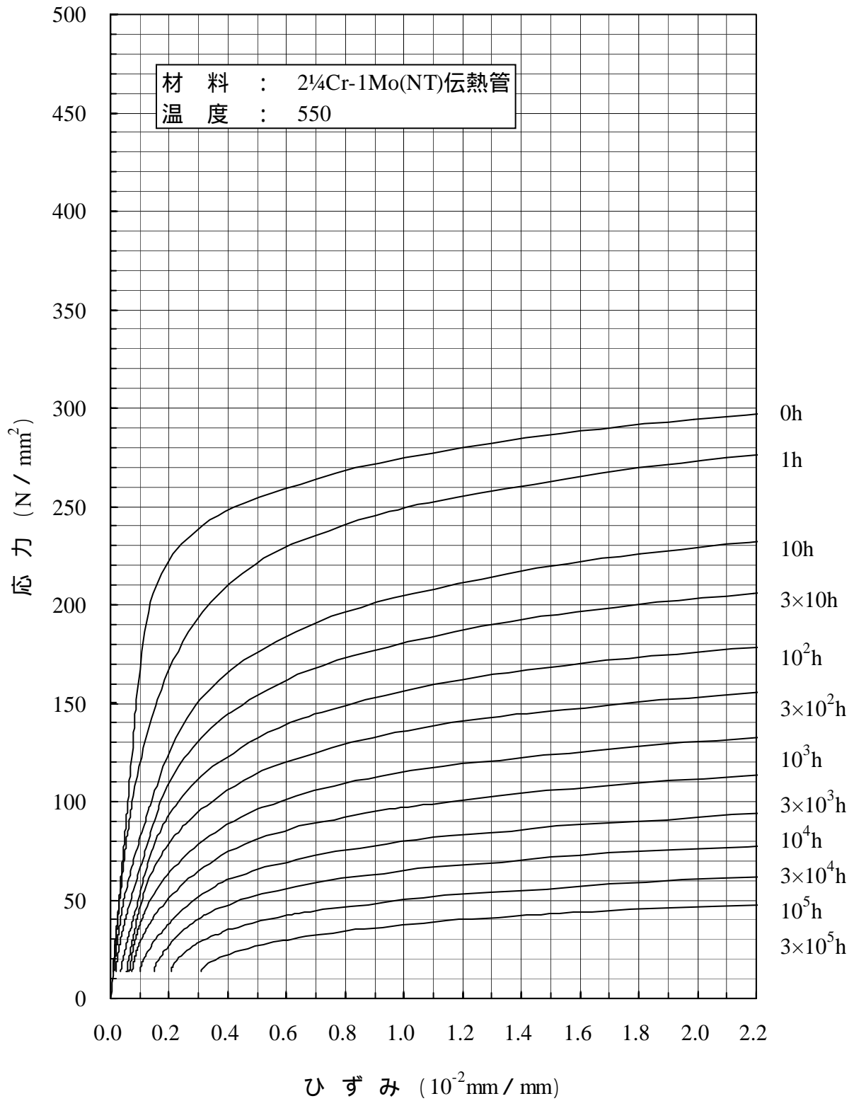
別図1.11-(e)(8) 2 \frac{1}{4} Cr-1Mo(NT)伝熱管の等時応力 - ひずみ線図
