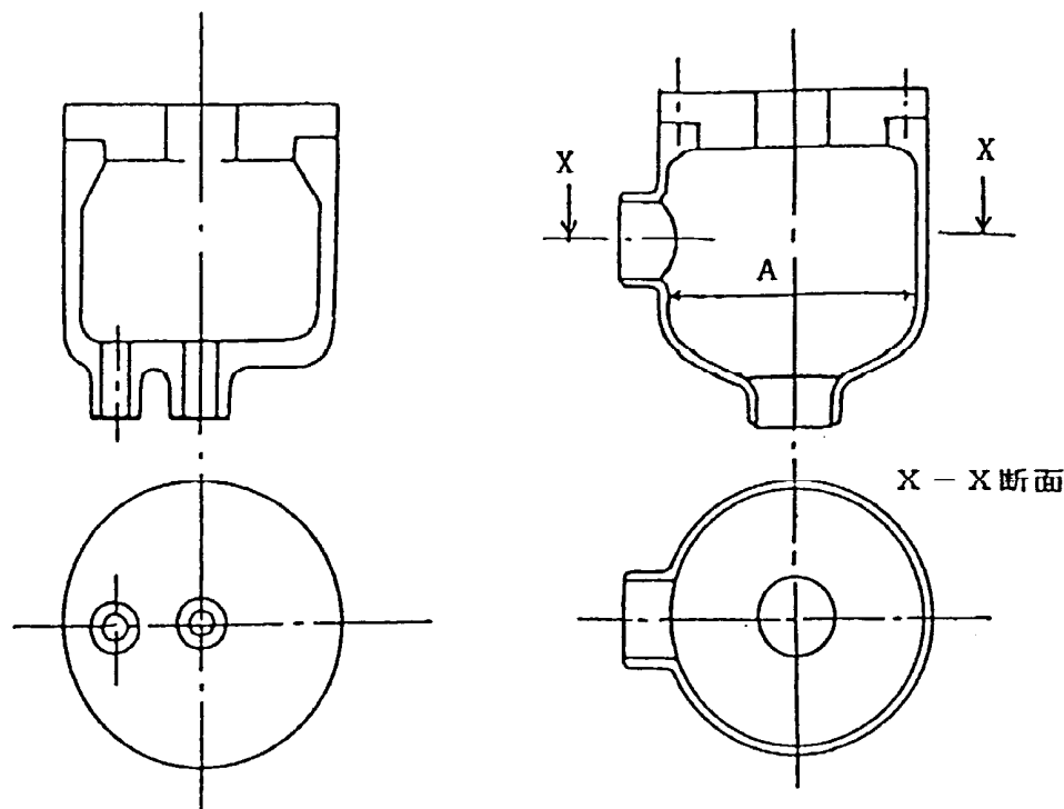
図5 ターボポンプであって、ケーシングが軸垂直割りで軸対称であるもの
