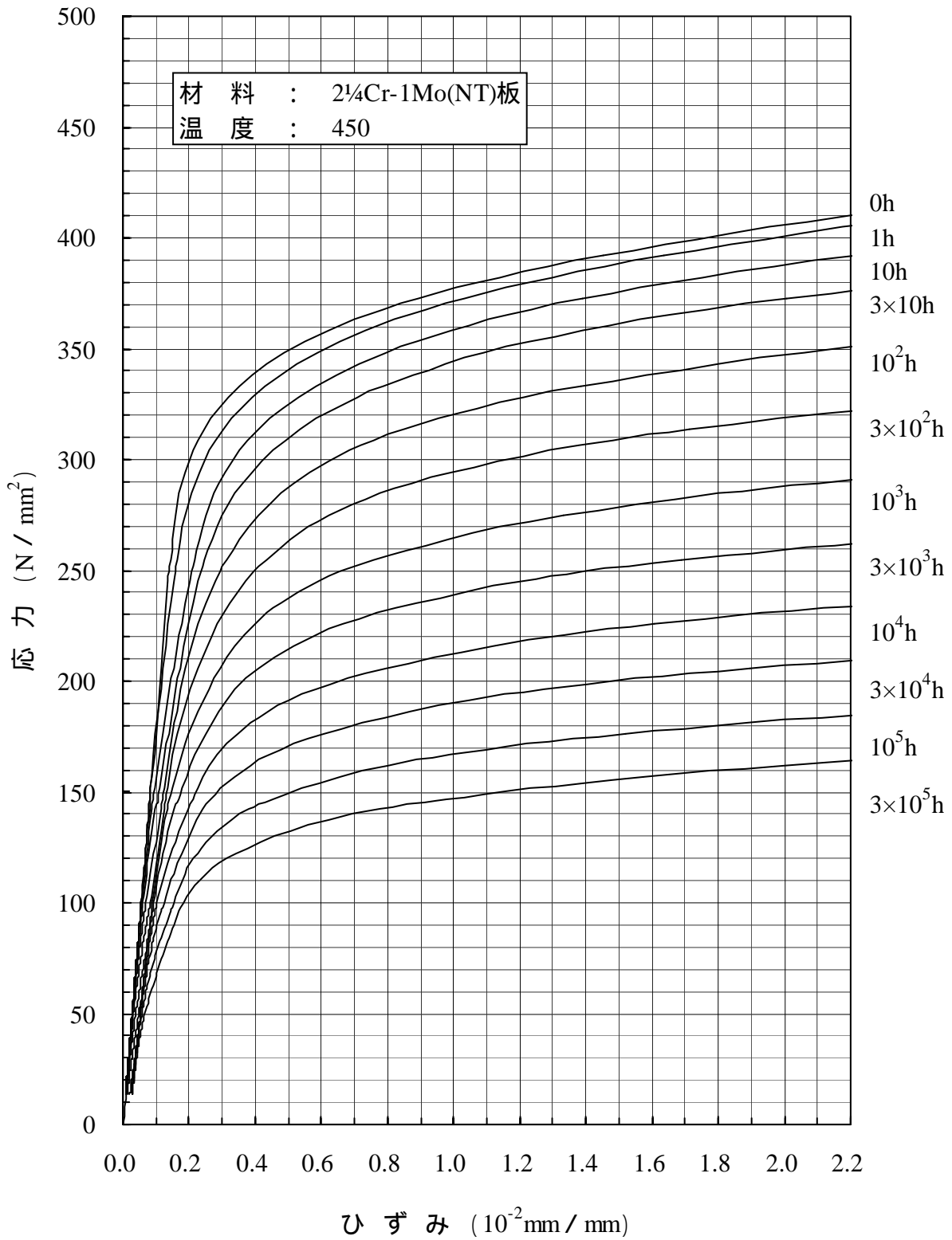
別図1.11-(d)(4) 2 \frac{1}{4} Cr-1Mo(NT)板の等時応力 - ひずみ線図
