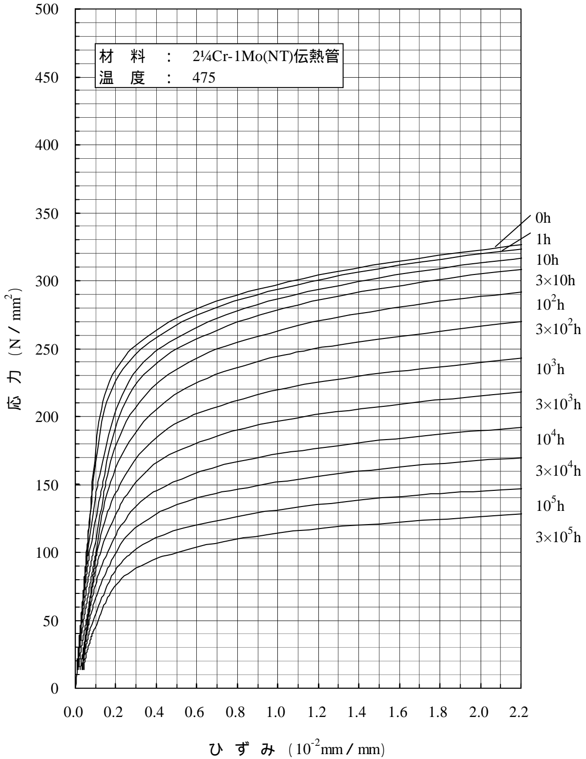
別図1.11-(e)(5) 2 \frac{1}{4} Cr-1Mo(NT)伝熱管の等時応力 - ひずみ線図
