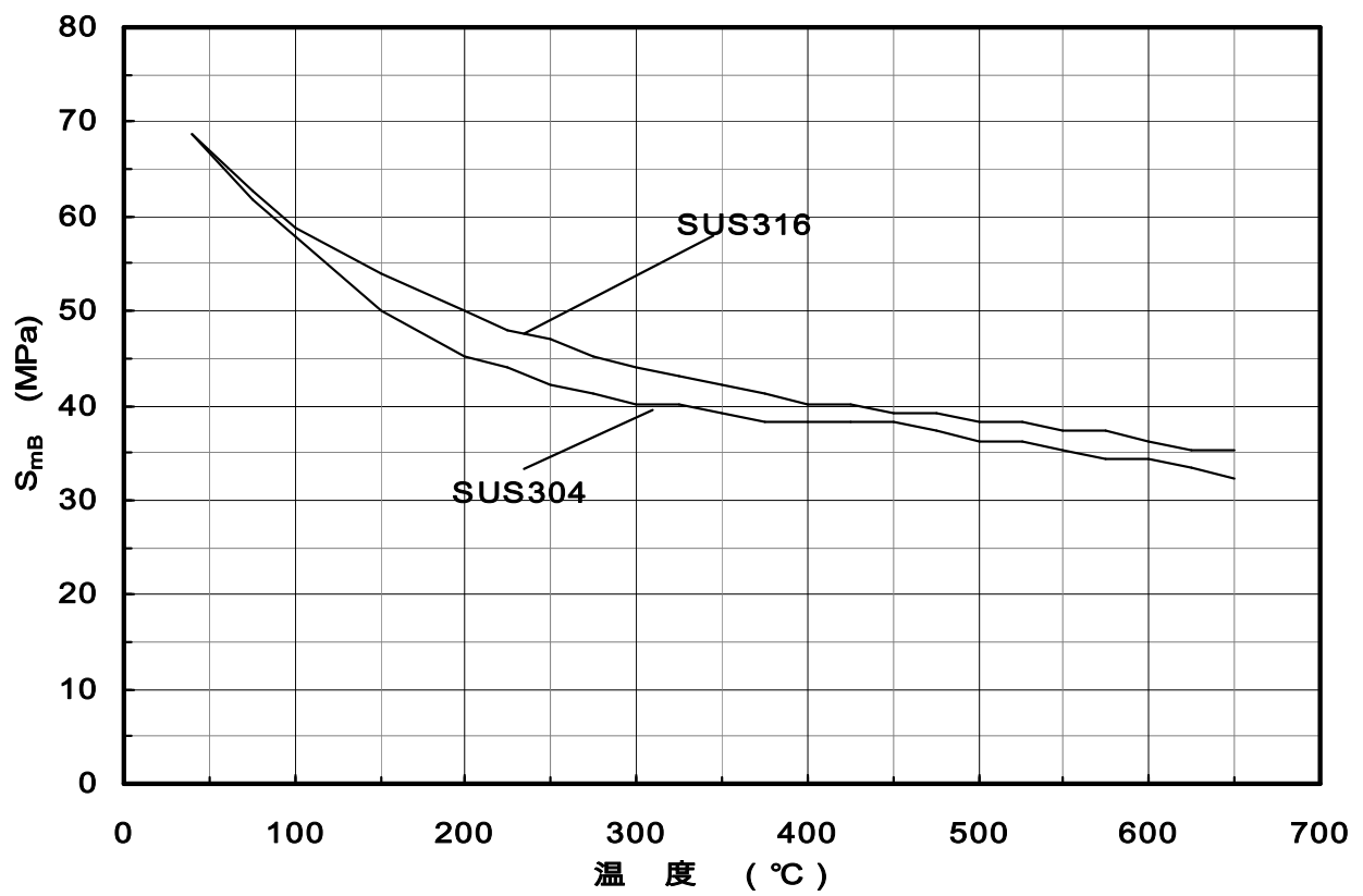
付図A.2 設計応力強さ S_{mB}
