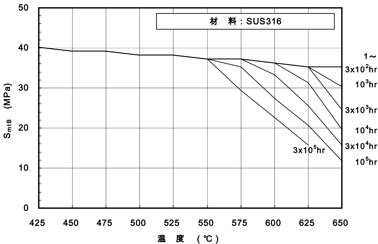
付図 A.3-(b) 計応力強さ S_{mtB} (SUS316)
