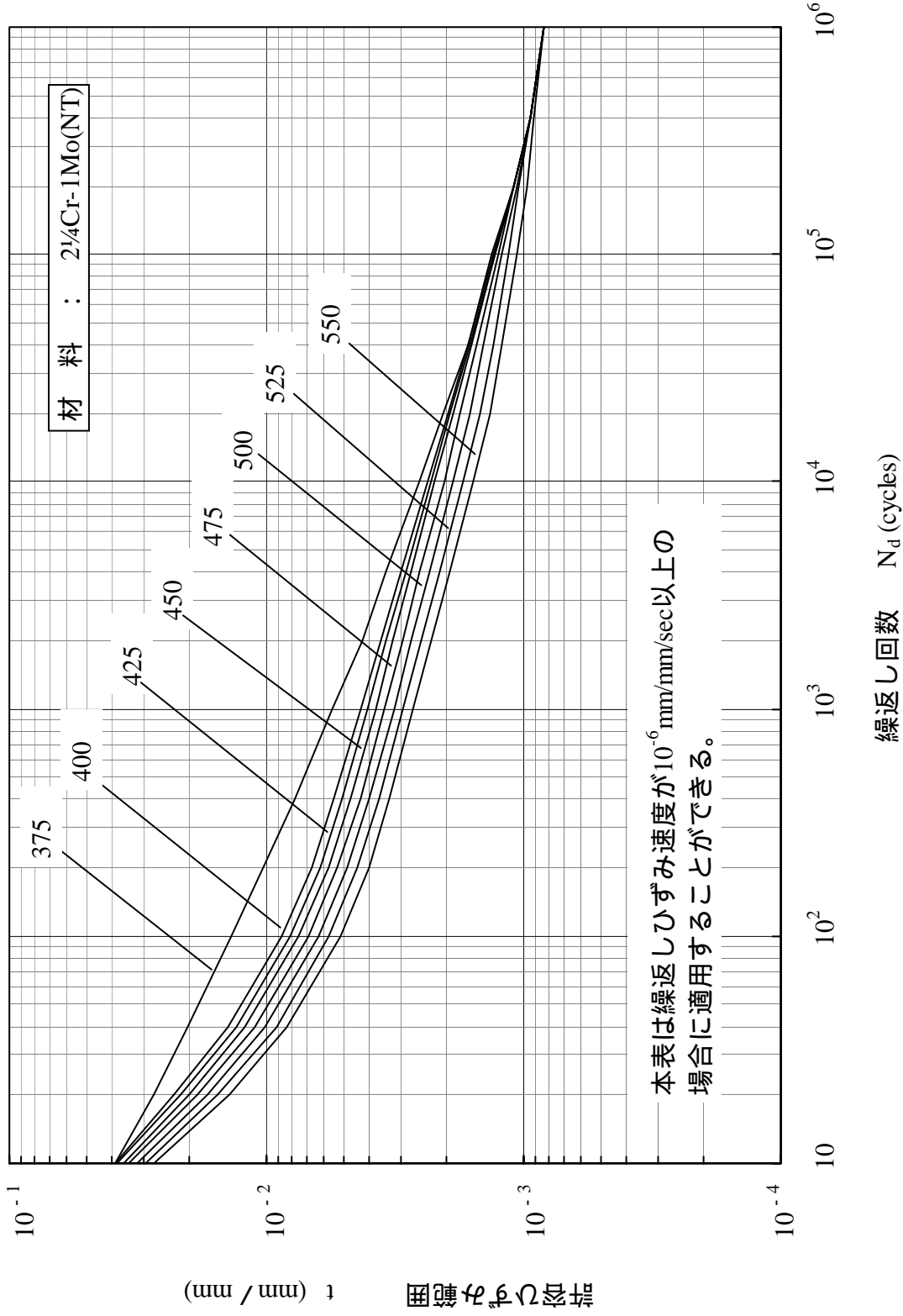
別図1.9-(d),(e) 2 1 / 4 Cr-1Mo(NT)の許容ひずみ範囲(B) \Delta\sigma (mm / mm)
