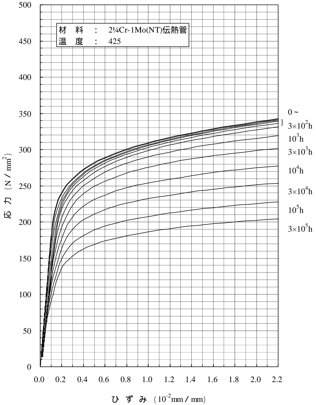
別図1.11-(e)(3) 2 1/4Cr-1Mo(NT)伝熱管の等時応力 - ひずみ線図
