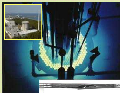
反応度事故模擬試験
