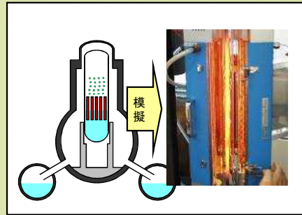
冷却材喪失事故模擬試験
