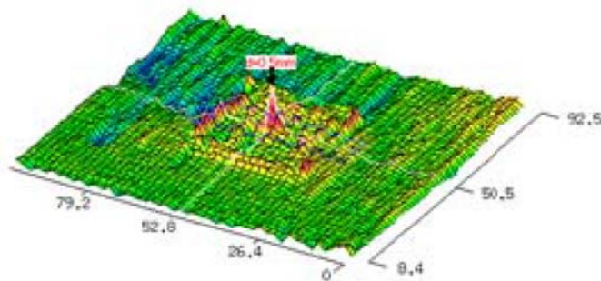
図 3.2.4.3 MAG 型プローブによる波形例
