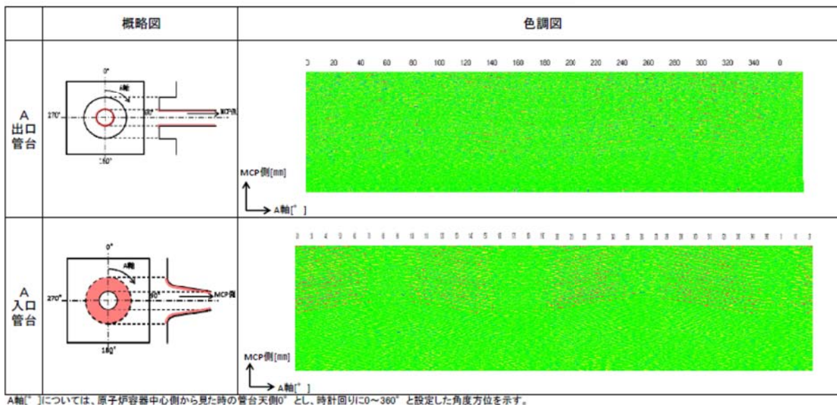
図 4.2.1 ノズルコーナー部 ECT 色調図（例）
