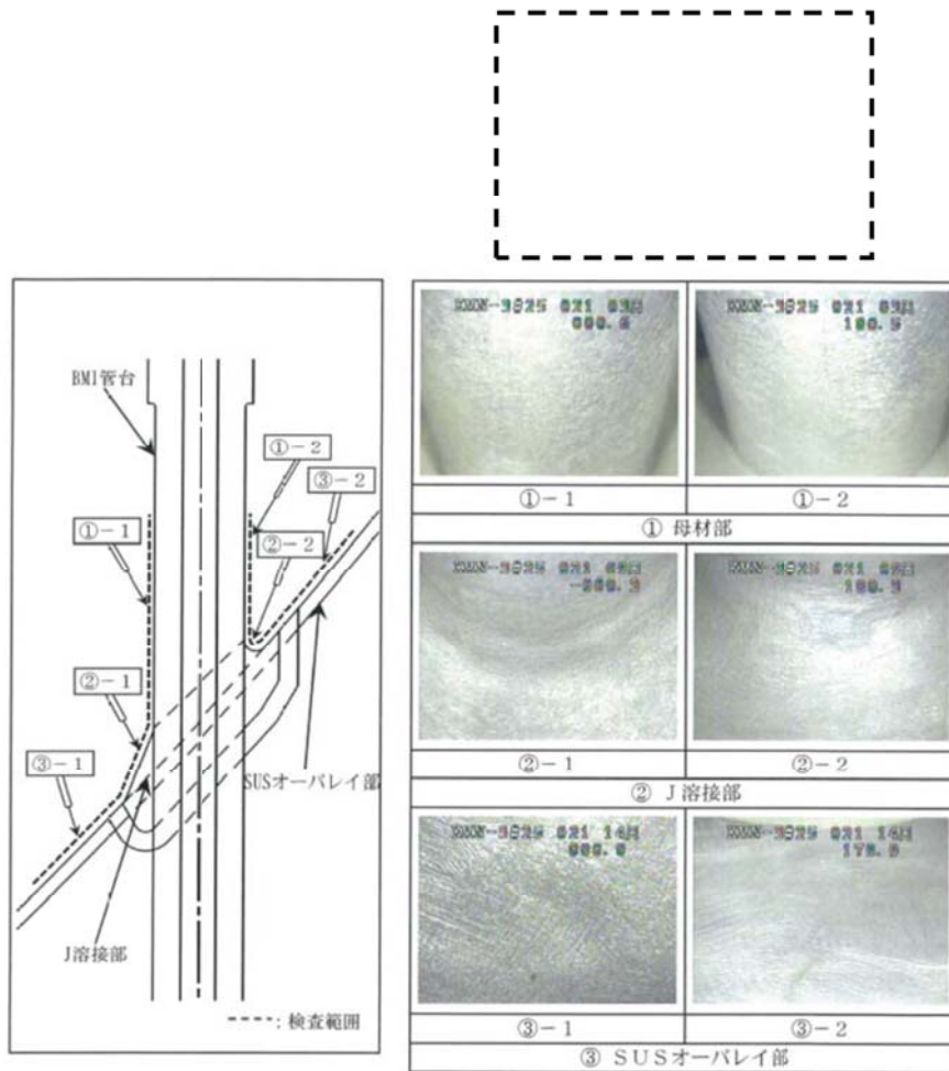
図 4.3.2 1 ミルワイヤ及び MVT-1 BMI 画像 (例)
