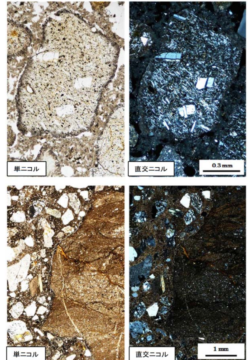
偏光顕微鏡観察結果
