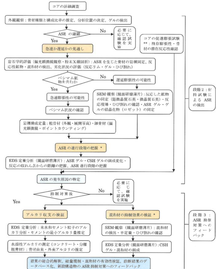
コンクリート建造物のASR診断フロー(案)
