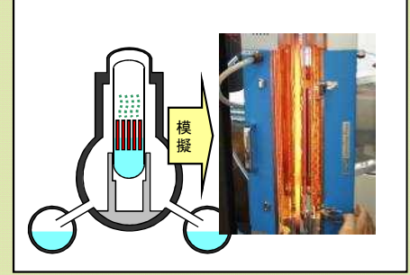
冷却材喪失事故模擬試験
