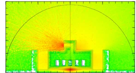
使用済燃料貯蔵施設の敷地境界線量解析の例
