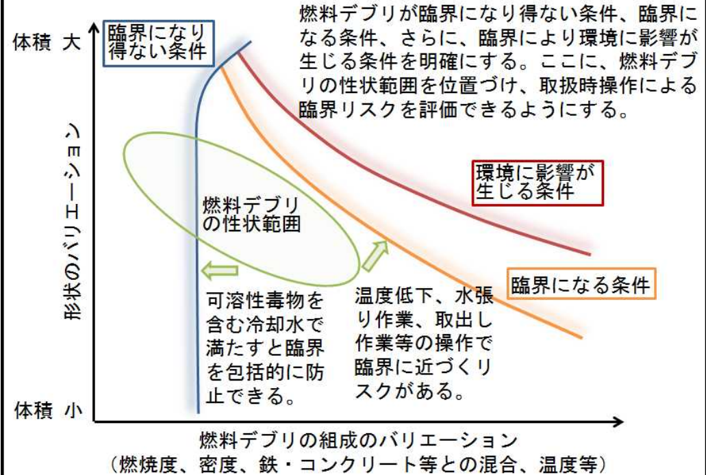
図1 燃料デブリの臨界リスク評価
