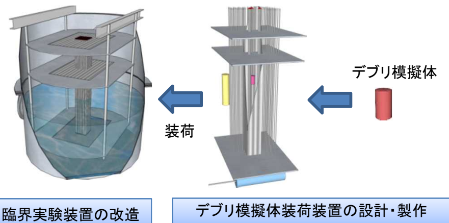
図2 臨界実験装置及び燃料デブリ模擬臨界実験
