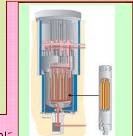
試験研究炉 照射容器 照射成長試験
