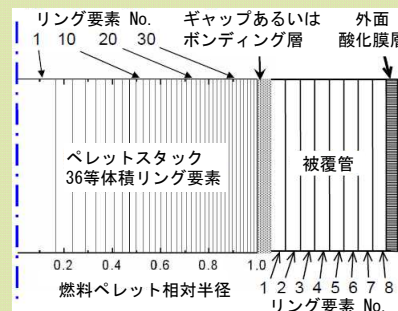
解析要素体系 反応度事故模擬試験解析
