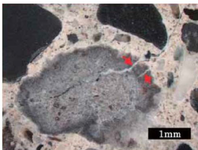
図3. 2. 4-1 実体顕微鏡観察での膨張ひび割れの確認事例 5)
