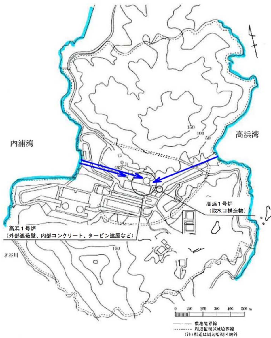
図一別紙7-1 高浜発電所 海岸線からの位置関係
