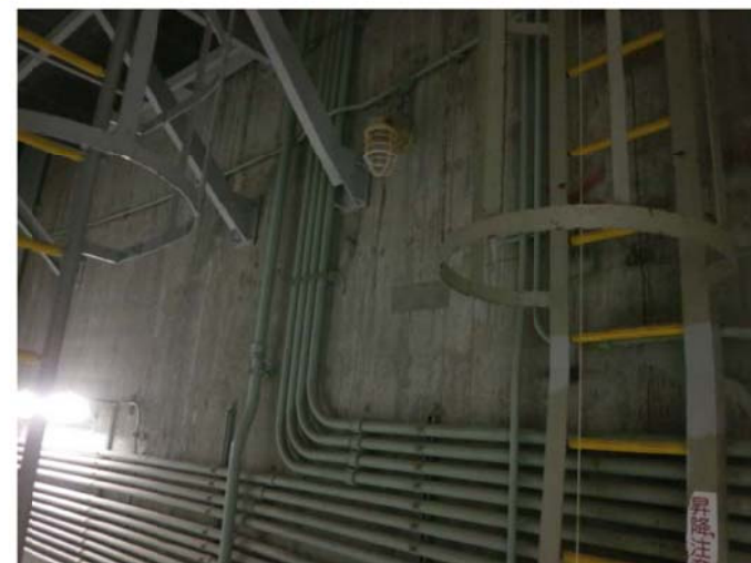
原子炉格納施設等 外部遮蔽壁(2号炉)
