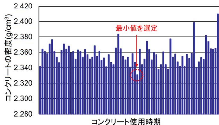
計算上のコンクリート密度(外部遮蔽壁)
