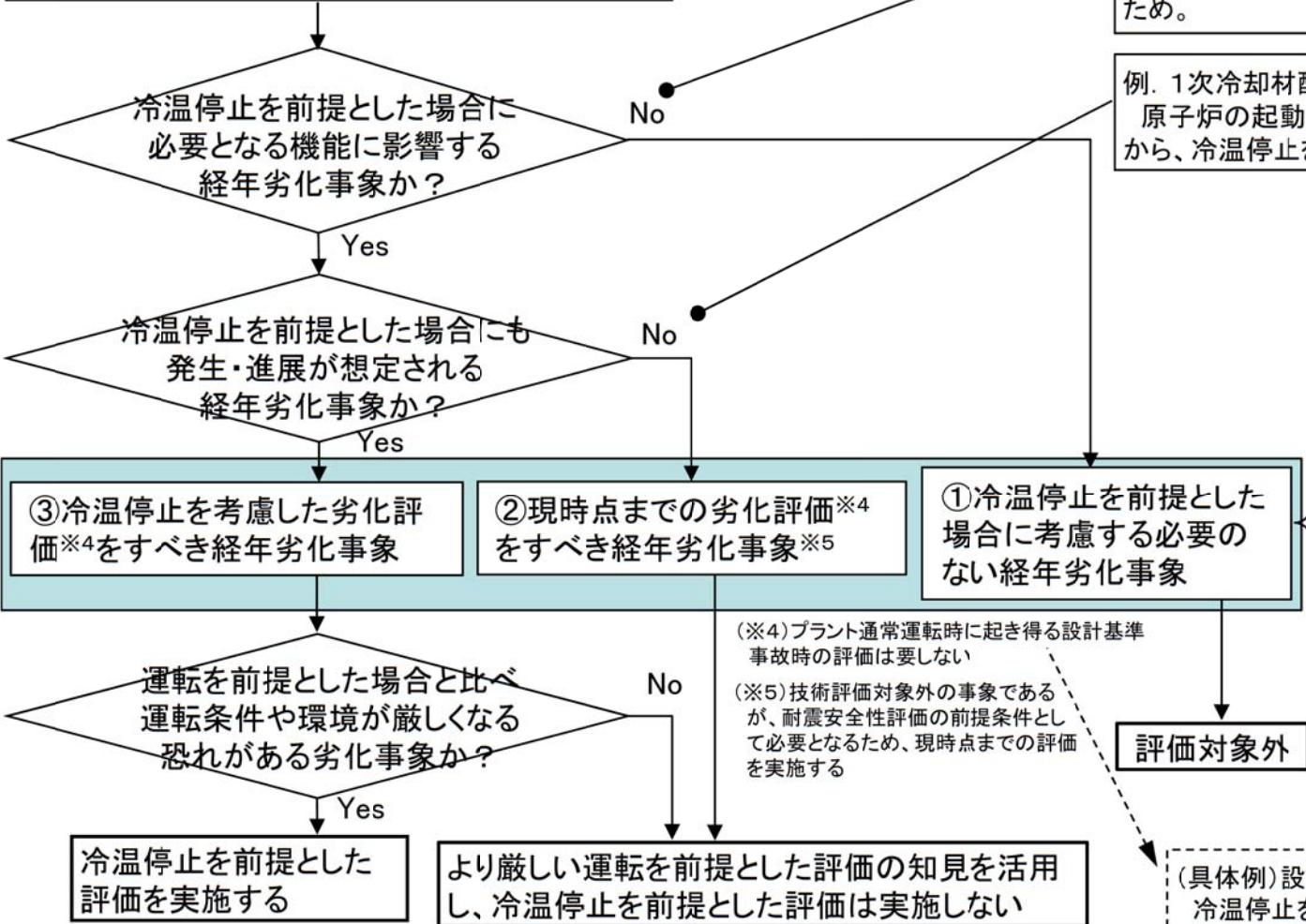
冷温停止を前提とした経年劣化事象の抽出フロー
