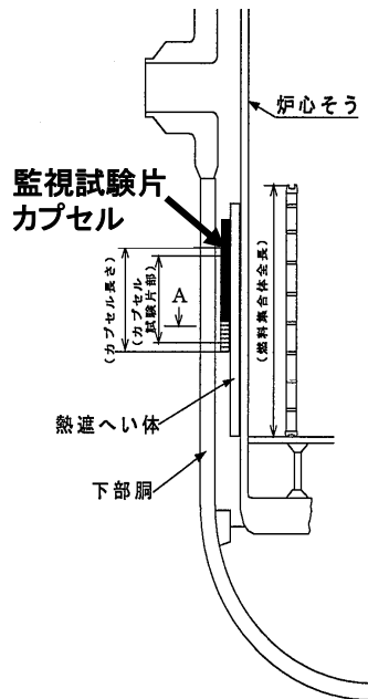
監視試験片の装荷位置
