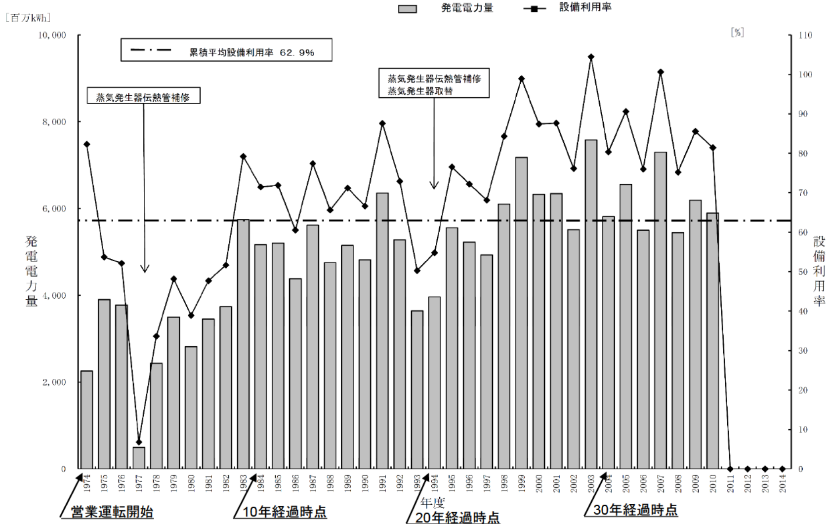
高浜発電所1号炉 発電電力量・設備利用率の年度推移
