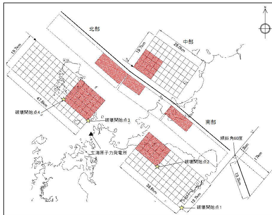
震源モデル
