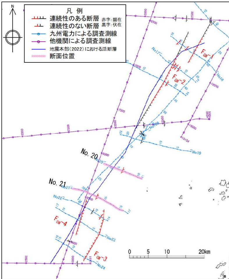
断層分布図
