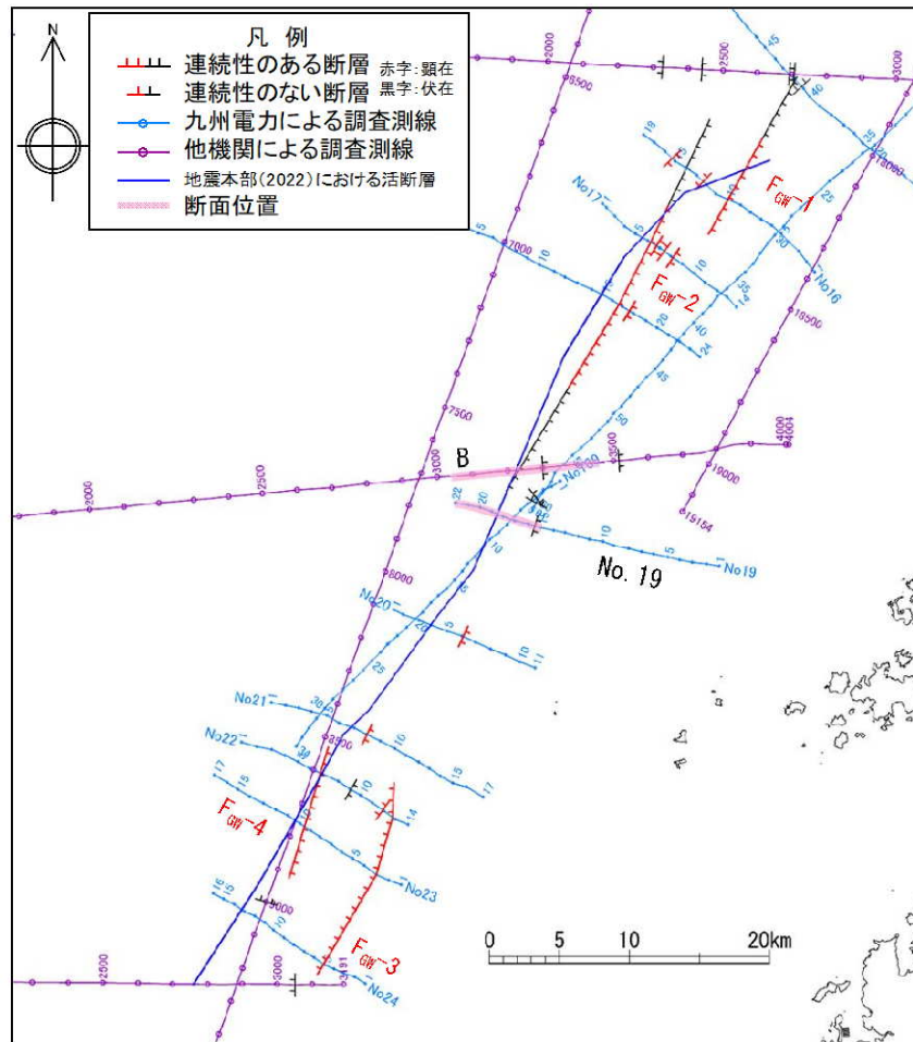
断層分布図
