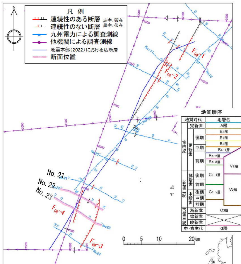
断層分布図
