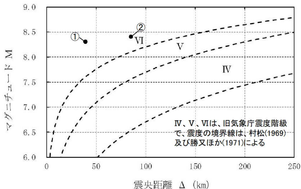
M- \Delta 図
