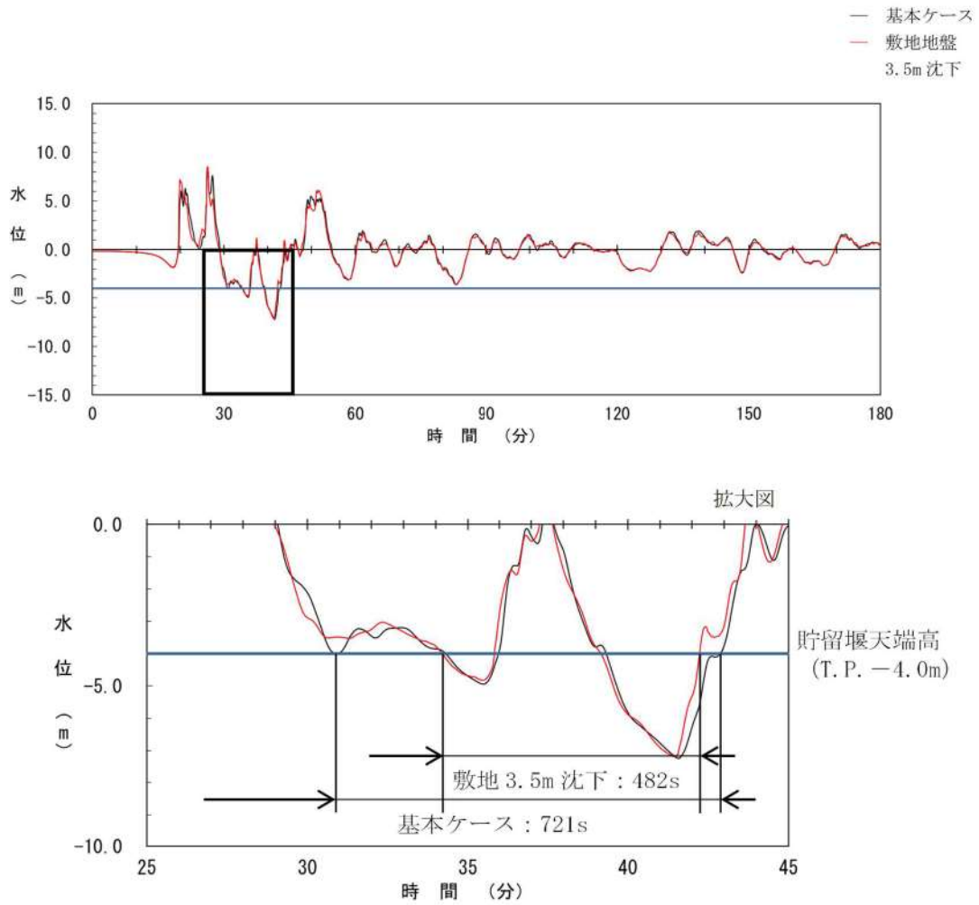
図 2.1.c.b-22 (31) 敷地（陸域）の地盤変状（3.5m 沈下）の有無による貯留堰を下回る時間の比較（基準津波（波源 I，防波堤損傷なし））
