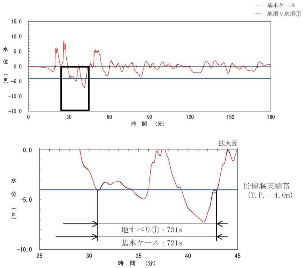
図 2. 1. b. c-1 (31) 地滑り地形①の斜面崩壊の有無による貯留堰を下回る時間の比較 (基準津波 (波源 I, 防波堤損傷なし))
