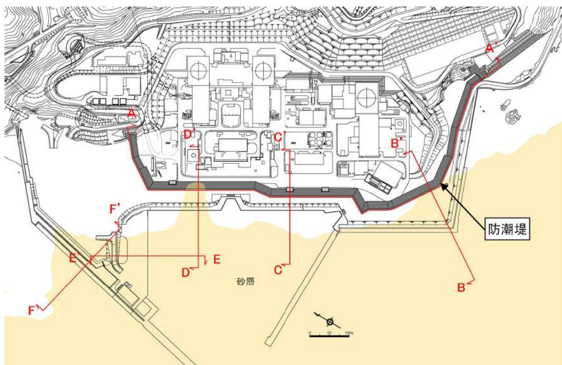
図 2.1.c.b-8 敷地平面図
