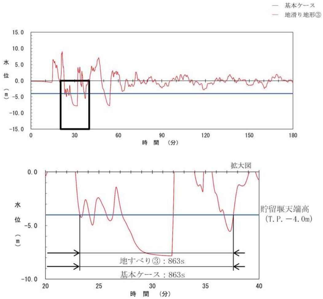
図 2. 1. b. c-2 (40) 地滑り地形③の斜面崩壊の有無による貯留堰を下回る時間の比較 (基準津波 (波源 L, 北防波堤損傷))
