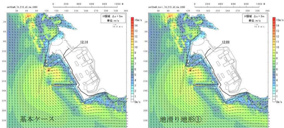
図 2. 1. b. c-1 (58) 地滑り地形①の斜面崩壊の有無による最大流速分布の比較 (基準津波 (波源L, 北防波堤損傷))
