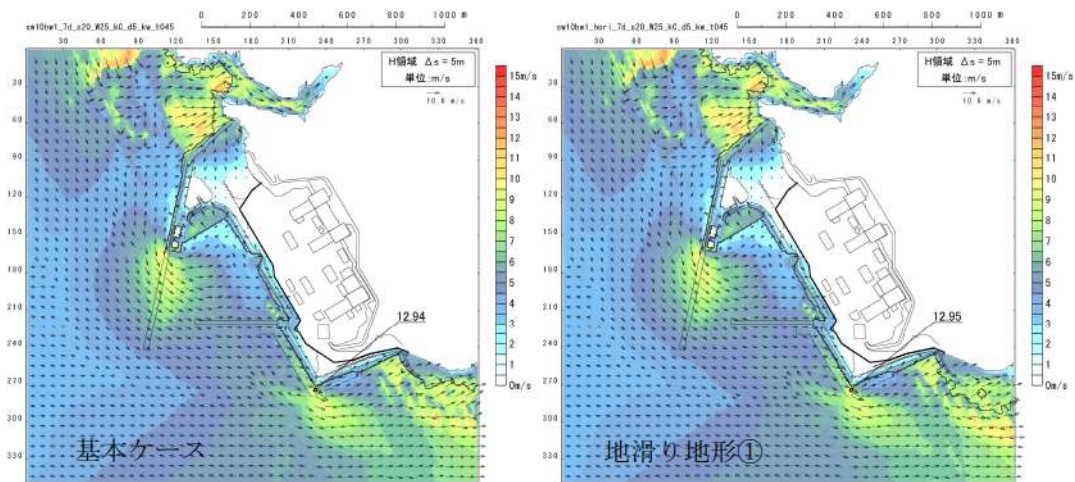
図 2.1.b.c-1 (56) 地滑り地形①の斜面崩壊の有無による最大流速分布の比較 (基準津波 (波源 J, 北及び南防波堤損傷))
