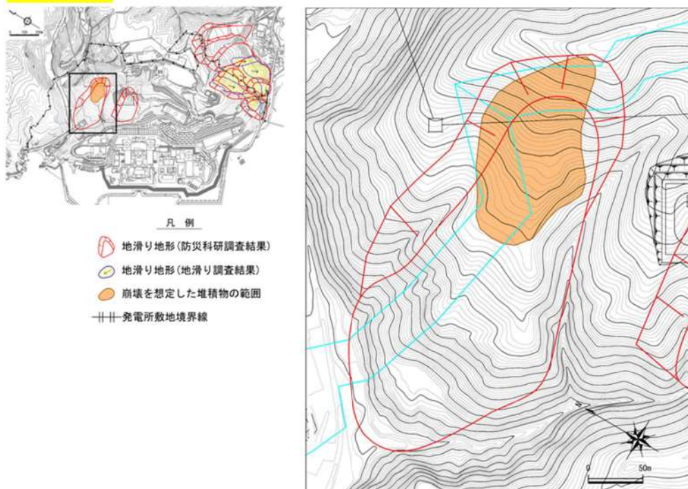
図 2.1.b.a-5 地滑り地形③分布図
