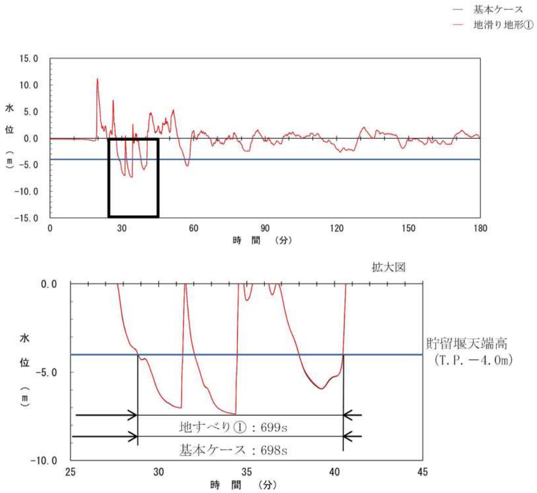
図 2. 1. b. c-1 (34) 地滑り地形①の斜面崩壊の有無による貯留堰を下回る時間の比較 (基準津波 (波源 J, 北及び南防波堤損傷))
