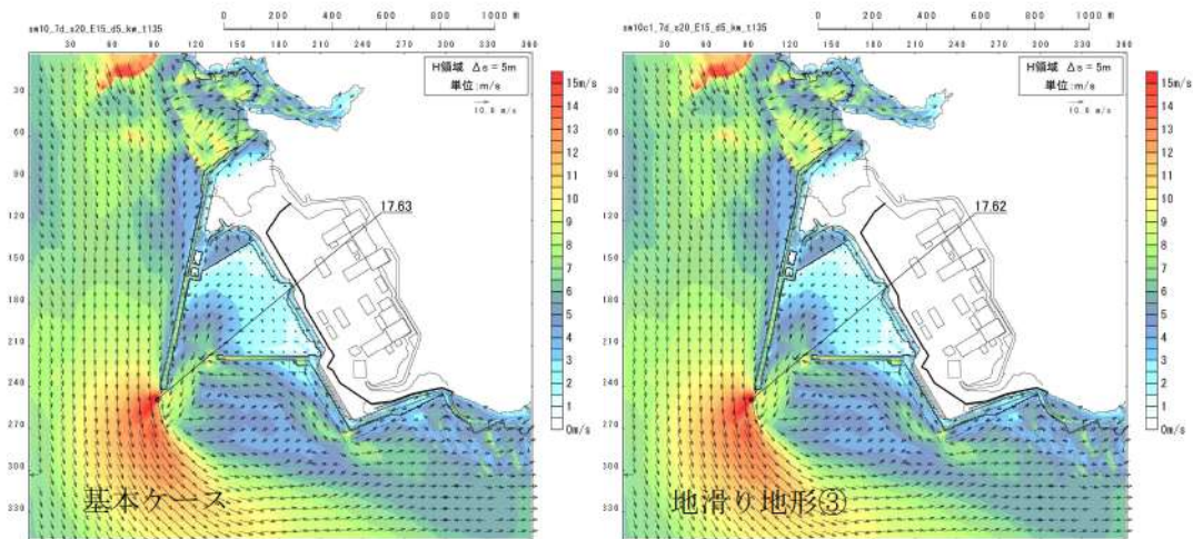
図 2. 1. b. c-2 (59) 地滑り地形③の斜面崩壊の有無による最大流速分布の比較 (最大流速波源 (波源K, 防波堤損傷なし))
