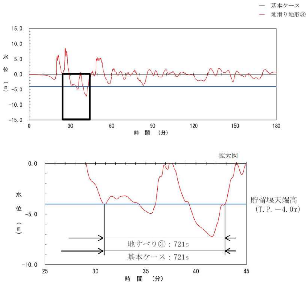
図 2. 1. b. c-2 (31) 地滑り地形③の斜面崩壊の有無による貯留堰を下回る時間の比較 (基準津波 (波源 I, 防波堤損傷なし))
