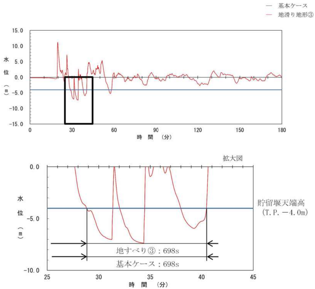
図 2. 1. b. c-2 (34) 地滑り地形③の斜面崩壊の有無による貯留堰を下回る時間の比較 (基準津波 (波源 J, 北及び南防波堤損傷))
