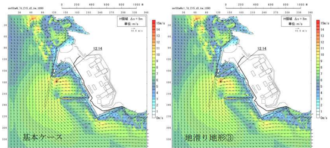
図 2. 1. b. c-2 (58) 地滑り地形③の斜面崩壊の有無による最大流速分布の比較 (基準津波 (波源 L, 北防波堤損傷))
