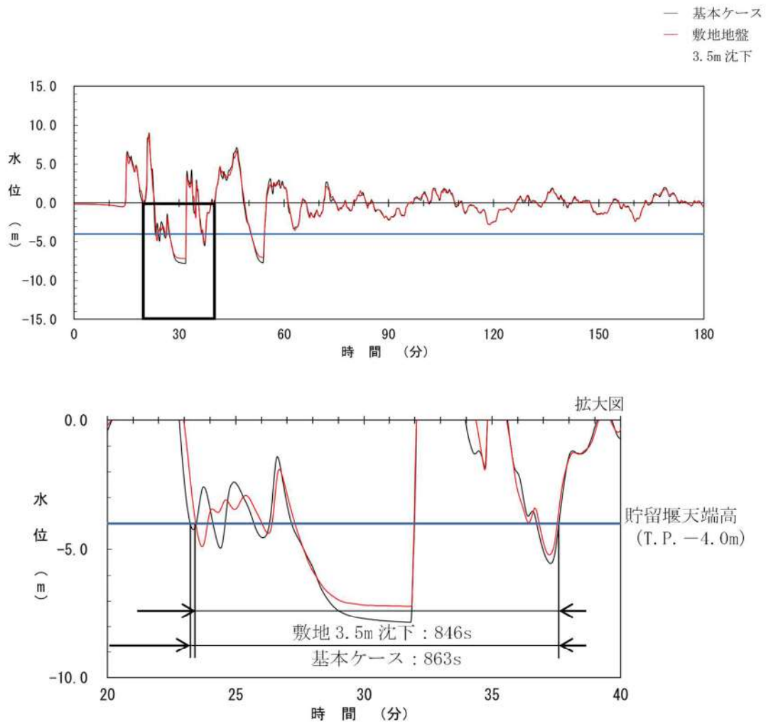
図 2.1.c.b-22 (40) 敷地（陸域）の地盤変状（3.5m 沈下）の有無による貯留堰を下回る時間の比較（基準津波（波源 L，北防波堤損傷））
