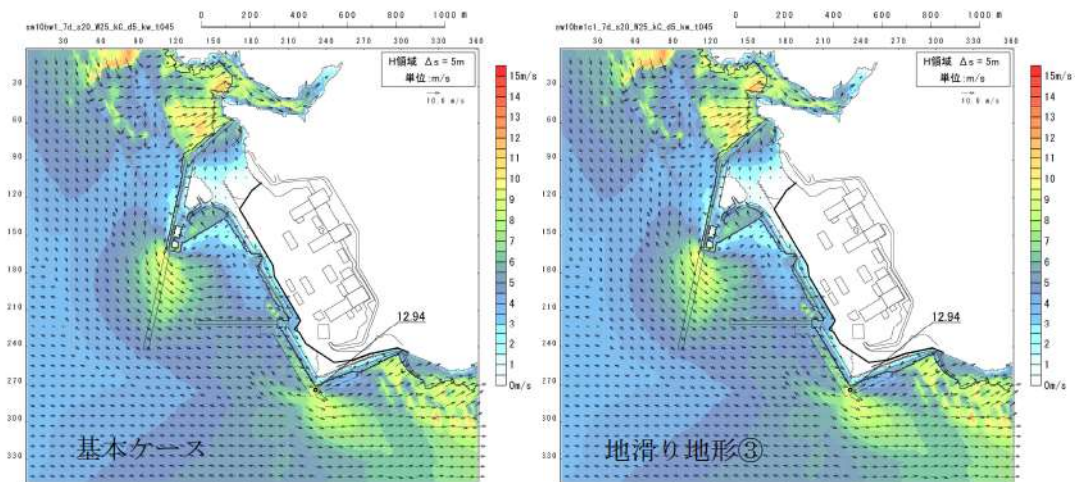
図 2. 1. b. c-2 (56) 地滑り地形③の斜面崩壊の有無による最大流速分布の比較 (基準津波 (波源 J, 北及び南防波堤損傷))
