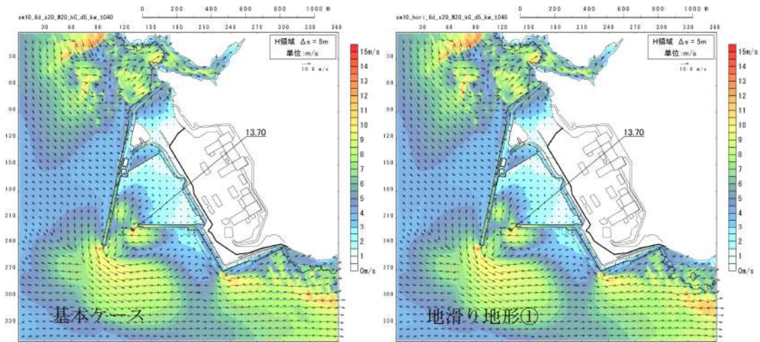
図 2.1.b.c-1 (55) 地滑り地形①の斜面崩壊の有無による最大流速分布の比較 (基準津波 (波源 I, 防波堤損傷なし))
