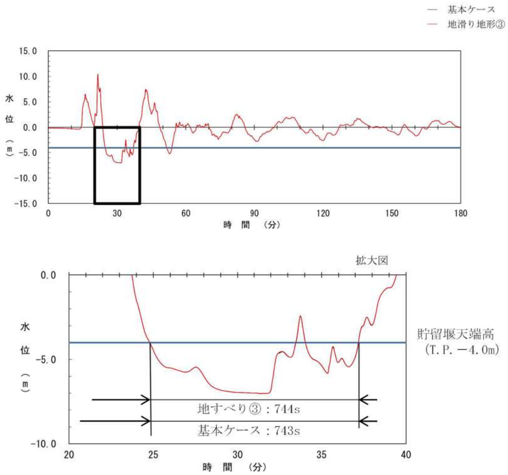
図 2. 1. b. c-2 (37) 地滑り地形③の斜面崩壊の有無による貯留堰を下回る時間の比較 (基準津波 (波源K, 南防波堤損傷))
