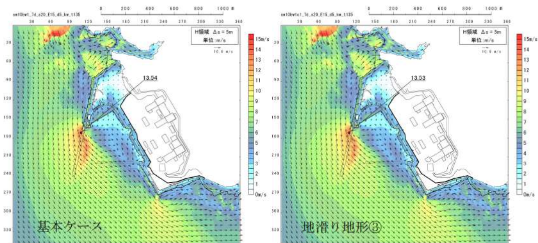
図 2. 1. b. c-2 (60) 地滑り地形③の斜面崩壊の有無による最大流速分布の比較 (最大流速波源 (波源K, 北及び南防波堤損傷))
