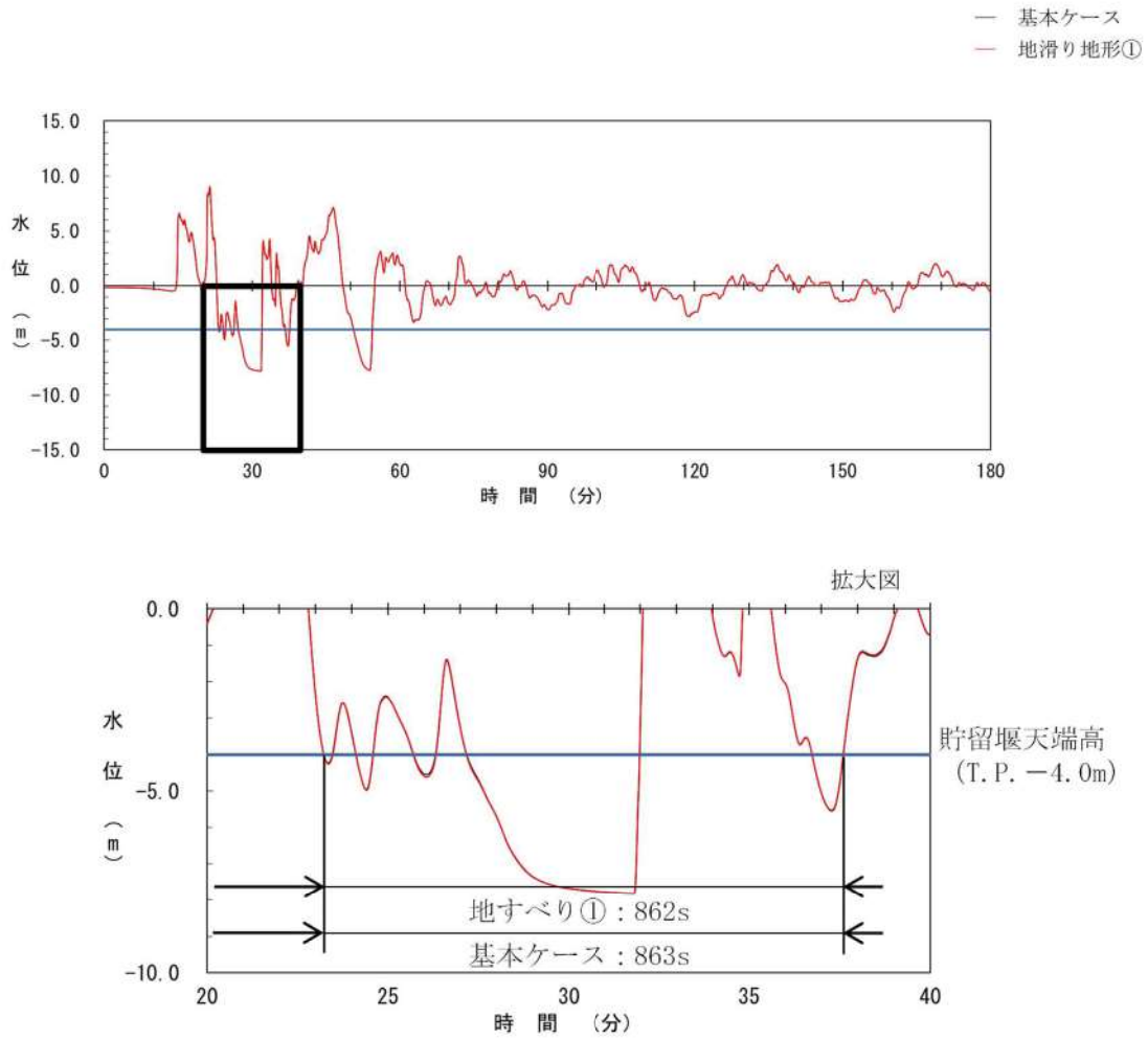
図 2. 1. b. c-1 (40) 地滑り地形①の斜面崩壊の有無による貯留堰を下回る時間の比較 (基準津波 (波源 L, 北防波堤損傷))
