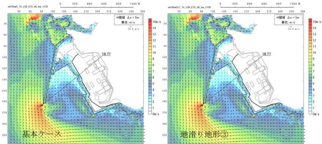
図 2. 1. b. c-2 (47) 地滑り地形③の斜面崩壊の有無による最大流速分布の比較 (基準津波 (波源D, 南防波堤損傷))
