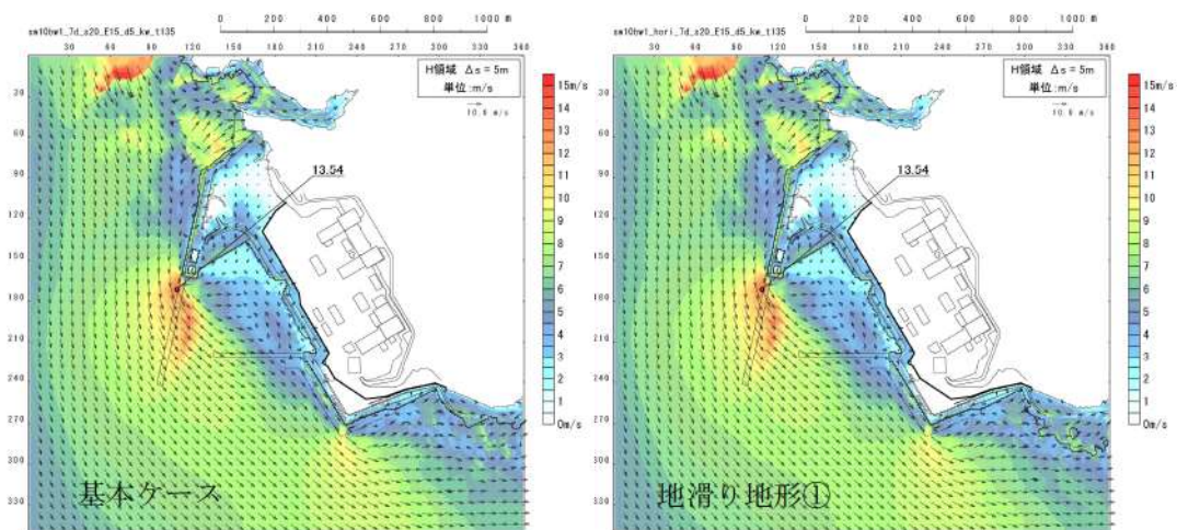
図 2.1.b.c-1 (60) 地滑り地形①の斜面崩壊の有無による最大流速分布の比較 (最大流速波源 (波源K, 北及び南防波堤損傷))
