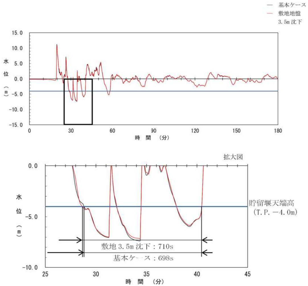
図 2.1.c.b-22 (34) 敷地（陸域）の地盤変状（3.5m 沈下）の有無による貯留堰を下回る時間の比較（基準津波（波源 J，北及び南防波堤損傷））
