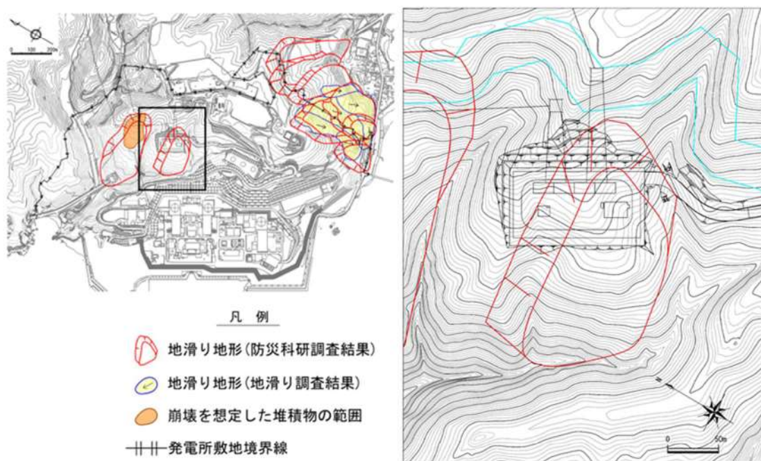
図 2.1. b. a-4 地滑り地形②分布図
