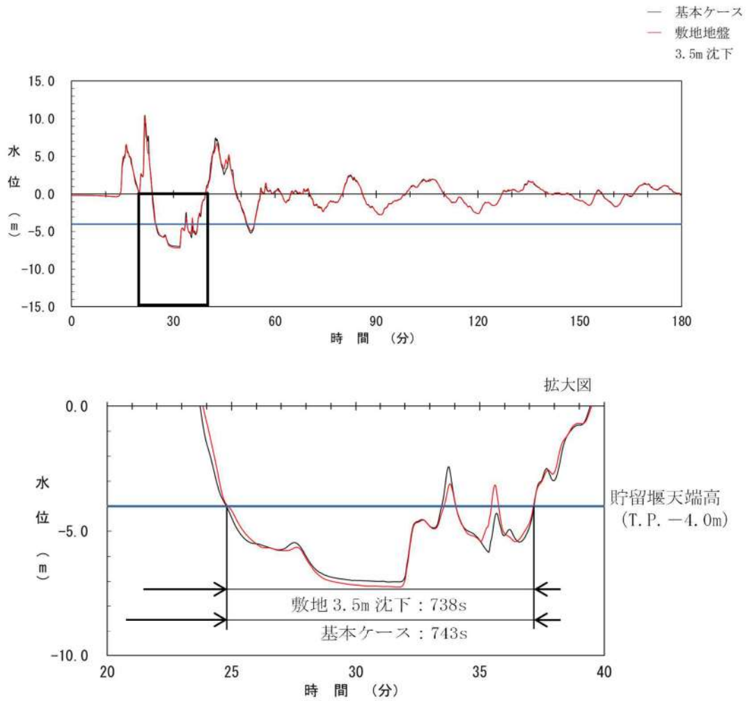
図 2.1.c.b-22 (37) 敷地（陸域）の地盤変状（3.5m 沈下）の有無による貯留堰を下回る時間の比較（基準津波（波源K，南防波堤損傷））
