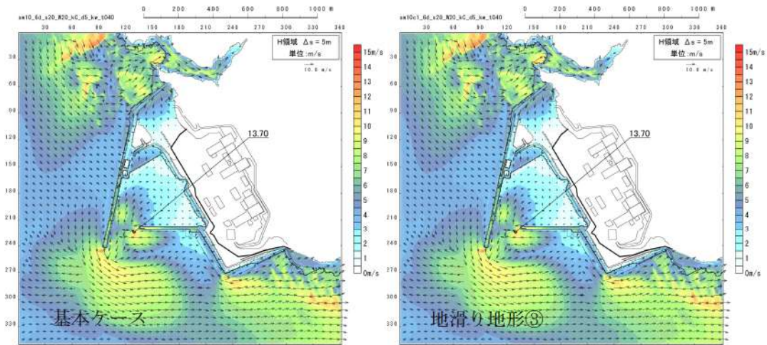
図 2. 1. b. c-2 (55) 地滑り地形③の斜面崩壊の有無による最大流速分布の比較 (基準津波 (波源 I, 防波堤損傷なし))
