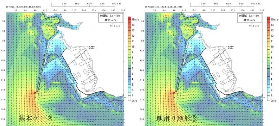
図 2. 1. b. c-2 (53) 地滑り地形③の斜面崩壊の有無による最大流速分布の比較 (基準津波 (波源G, 南防波堤損傷))
