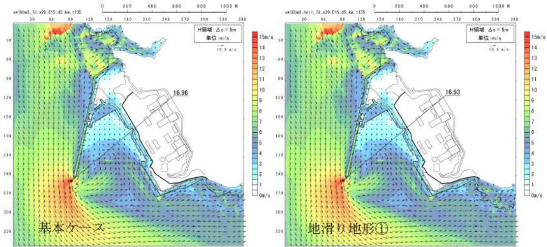
図 2. 1. b. c-1 (57) 地滑り地形①の斜面崩壊の有無による最大流速分布の比較 (基準津波 (波源K, 南防波堤損傷))
