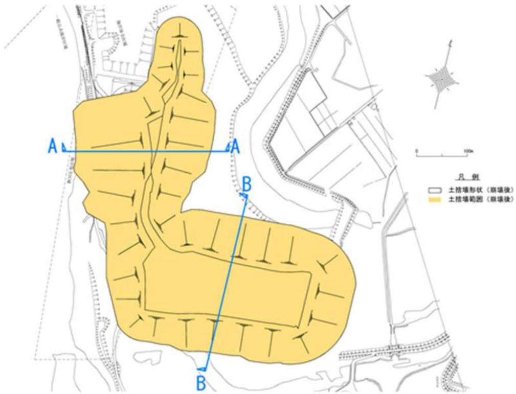
図 2.1. e. c-2 (1) 斜面崩壊を考慮した土捨場形状
