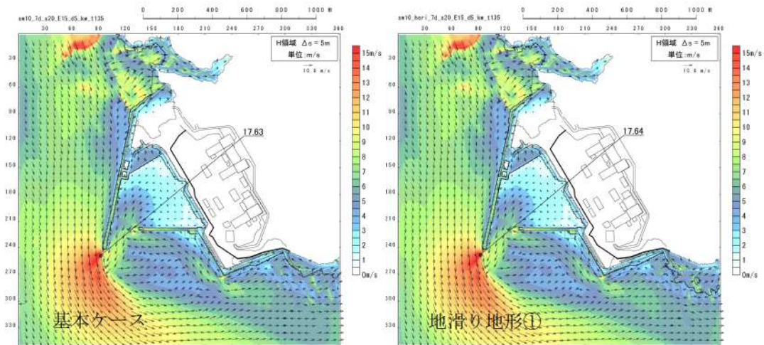
図 2.1.b.c-1 (59) 地滑り地形①の斜面崩壊の有無による最大流速分布の比較 (最大流速波源 (波源K, 防波堤損傷なし))
