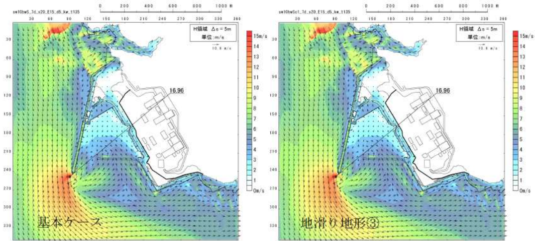
図 2. 1. b. c-2 (57) 地滑り地形③の斜面崩壊の有無による最大流速分布の比較 (基準津波 (波源 K, 南防波堤損傷))
