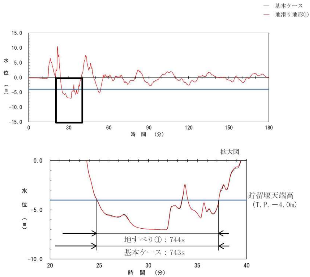
図 2. 1. b. c-1 (37) 地滑り地形①の斜面崩壊の有無による貯留堰を下回る時間の比較 (基準津波 (波源K, 南防波堤損傷))
