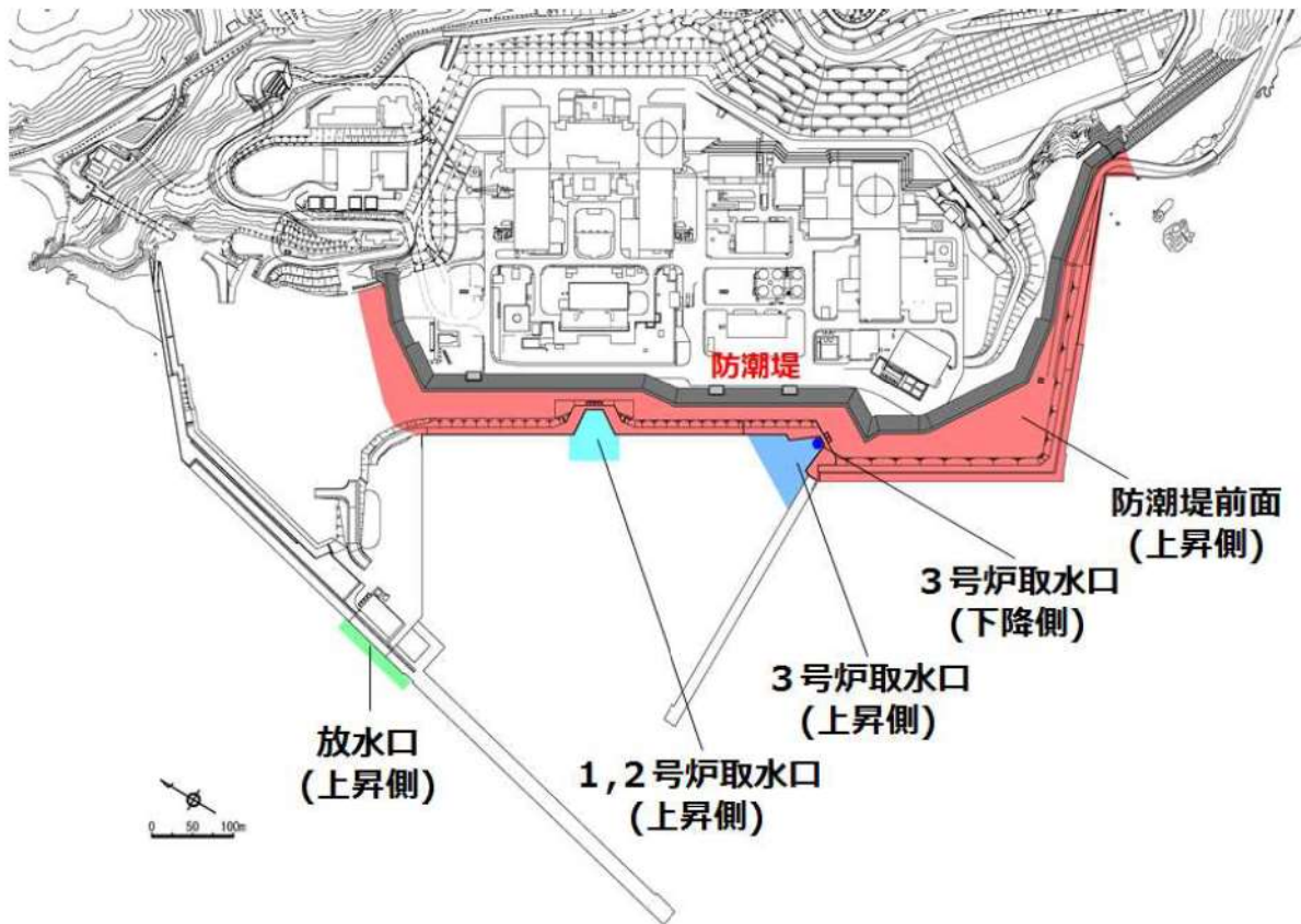
第 1.4-1 図 津波水位の評価地点
