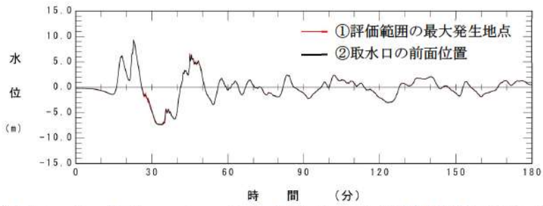
参考図 3-6 (5) 1, 2号炉取水口水位時刻歴波形の比較 (基準津波 (波源C, 防波堤損傷なし))
