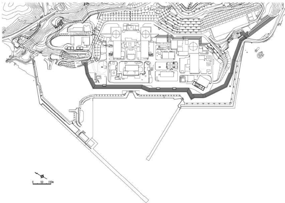
図 1.1.a.c-4 敷地平面図
