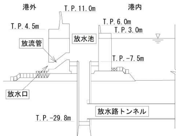
参考図 3-12 放水池断面図
