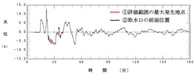
参考図 3-6 (4) 3号炉取水口水位時刻歴波形の比較 (基準津波 (波源 B, 北防波堤損傷なし))
