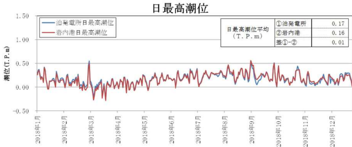
第1.5-5図 泊発電所と岩内港の日最高潮位の比較
