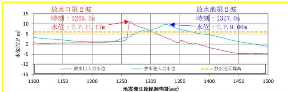
参考図 3-14 (2) 放水口・放水池の水位時刻歴波形の比較 (拡大) (基準津波 (波源D, 防波堤損傷なし))
