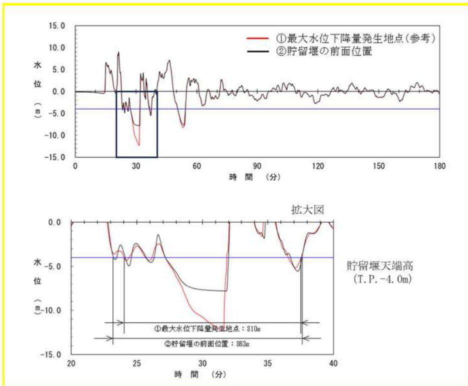
参考図 3-11 (4) 3号炉取水口水位時刻歴波形の比較 (基準津波 (波源L, 北防波堤損傷))
