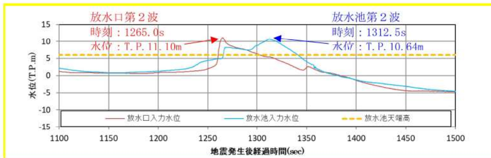
参考図 3-14 (4) 放水口・放水池の水位時刻歴波形の比較 (拡大) (基準津波 (波源D, 北及び南防波堤損傷))
