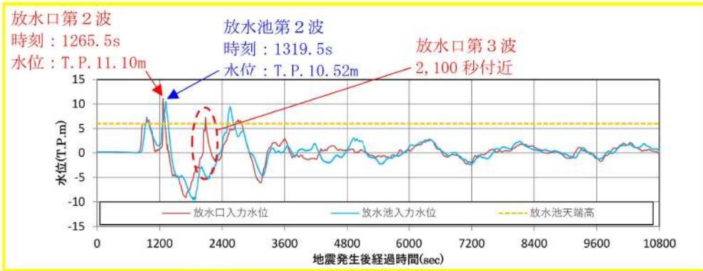
参考図 3-14 (5) 放水口・放水池の水位時刻歴波形の比較 (基準津波 (波源D, 南防波堤損傷))
