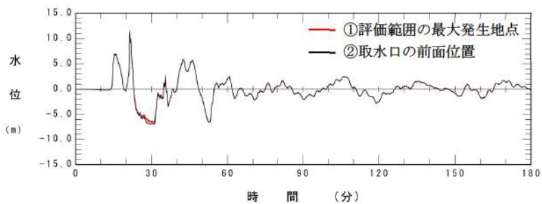
参考図 3-6 (8) 1, 2号炉取水口水位時刻歴波形の比較 (基準津波 (波源H, 北防波堤損傷なし))
