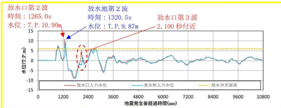
参考図 3-14 (7) 放水口・放水池の水位時刻歴波形の比較 (基準津波 (波源D, 北防波堤損傷))
