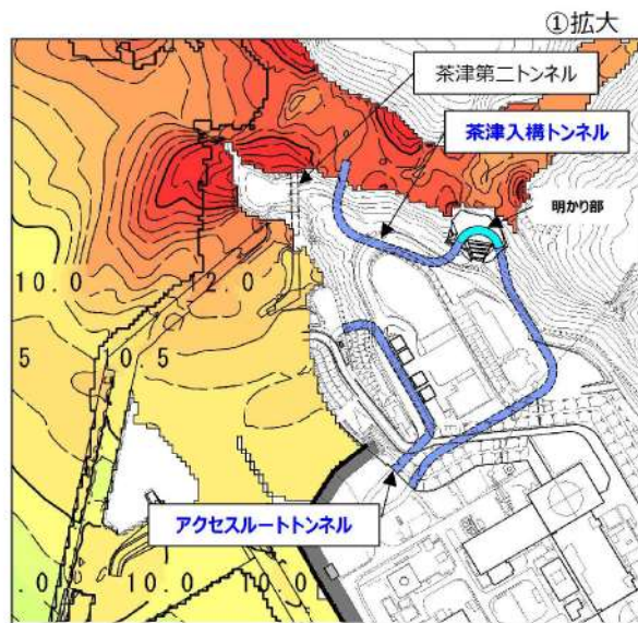
図 1.2. c-1 (2) 最大水位上昇量分布図 (基準津波 (波源 J, 北及び南防波堤損傷) ※) ※現時点における最大ケース
