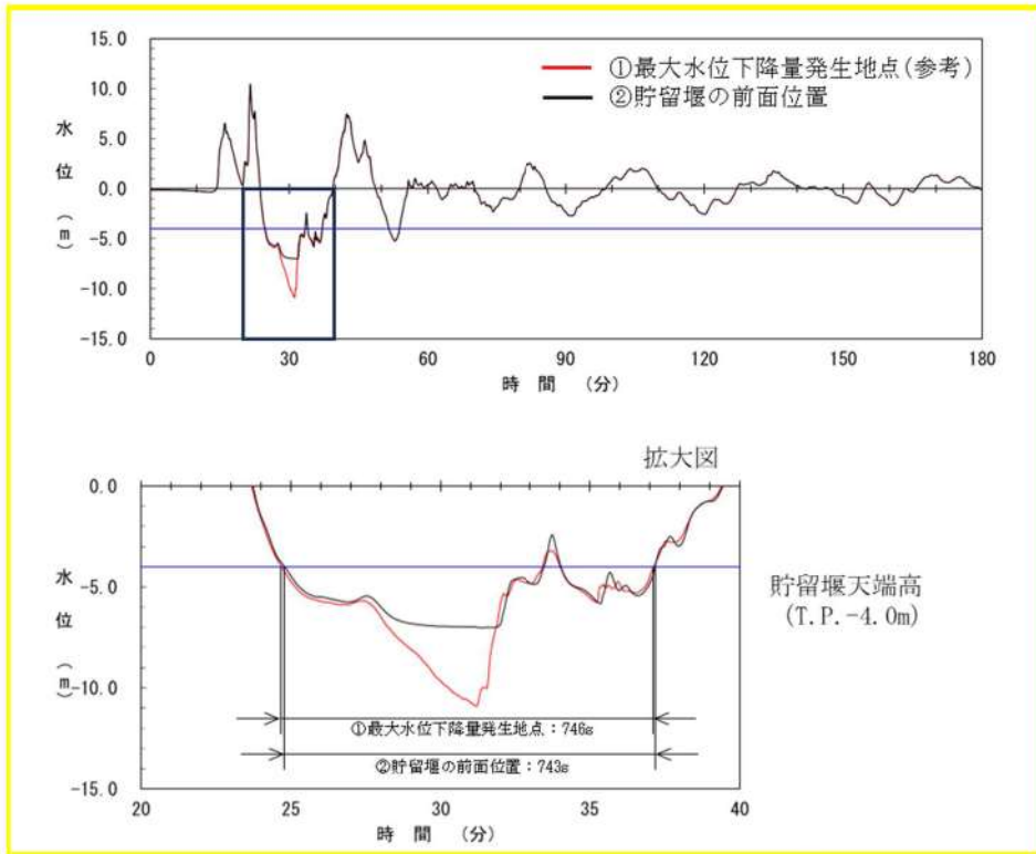
参考図 3-11 (3) 3号炉取水口水位時刻歴波形の比較 (基準津波 (波源K, 南防波堤損傷))
