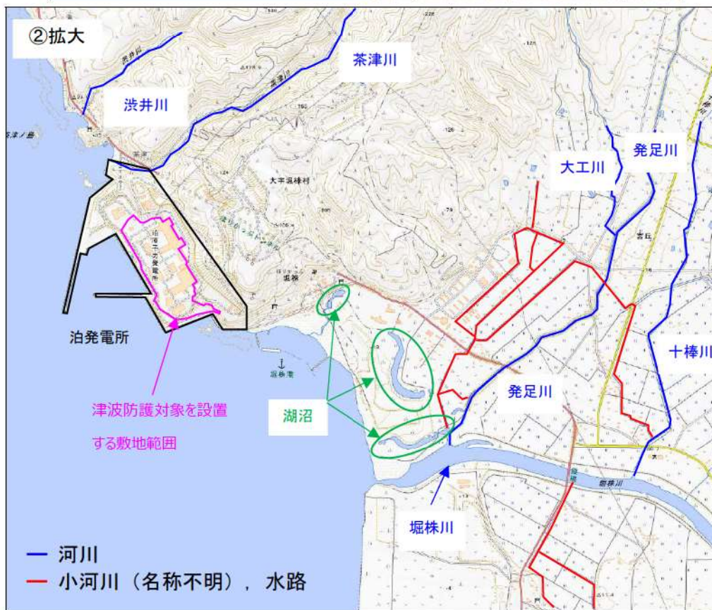
図 1.1.c.a-1 (2) 敷地周辺の河川・水路抽出範囲※
