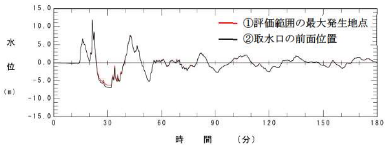
参考図 3-6 (3) 3号炉取水口水位時刻歴波形の比較 (基準津波 (波源 E, 南防波堤損傷))
