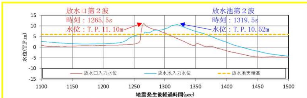
参考図 3-14 (6) 放水口・放水池の水位時刻歴波形の比較 (拡大) (基準津波 (波源D, 南防波堤損傷))
