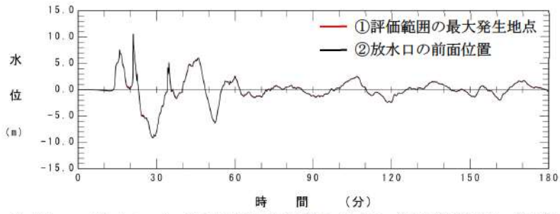
参考図 3-8 (4) 放水口水位時刻歴波形の比較 (基準津波 (波源D, 北防波堤損傷なし))
