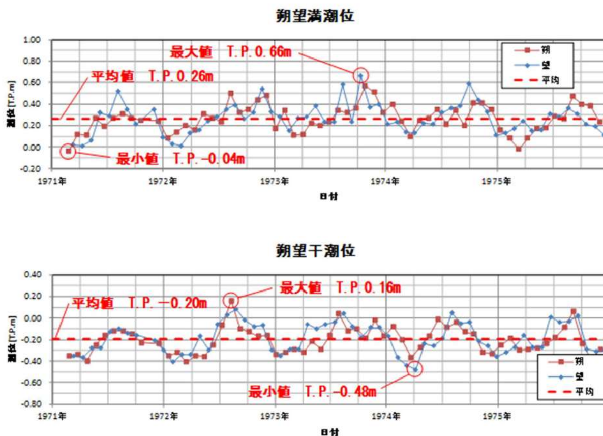
第 1.5-4 図 各月の朔望満干潮位 (1971 年 3 月～1975 年 12 月)
