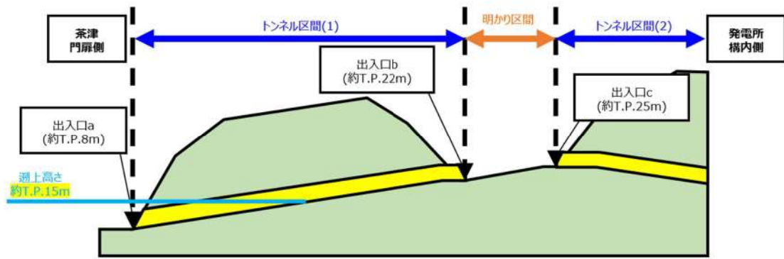
図 1.2. c-1 (3) 茶津入構トンネル断面図
