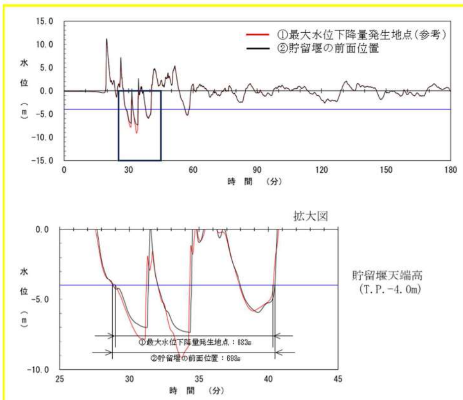
参考図 3-11 (2) 3号炉取水口水位時刻歴波形の比較 (基準津波 (波源 J, 北及び南防波堤損傷))
