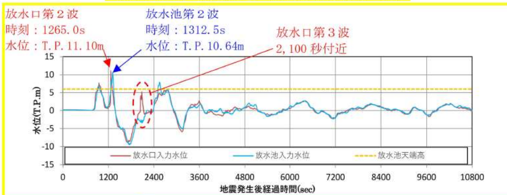
参考図 3-14 (3) 放水口・放水池の水位時刻歴波形の比較 (基準津波 (波源D, 北及び南防波堤損傷))
