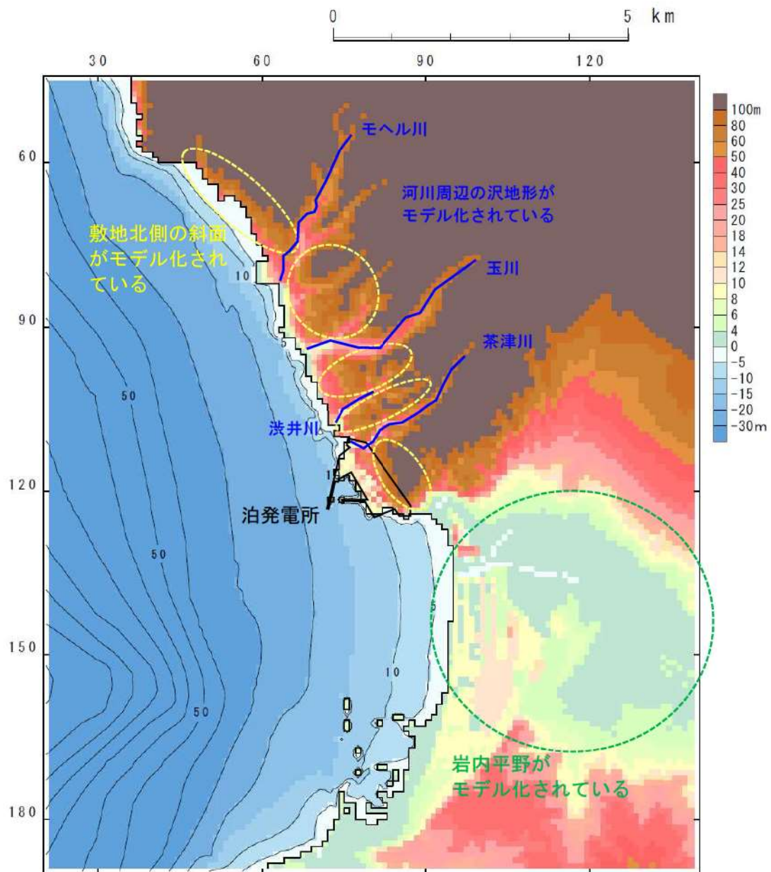
図 1.1. a. c-5 地形モデル (93m 計算格子領域)
