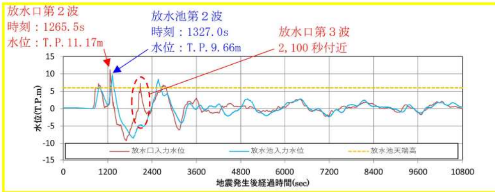
参考図 3-14 (1) 放水口・放水池の水位時刻歴波形の比較 (基準津波 (波源D, 防波堤損傷なし))
