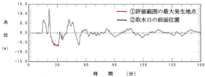
参考図 3-6 (6) 1, 2号炉取水口水位時刻歴波形の比較 (基準津波 (波源E, 北及び南防波堤損傷))
