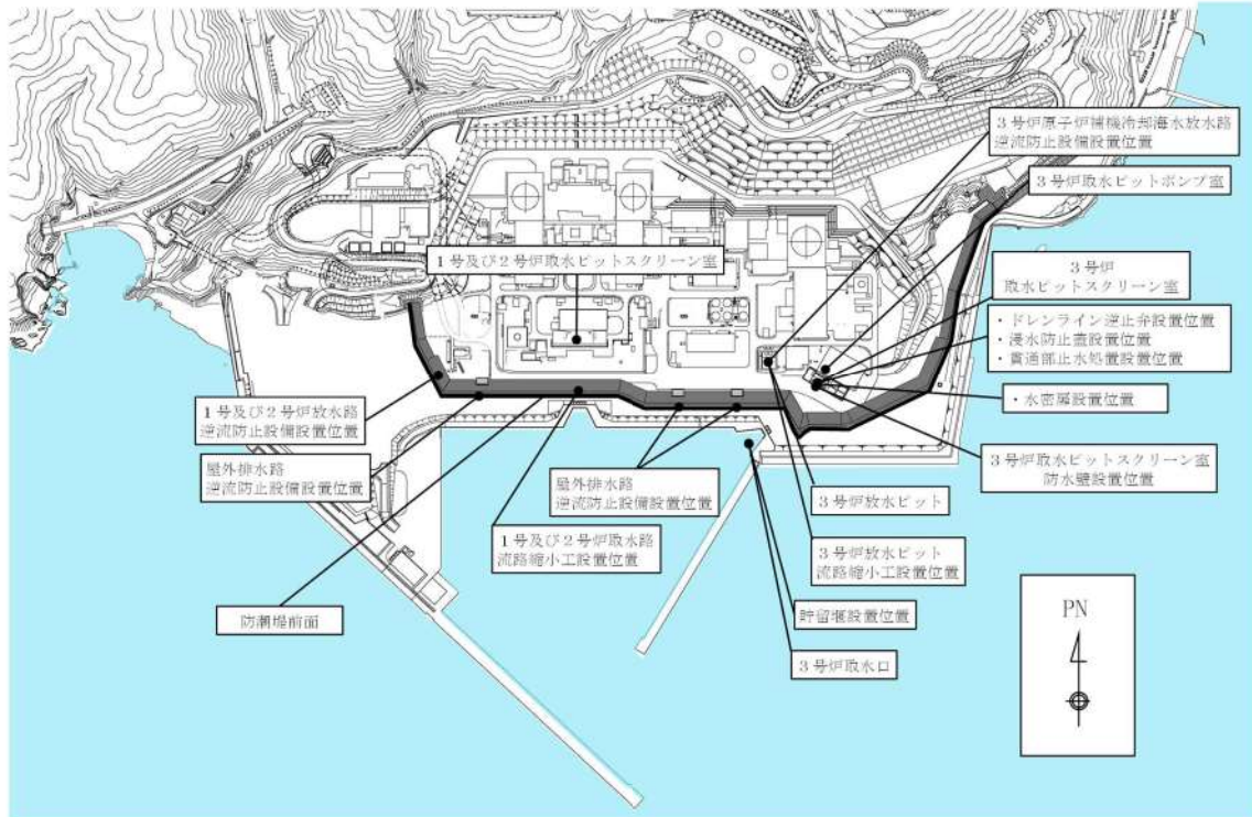
第 1. 4-2 図 入力津波設定位置
