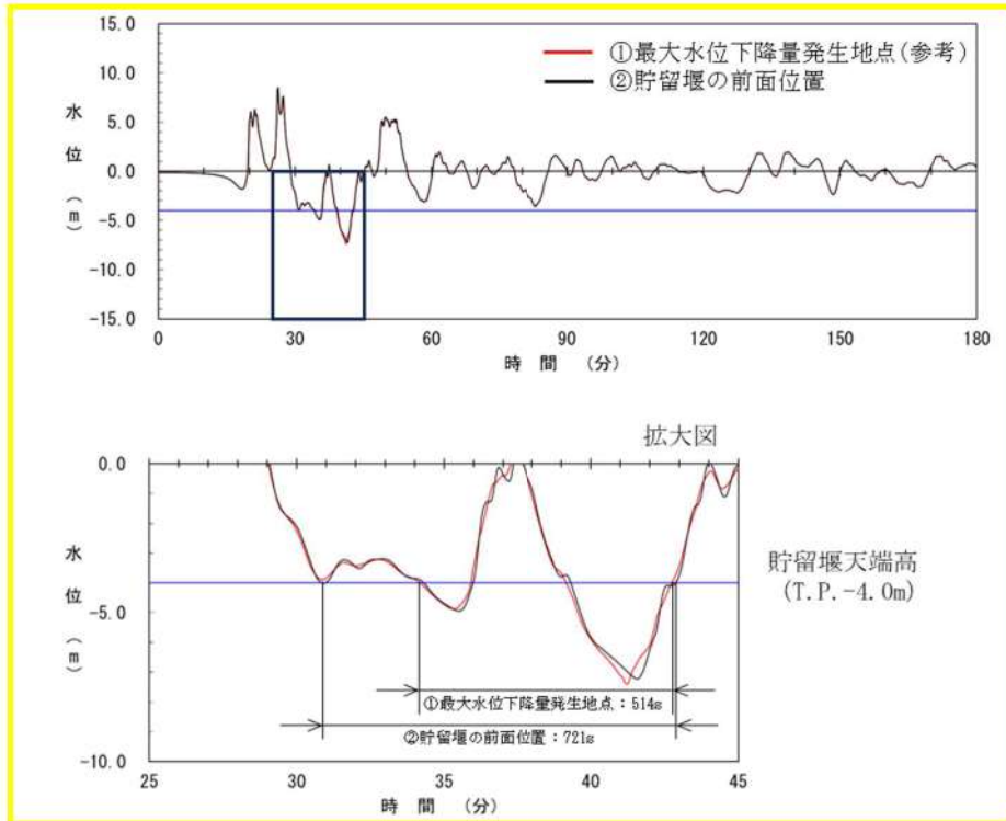
参考図 3-11 (1) 3号炉取水口水位時刻歴波形の比較 (基準津波 (波源 I, 防波堤損傷なし))
