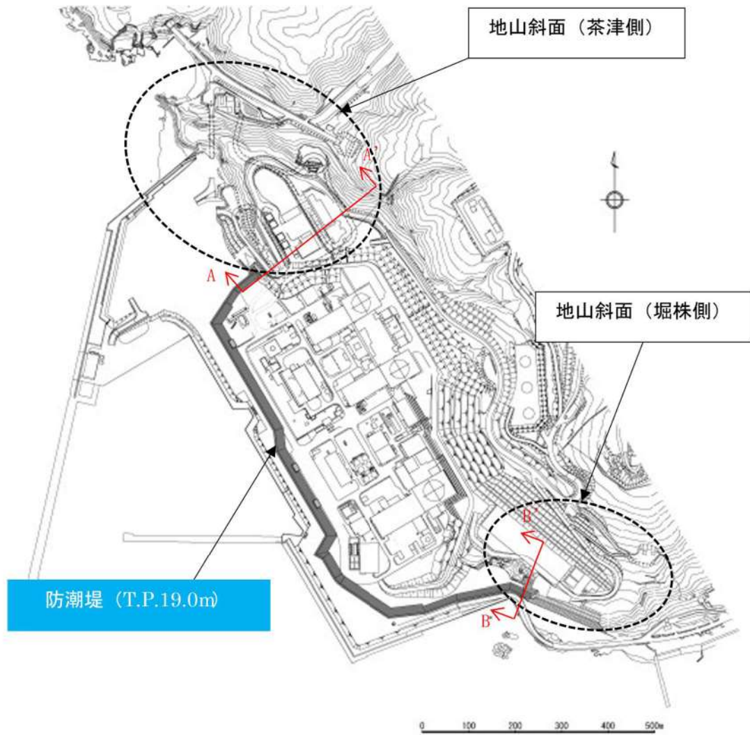
图 2.1. a. b-1 地山位置图
