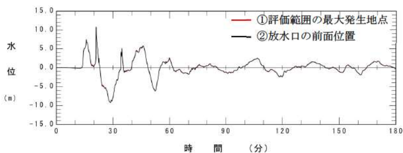
参考図 3-8 (2) 放水口水位時刻歴波形の比較（基準津波（波源D，北及び南防波堤損傷））
