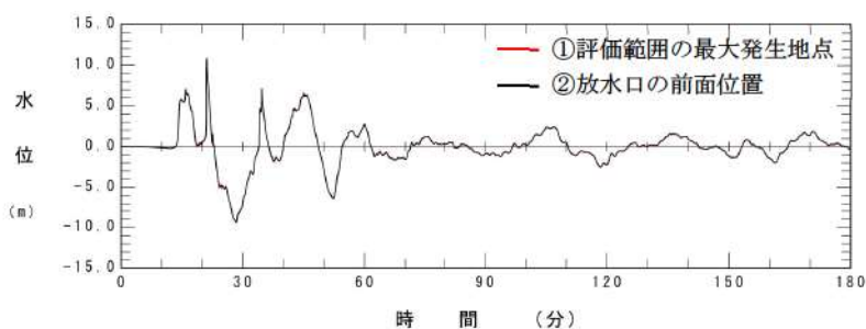
参考図 3-8 (3) 放水口水位時刻歴波形の比較（基準津波（波源D，南防波堤損傷なし））
