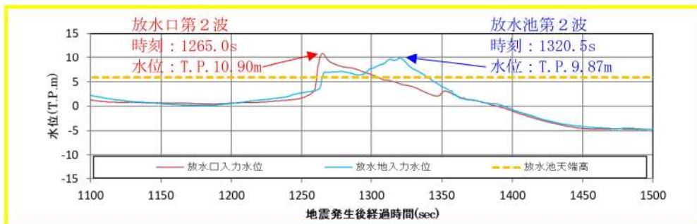
参考図 3-14 (8) 放水口・放水池の水位時刻歴波形の比較 (拡大) (基準津波 (波源D, 北防波堤損傷))
