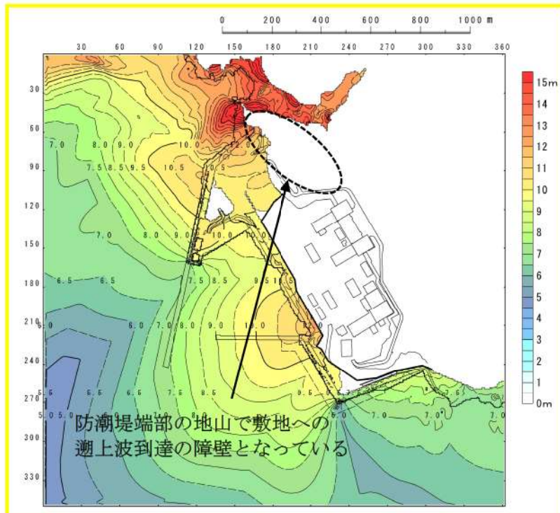
図 2.1.a.b-2 (2) 最大水位上昇量分布図 (基準津波：波源J，北及び南防波堤損傷)
