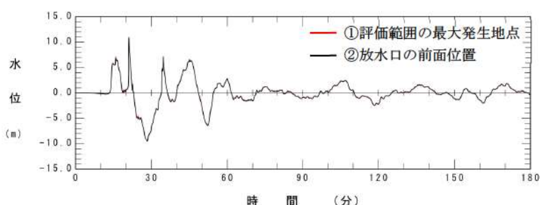
参考図 3-8 (1) 放水口水位時刻歴波形の比較（基準津波（波源D，防波堤損傷なし））
