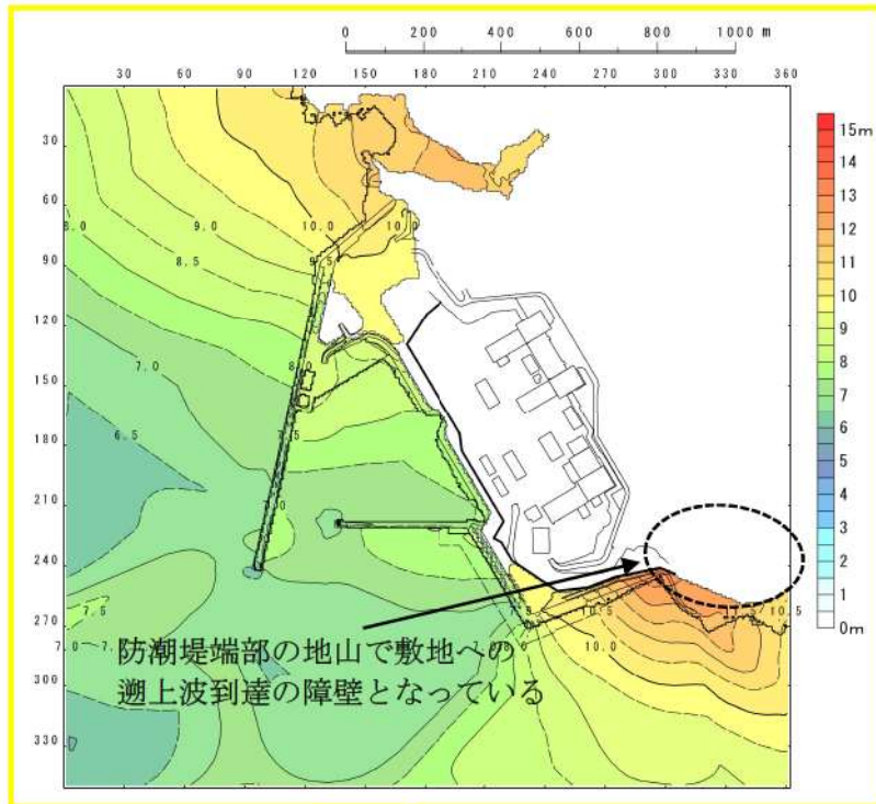
図 2.1.a.b-2 (1) 最大水位上昇量分布図 (基準津波：波源A，防波堤損傷なし)
