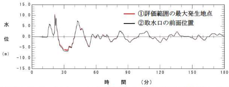
参考図 3-6 (1) 3号炉取水口水位時刻歴波形の比較 (基準津波 (波源 B, 防波堤損傷なし))
