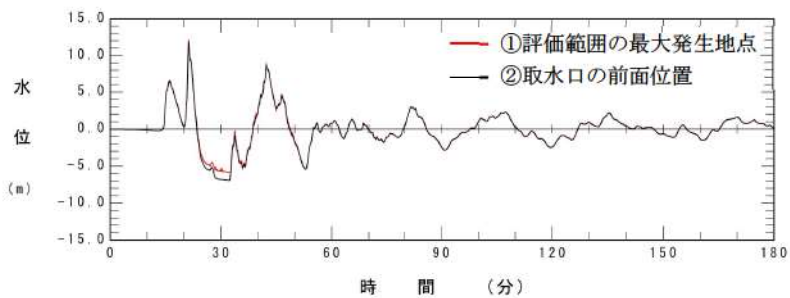
参考図 3-6 (7) 1, 2号炉取水口水位時刻歴波形の比較 (基準津波 (波源G, 南防波堤損傷))
