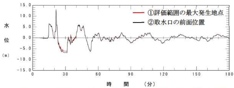
参考図 3-6 (2) 3号炉取水口水位時刻歴波形の比較 (基準津波 (波源 F, 北及び南防波堤損傷))
