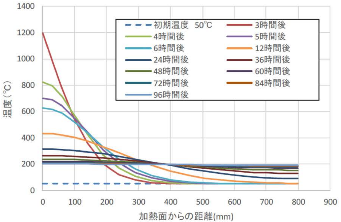
第 3.1.4.4-13 図 評価対象外壁における温度分布 (燃焼継続 3 時間)
