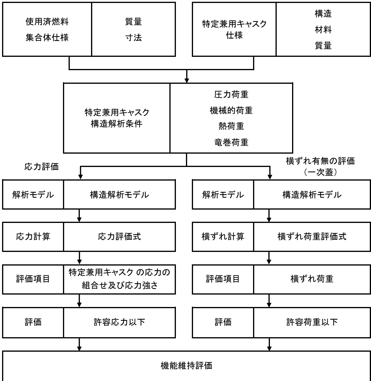
図 1 竜巻荷重作用時の機能維持評価フロー
