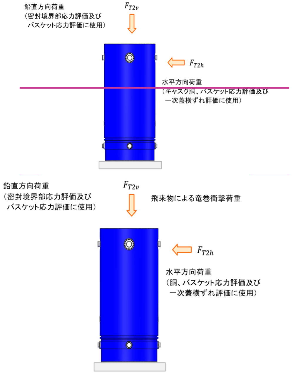
図 A-1 竜巻荷重の作用方向
