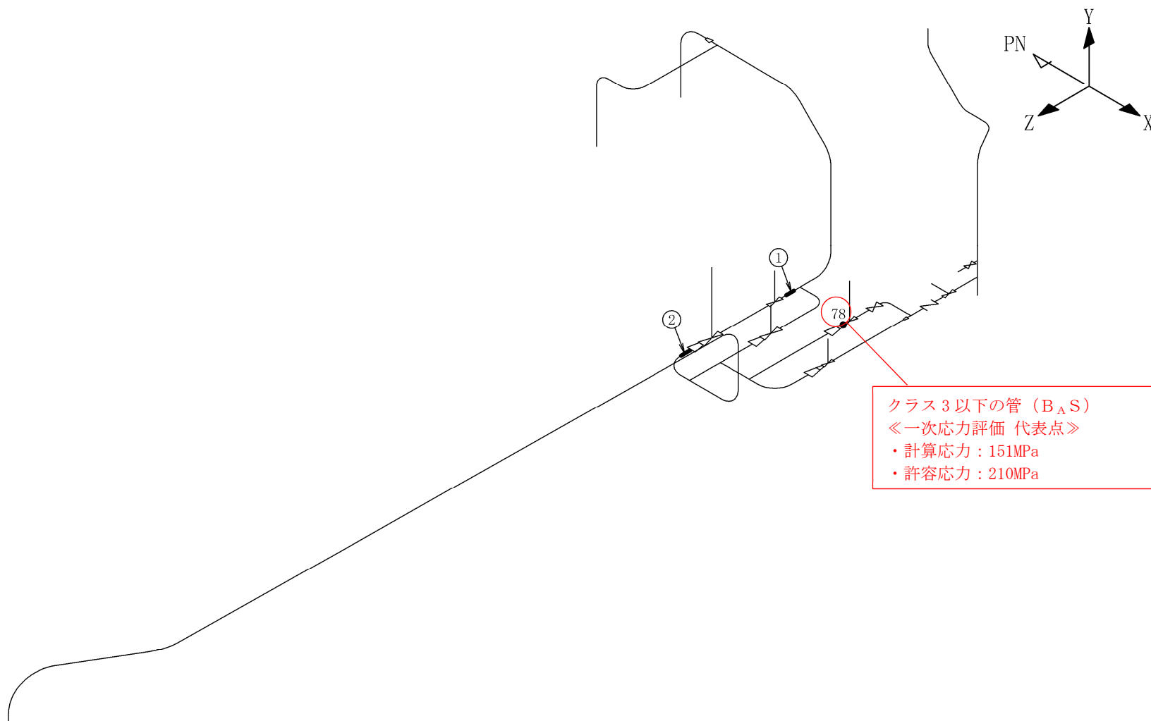
図 3-6-2 TGS-T-3 解析モデル図
